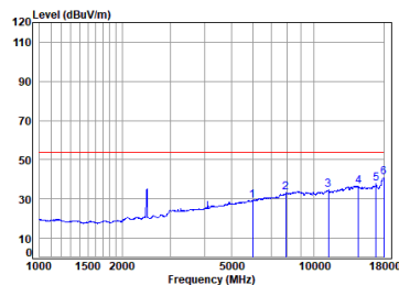
11n_20M_TX_CH_11_Vertical-Avg
