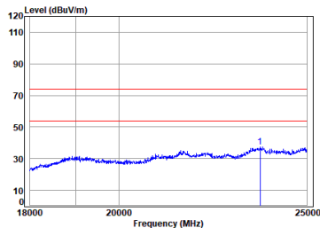
11b_TX_CH_06_Vertical
