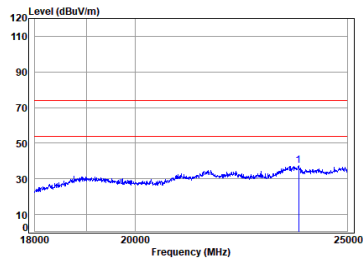
11g_TX_CH_01_Horizontal
