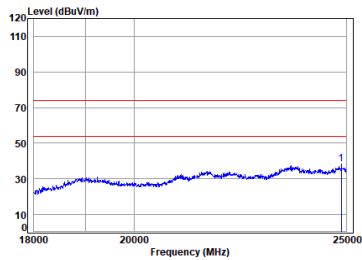
11n_20M_TX_CH_06_Horizontal
