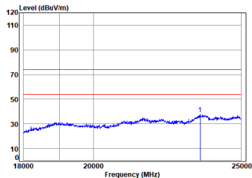
11g_TX_CH_11_Horizontal
