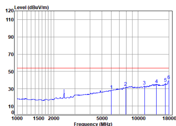
11n_20M_TX_CH_06_Horizontal-Avg
