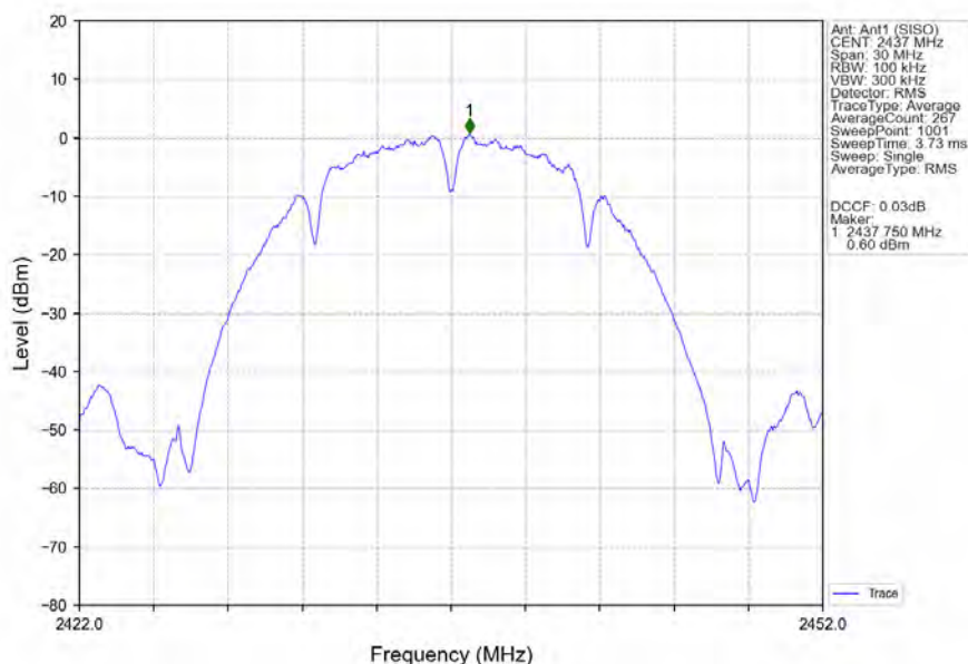
802.11b_MCH_2437MHz_Ant1 (SISO)_NTNV
