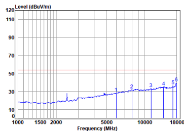
11n_20M_TX_CH_06_Vertical-Avg
