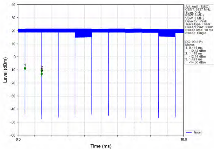
802.11b_MCH_2437MHz_Ant1 (SISO)_NTNV
