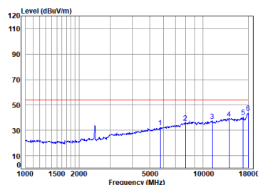
11n_20M_TX_CH_11_Horizontal-Avg
