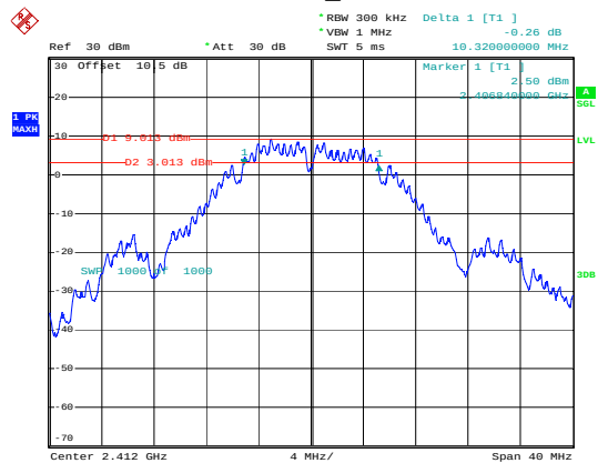
802.11b_2412MHz
