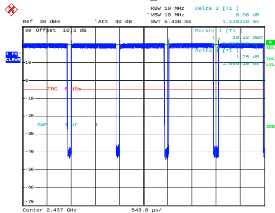
802.11b_2437MHz
