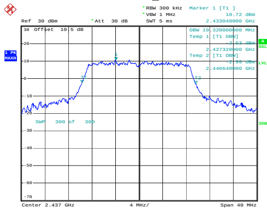
802.11n20_2437MHz
