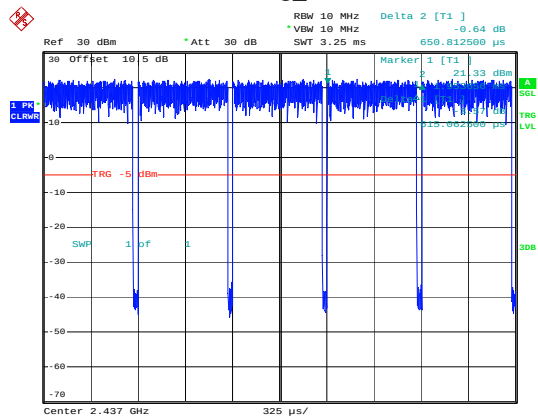
802.11g_2437MHz
