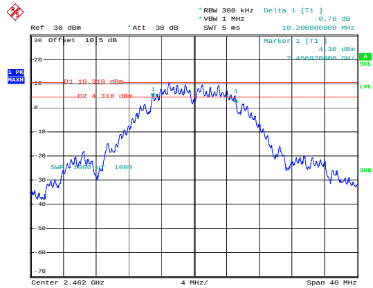
802.11b_2462MHz
