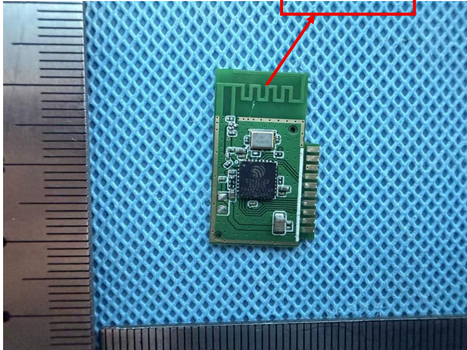
2.4 GHz Antenna
