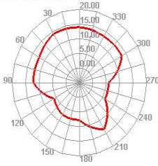
Wifi 13 TRP E2
