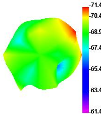
Wifi 7 TIS E1
