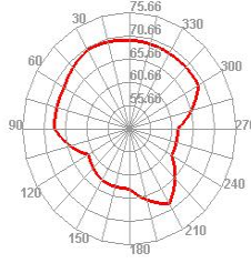
Wifi 13 TIS E2
