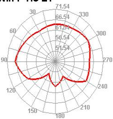
Wifi 7 TIS E1
