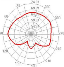
Wifi 7 TIS E1
