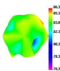
Wifi 13 TIS E1
