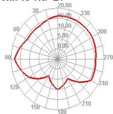
Wifi 13 TRP E1
