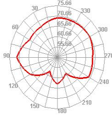
Wifi 13 TIS E1
