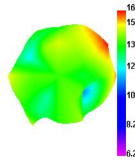
Wifi 7 TRP E1
