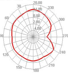
Wifi 7 TRP E2
