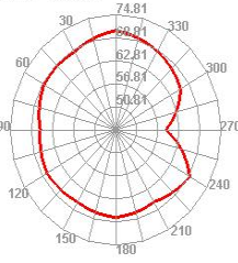
Wifi 7 TIS E2
