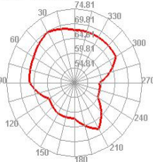
Wifi 7 TIS E2
