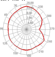
Wifi 7 TRP E2
