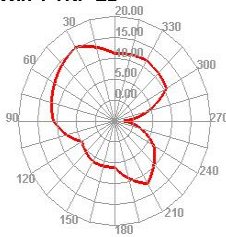
Wifi 1 TRP E2
