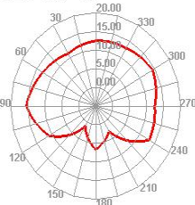
Wifi 7 TRP E1
