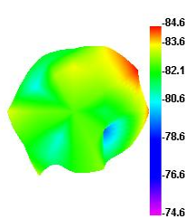
Wifi 7 TIS E1
