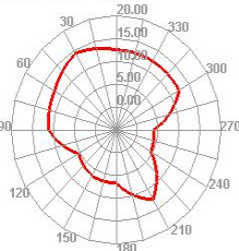
Wifi 7 TRP E2
