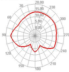
Wifi 13 TRP E1
