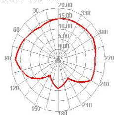
Wifi 7 TRP E1
