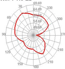
Wifi 1 TIS E2
