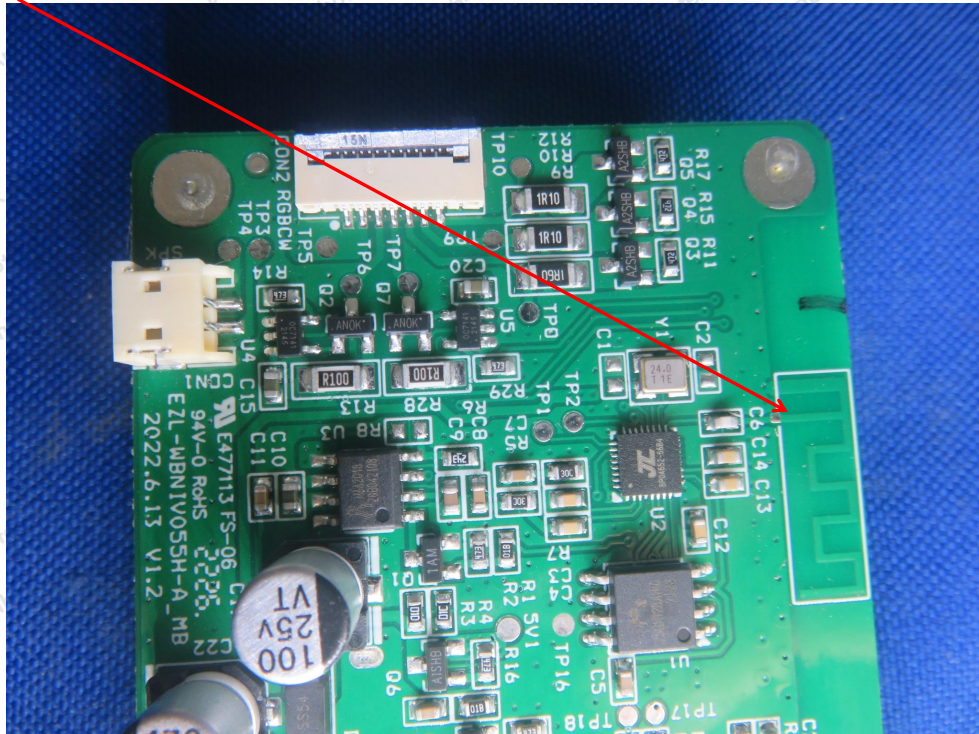
BT ANT
