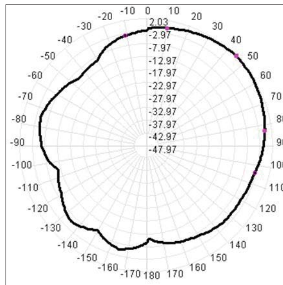
2440MHz
