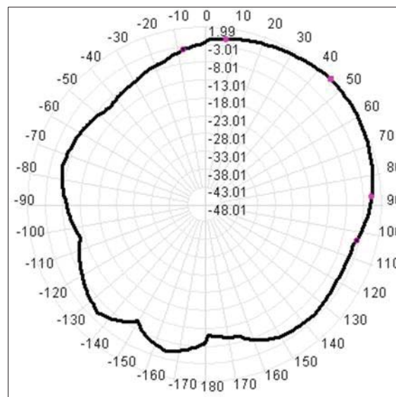
2480MHz
