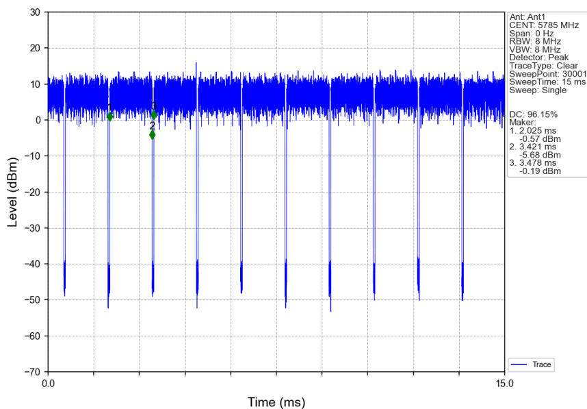
802.11a_MCH_5785MHz_Ant1_NTNV
