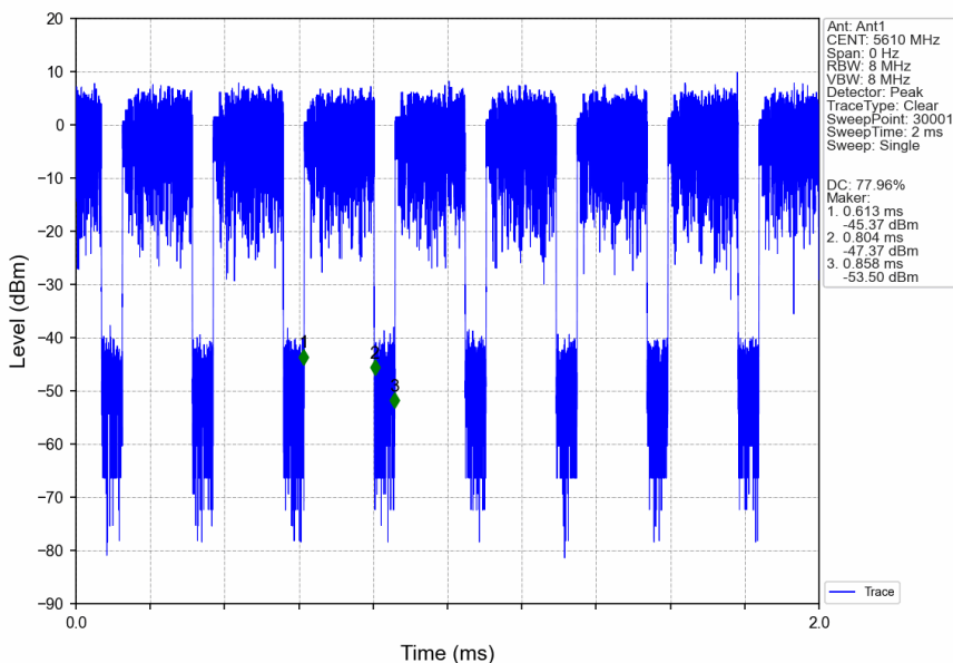
802.11ac(VHT80)_HCH_5610MHz_Ant1_NTNV
