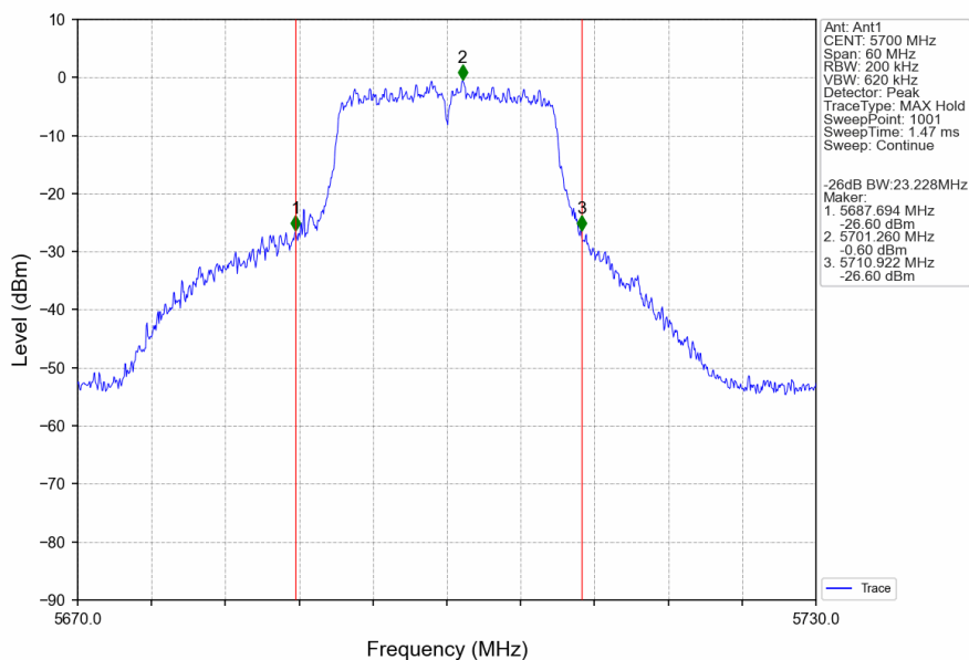
802.11ac(VHT20)_HCH_5700MHz_Ant1_NTNV
