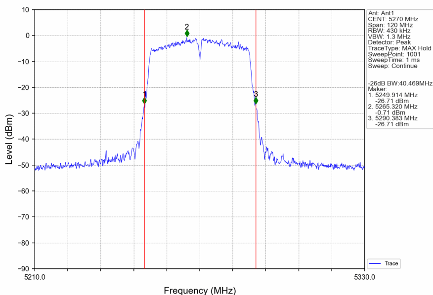
802.11ac(VHT40)_LCH_5270MHz_Ant1_NTNV
