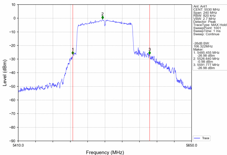
802.11ac(VHT80)_LCH_5530MHz_Ant1_NTNV
