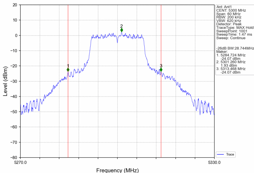
802.11a_MCH_5300MHz_Ant1_NTNV
