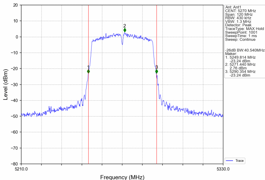
802.11n(HT40)_LCH_5270MHz_Ant1_NTNV
