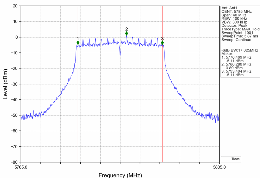
802.11n(HT20)_MCH_5785MHz_Ant1_NTNV
