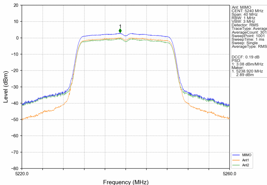
802.11n(HT20)_HCH_5240MHz_MIMO_NTNV
