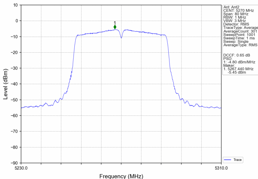
802.11ac(VHT40)_LCH_5270MHz_Ant2_NTNV
