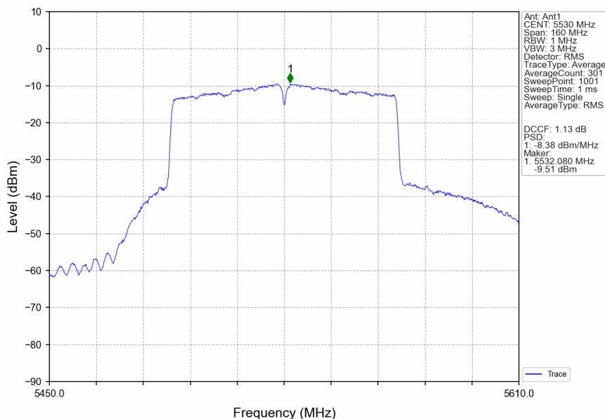
802.11ac(VHT80)_LCH_5530MHz_Ant1_NTNV
