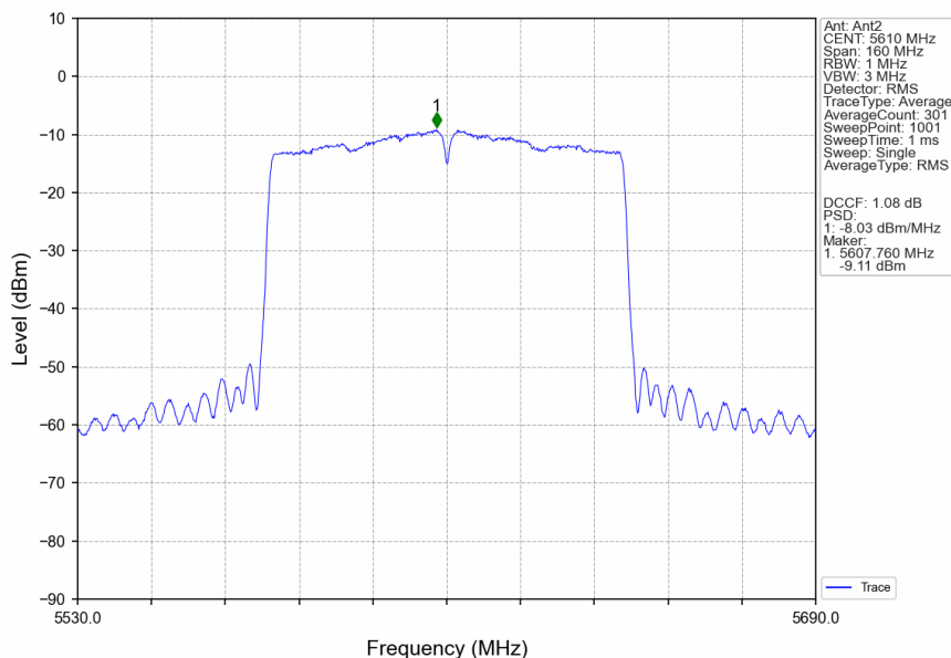
802.11ac(VHT80)_HCH_5610MHz_Ant2_NTNV
