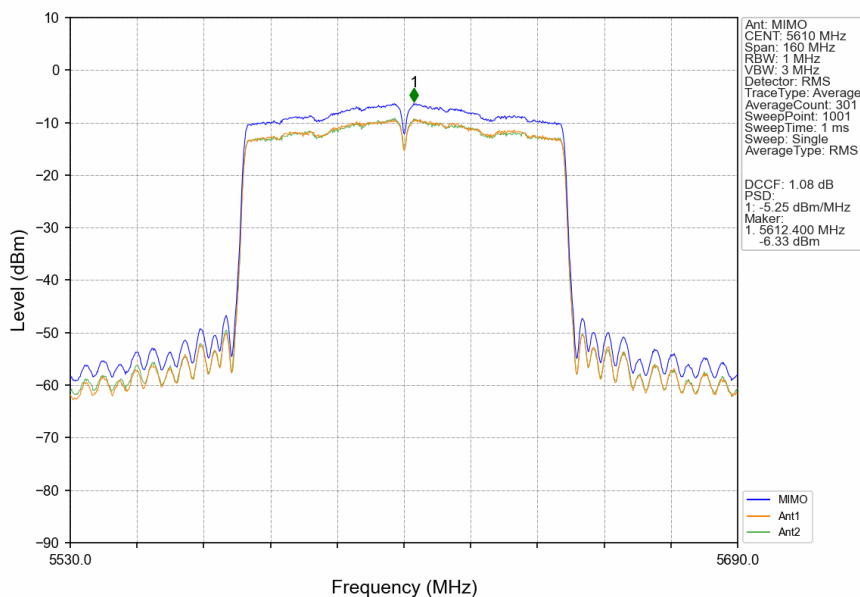
802.11ac(VHT80)_HCH_5610MHz_MIMO_NTNV
