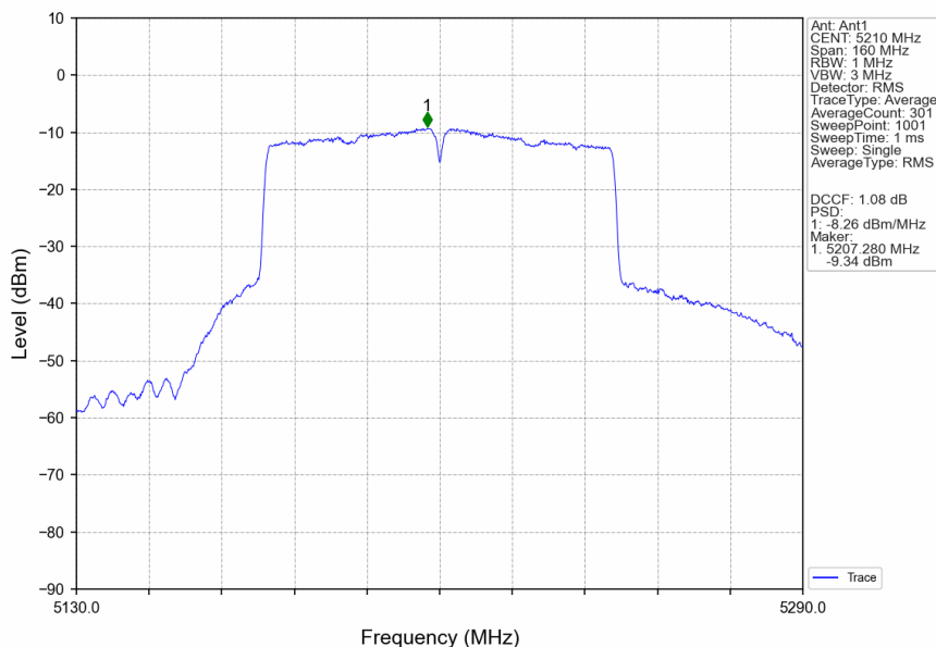
802.11ac(VHT80)_MCH_5210MHz_Ant1_NTNV
