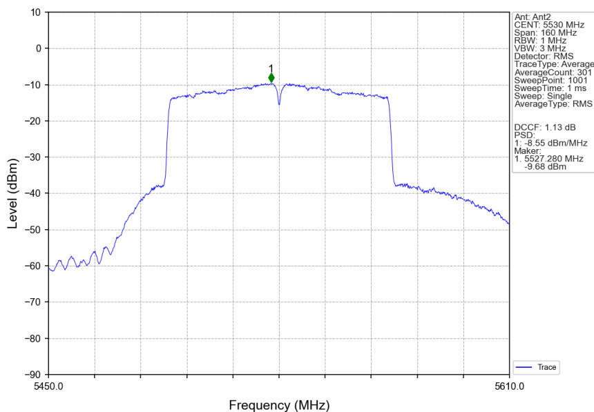
802.11ac(VHT80)_LCH_5530MHz_Ant2_NTNV
