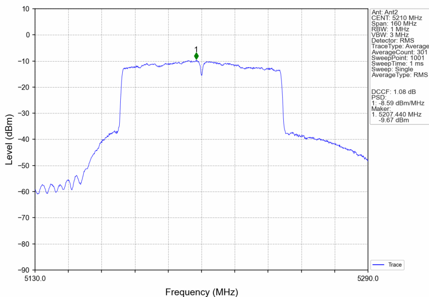
802.11ac(VHT80)_MCH_5210MHz_Ant2_NTNV
