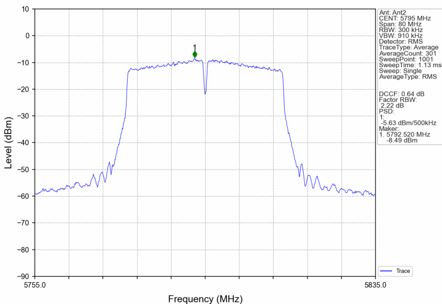
802.11n(HT40)_HCH_5795MHz_Ant2_NTNV
