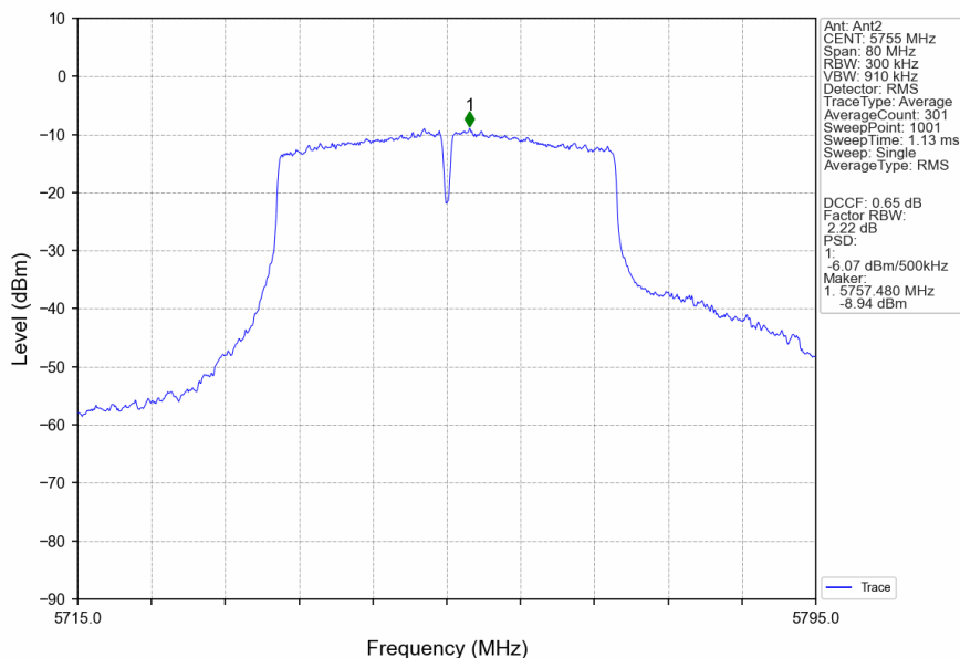
802.11n(HT40)_LCH_5755MHz_Ant2_NTNV
