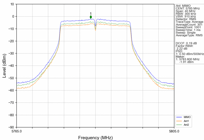
802.11n(HT20)_MCH_5785MHz_MIMO_NTNV
