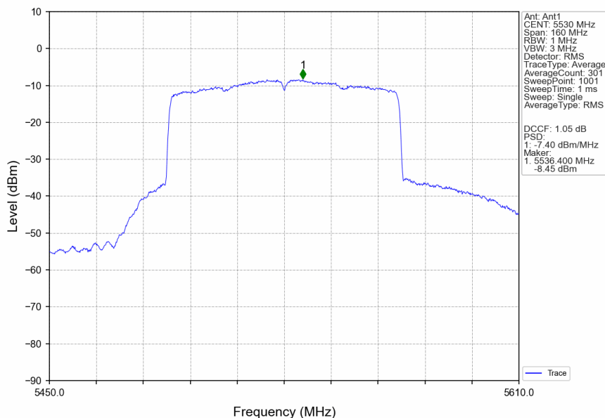
802.11ax(HEW80)_LCH_5530MHz_SU_ / _Ant1_NTNV
