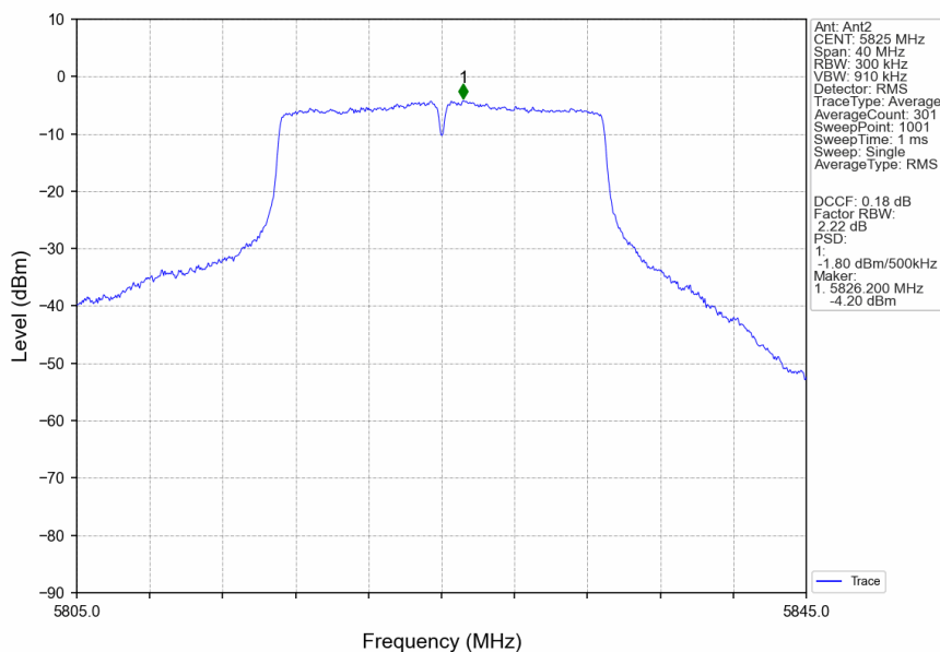
802.11n(HT20)_HCH_5825MHz_Ant2_NTNV
