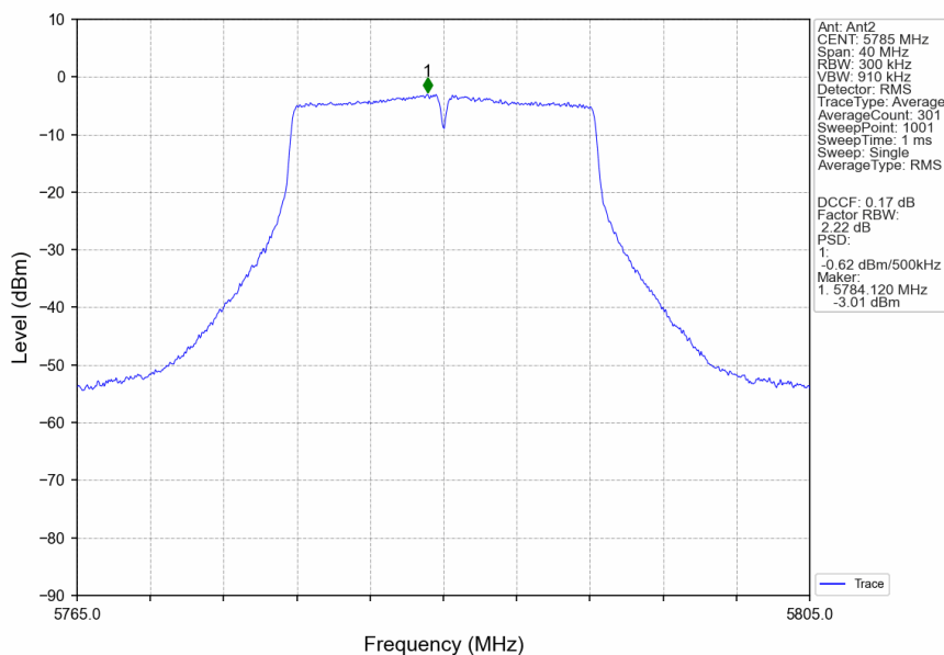
802.11a_MCH_5785MHz_Ant2_NTNV
