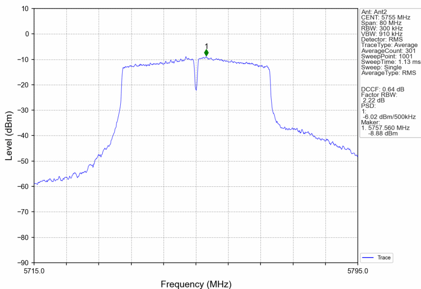
802.11ac(VHT40)_LCH_5755MHz_Ant2_NTNV
