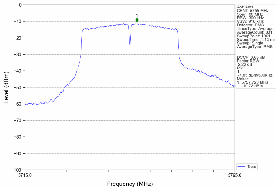
802.11n(HT40)_LCH_5755MHz_Ant1_NTNV
