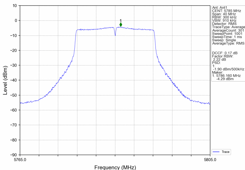
802.11a_MCH_5785MHz_Ant1_NTNV
