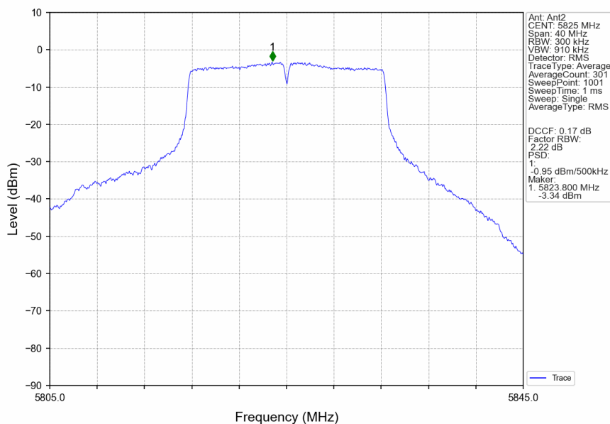
802.11a_HCH_5825MHz_Ant2_NTNV
