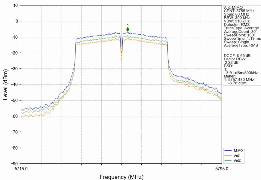
802.11n(HT40)_LCH_5755MHz_MIMO_NTNV
