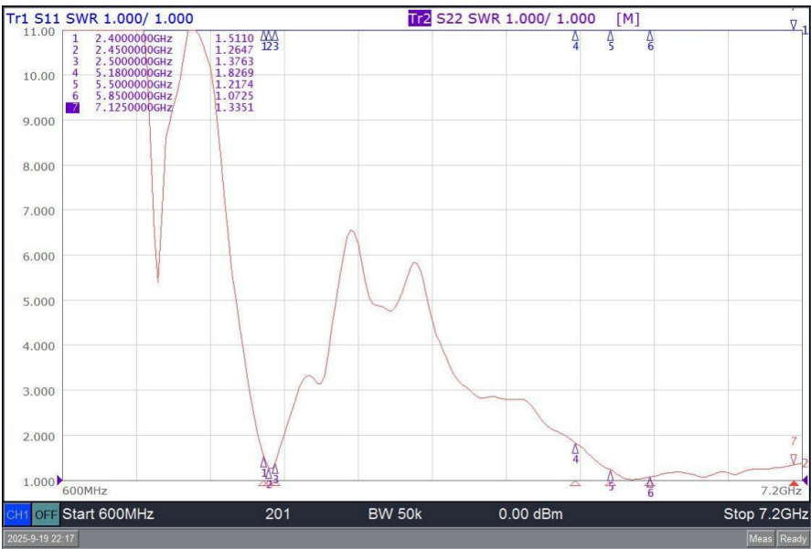
VSWR
