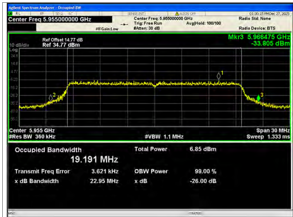
-26dB Bandwidth NVNT ax20 5955MHz Ant1 MIMO
