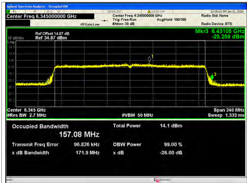
-26dB Bandwidth NVNT ax160 6345MHz Ant1 MIMO
