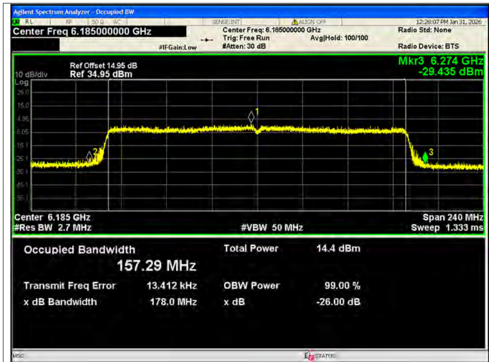
-26dB Bandwidth NVNT ax160 6185MHz Ant1 MIMO
