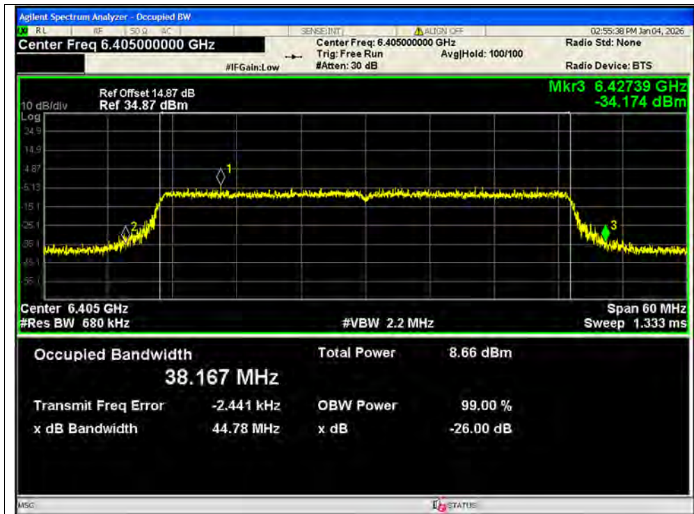
-26dB Bandwidth NVNT ax40 6405MHz Ant1 MIMO
