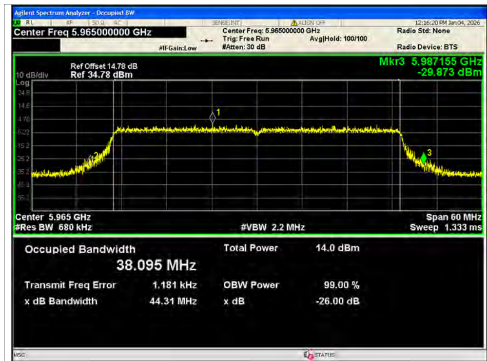
-26dB Bandwidth NVNT ax40 5965MHz Ant1 SISO
