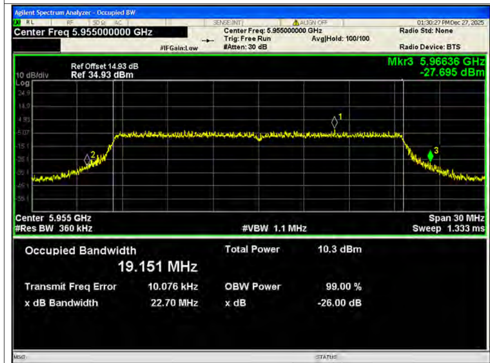
-26dB Bandwidth NVNT ax20 5955MHz Ant2 MIMO
