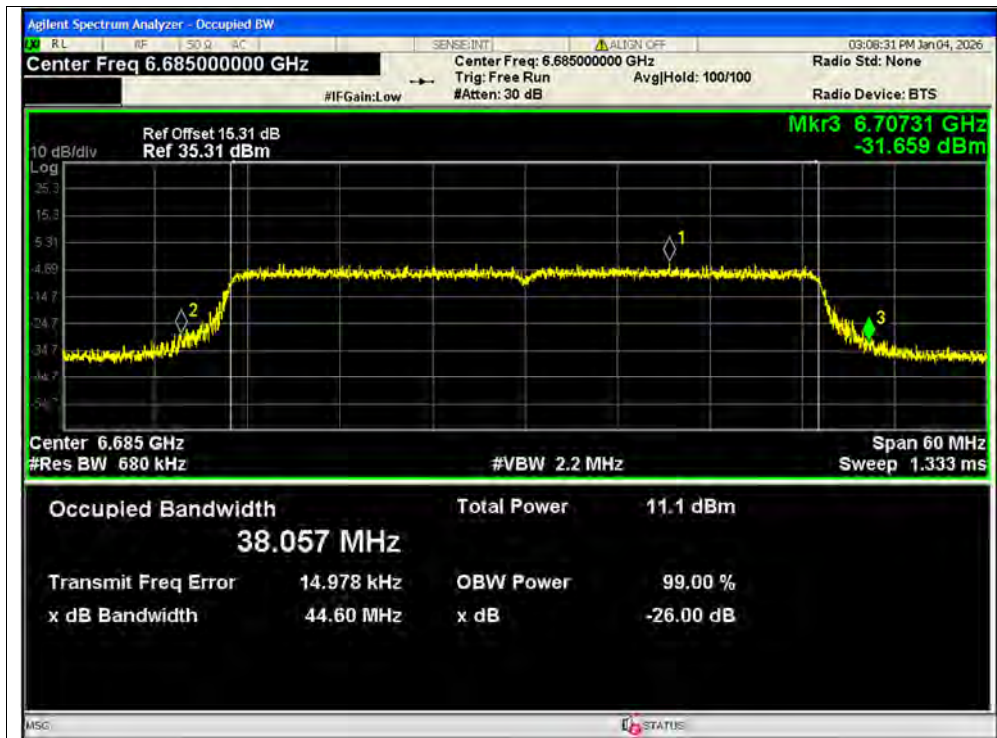
-26dB Bandwidth NVNT ax40 6685MHz Ant1 MIMO
