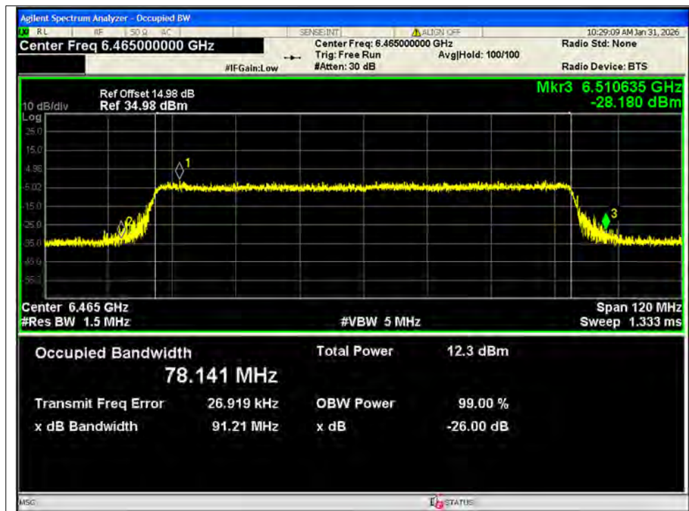
-26dB Bandwidth NVNT ax80 6465MHz Ant1 MIMO
