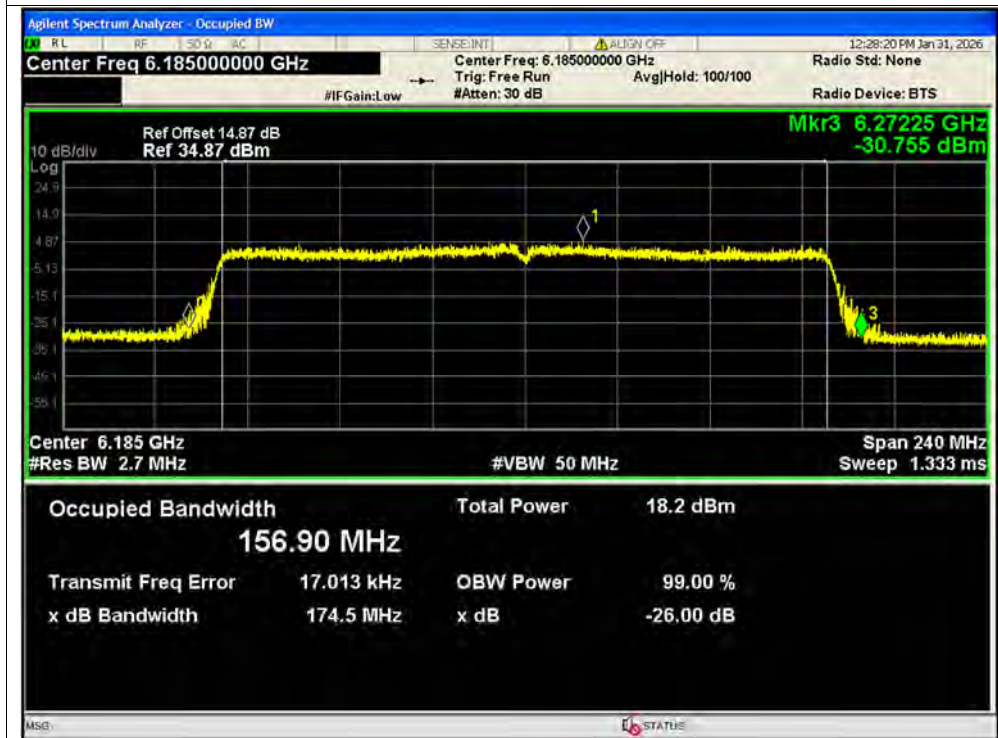
-26dB Bandwidth NVNT ax160 6185MHz Ant2 MIMO
