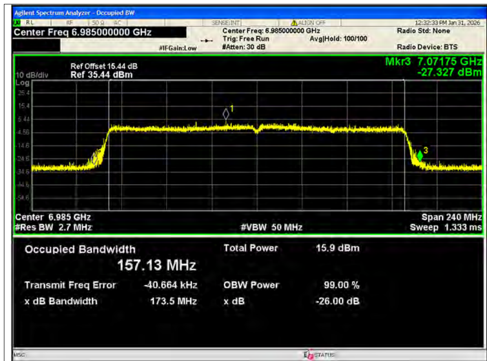
-26dB Bandwidth NVNT ax160 6985MHz Ant1 MIMO
