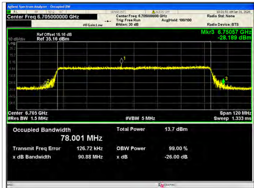
-26dB Bandwidth NVNT ax80 6705MHz Ant1 MIMO
