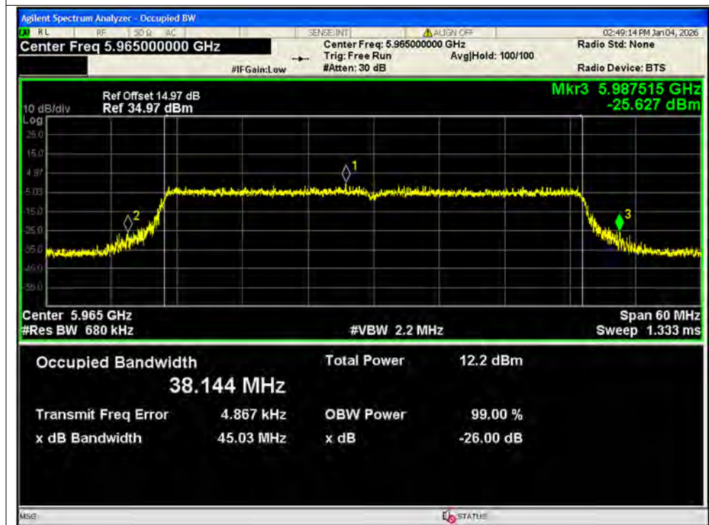
-26dB Bandwidth NVNT ax40 5965MHz Ant2 MIMO
