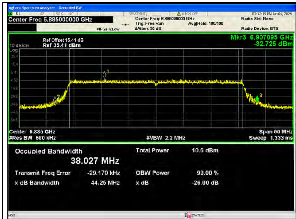
-26dB Bandwidth NVNT ax40 6885MHz Ant1 MIMO
