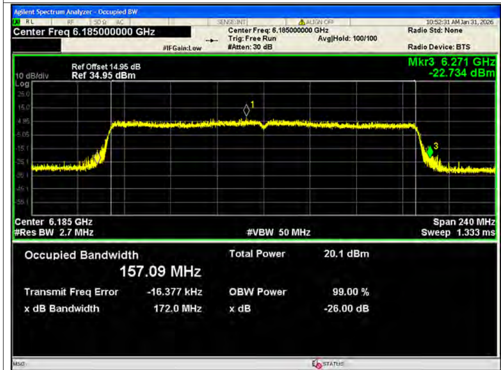
-26dB Bandwidth NVNT ax160 6185MHz Ant1 SISO
