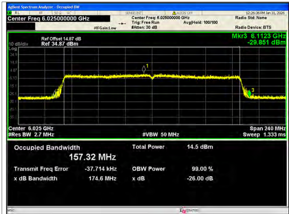
-26dB Bandwidth NVNT ax160 6025MHz Ant1 MIMO
