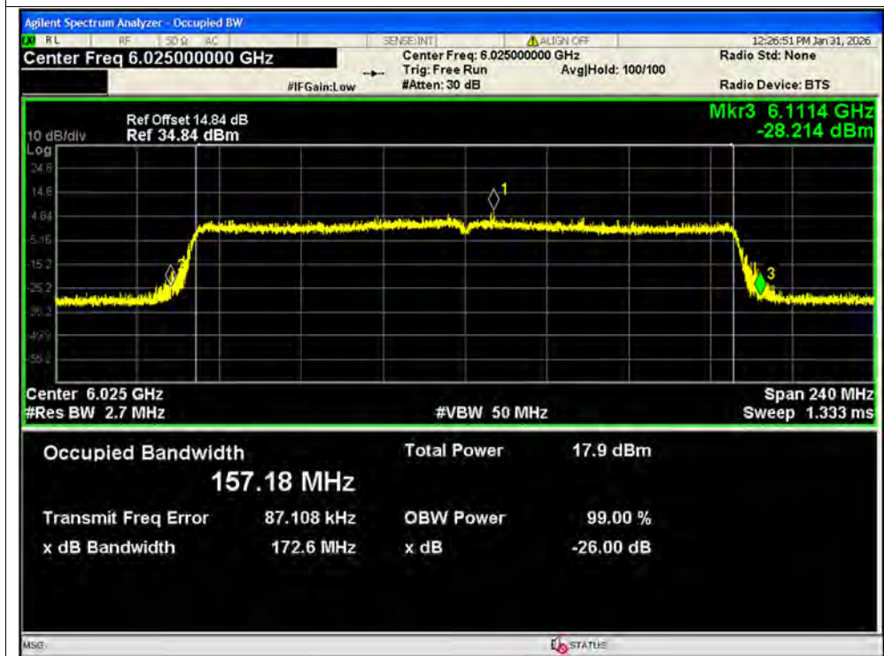
-26dB Bandwidth NVNT ax160 6025MHz Ant2 MIMO
