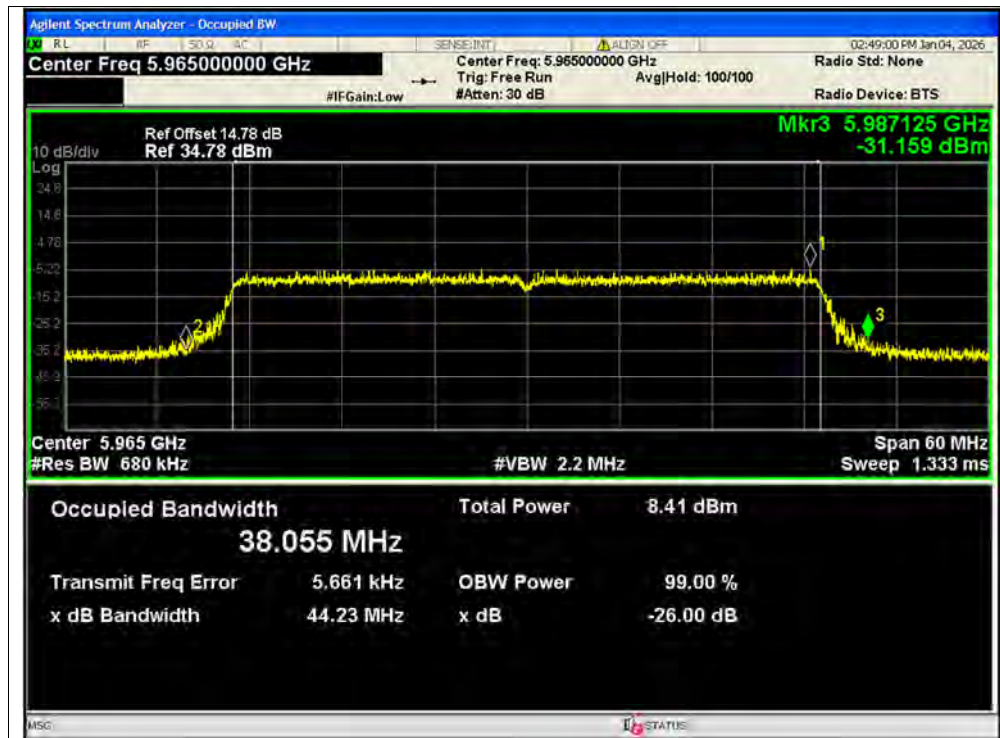
-26dB Bandwidth NVNT ax40 5965MHz Ant1 MIMO
