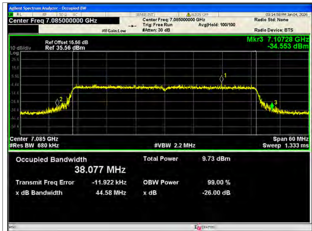
-26dB Bandwidth NVNT ax40 7085MHz Ant1 MIMO
