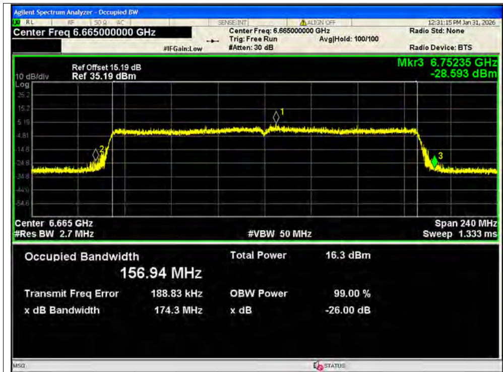
-26dB Bandwidth NVNT ax160 6665MHz Ant1 MIMO
