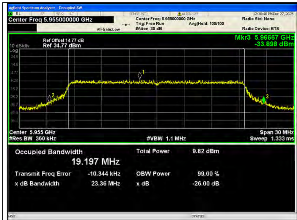
-26dB Bandwidth NVNT ax20 5955MHz Ant1 SISO
