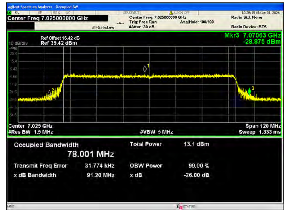
-26dB Bandwidth NVNT ax80 7025MHz Ant1 MIMO
