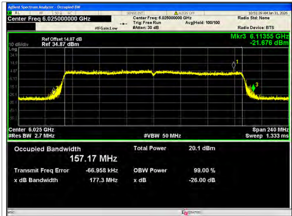
-26dB Bandwidth NVNT ax160 6025MHz Ant1 SISO
