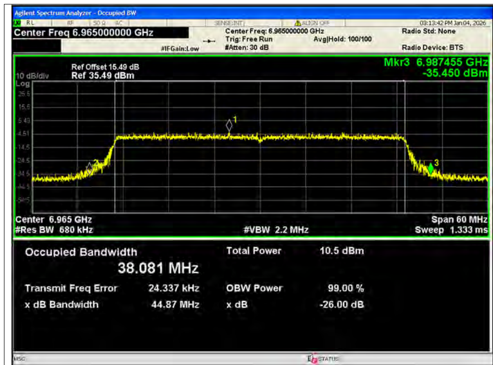
-26dB Bandwidth NVNT ax40 6965MHz Ant1 MIMO
