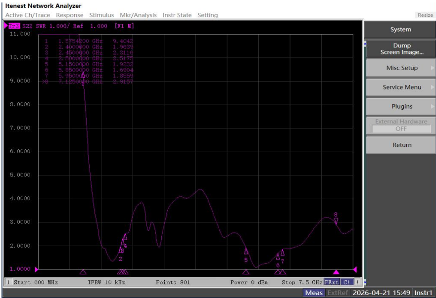
VSWR
