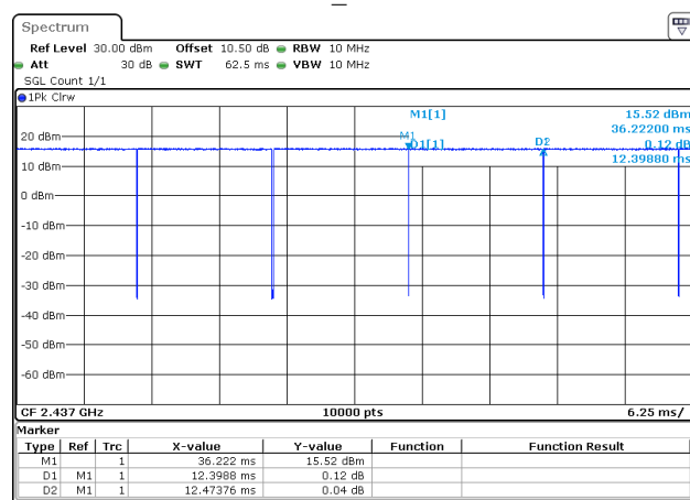
802.11b_2437MHz
