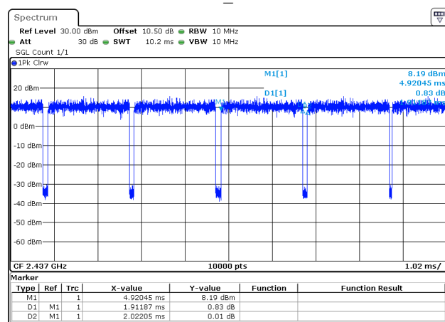
802.11n20_2437MHz
