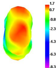
2500.000MHz
