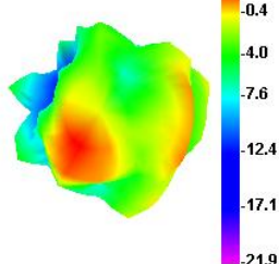
6000.000MHz
