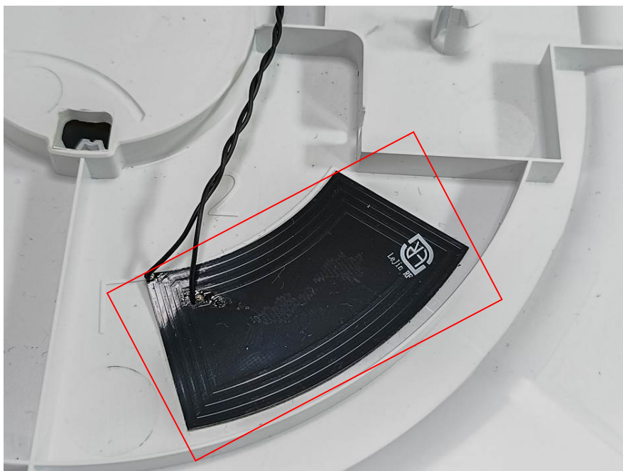
RFID ANT2
