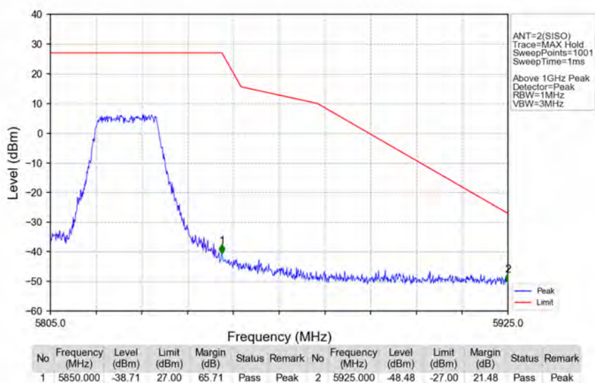
802.11a_HCH_5825MHz_Ant2_NTNV
