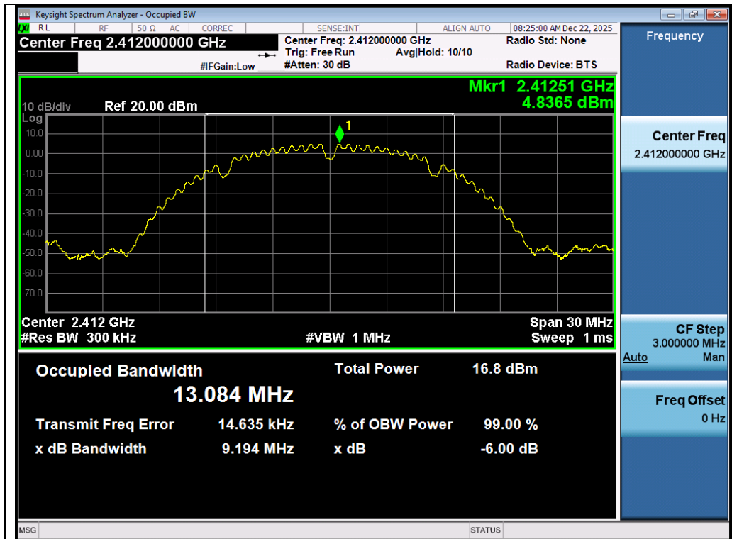
Test_Graph_802.11b_ANT1_2412_1Mbps_DTSBW
