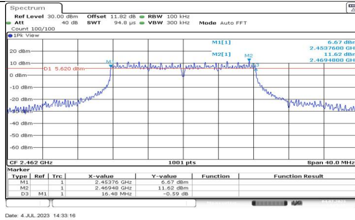
11G-CDD_Ant11_2462
