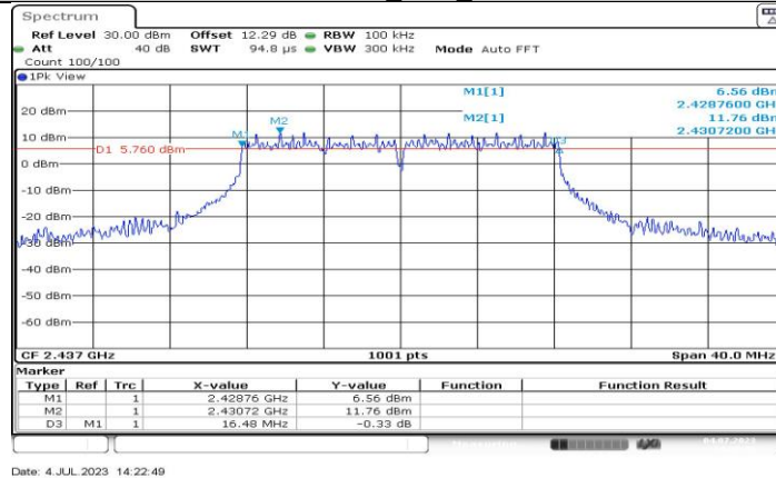
11G-CDD_Ant5_2437
