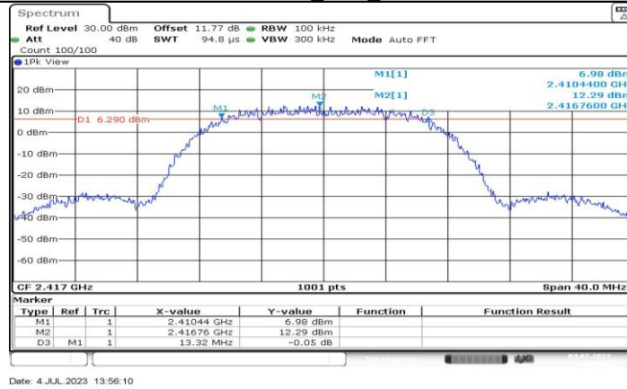
11B-CDD_Ant11_2417
