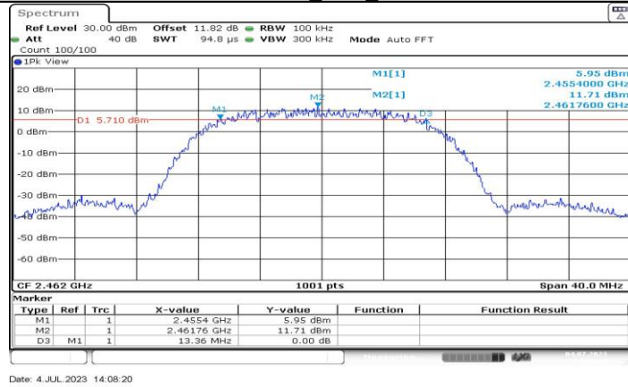
11B-CDD_Ant11_2462
