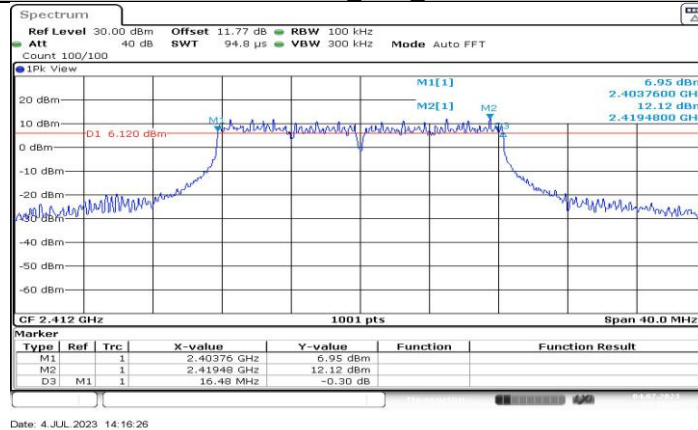
11G-CDD_Ant11_2412
