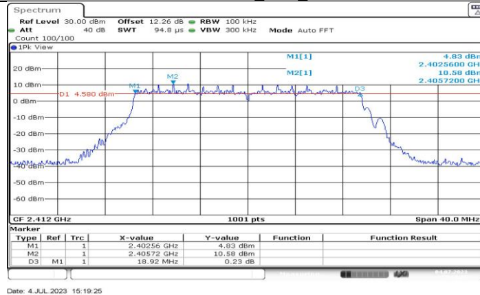
11BE20MIMO_Ant5_2412
