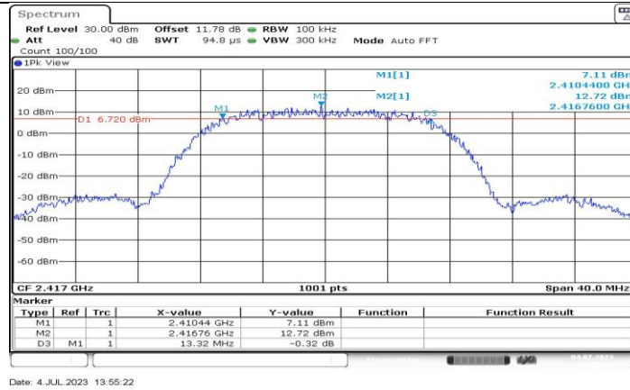
11B-CDD_Ant8_2417
