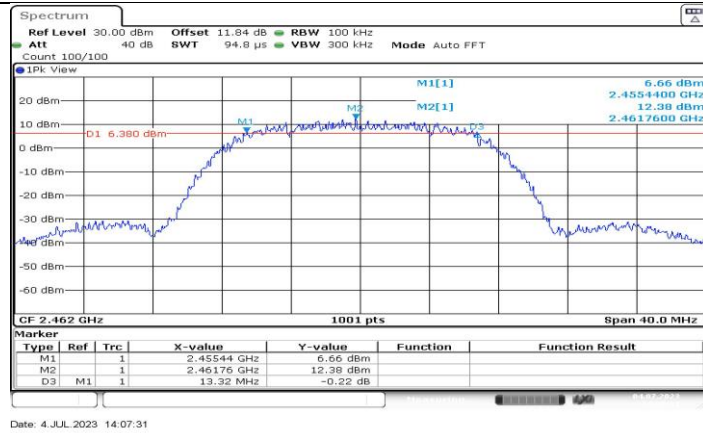
11B-CDD_Ant8_2462
