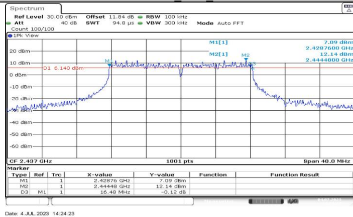
11G-CDD_Ant11_2437
