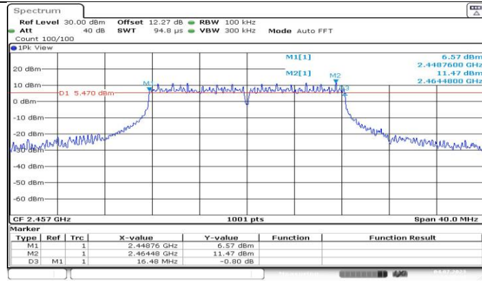
11G-CDD_Ant5_2457
