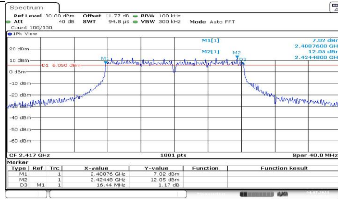
11G-CDD_Ant11_2417
