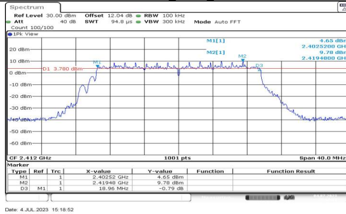
11BE20MIMO_Ant2_2412
