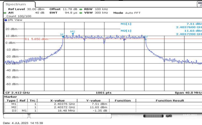
11G-CDD_Ant8_2412
