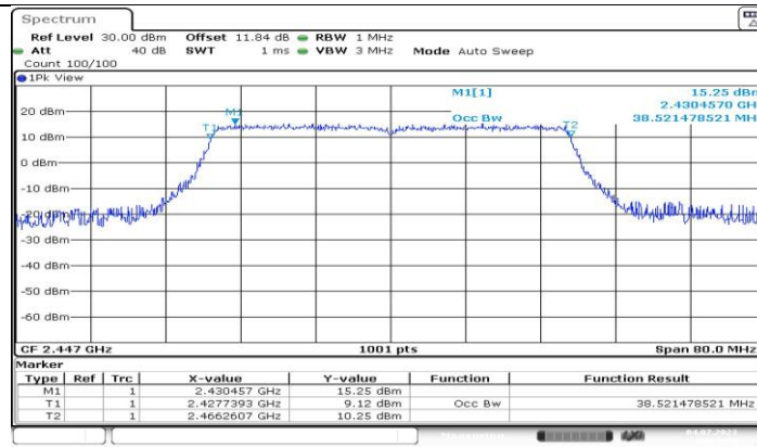
11BE40MIMO_Ant11_2447
