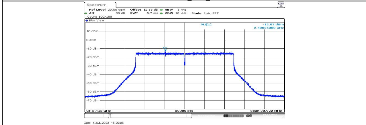
11BE20MIMO_Ant5_2412
