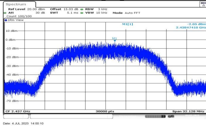
11B-CDD_Ant8_2437
