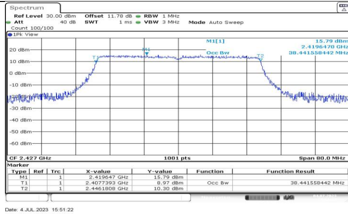
11BE40MIMO_Ant8_2427
