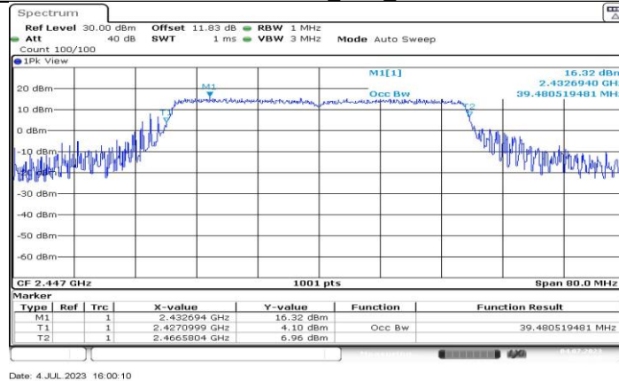
11BE40MIMO_Ant8_2447
