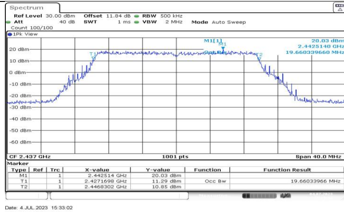
11BE20MIMO_Ant11_2437
