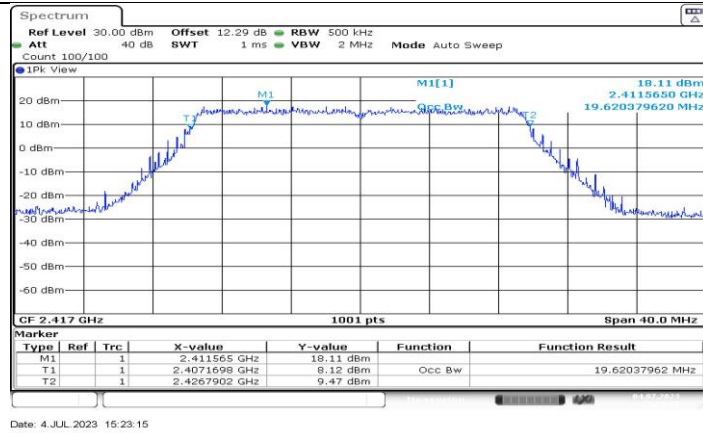
11BE20MIMO_Ant5_2417
