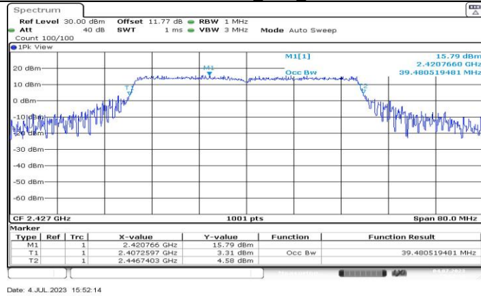
11BE40MIMO_Ant11_2427
