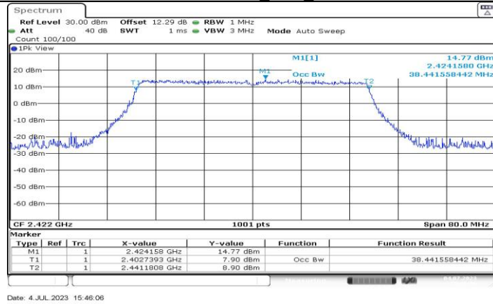
11BE40MIMO_Ant5_2422
