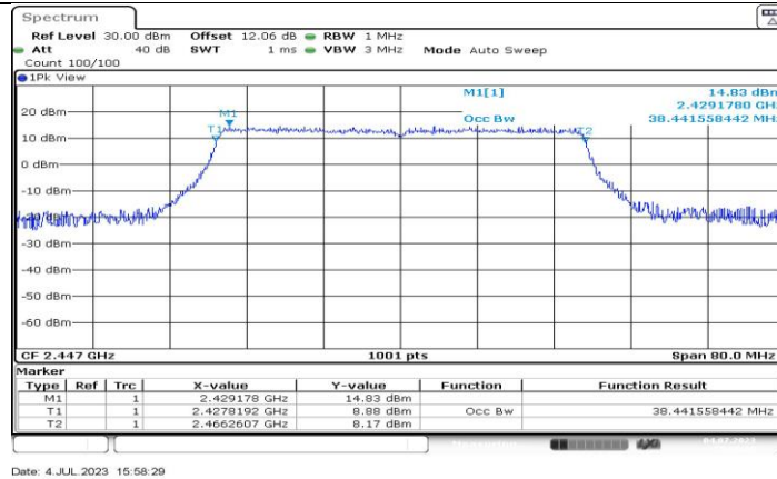
11BE40MIMO_Ant2_2447
