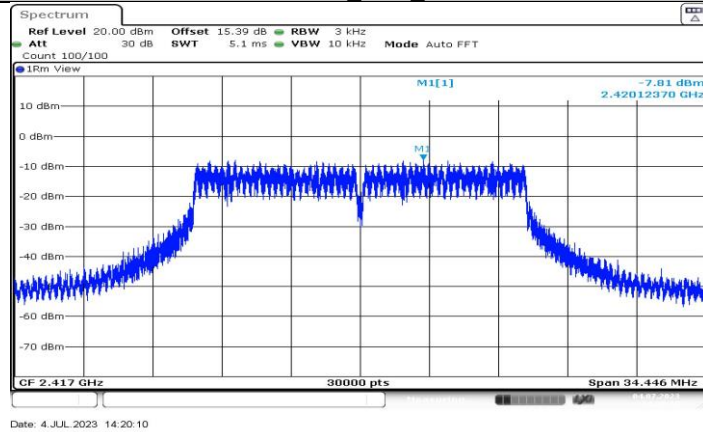
11G-CDD_Ant8_2417
