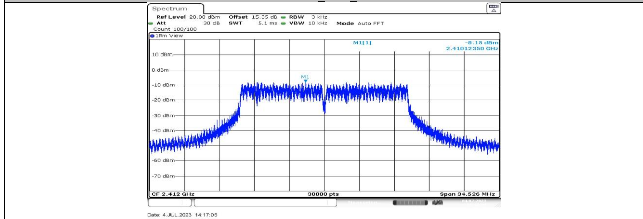
11G-CDD_Ant11_2412
