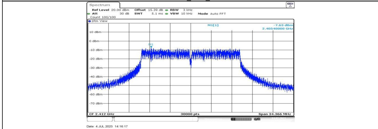
11G-CDD_Ant8_2412
