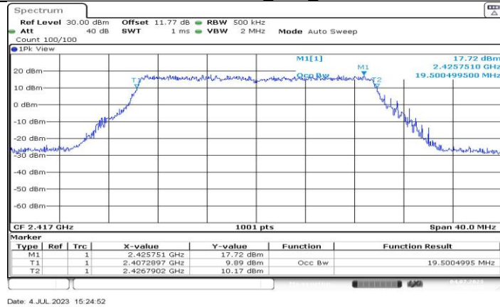
11BE20MIMO_Ant11_2417
