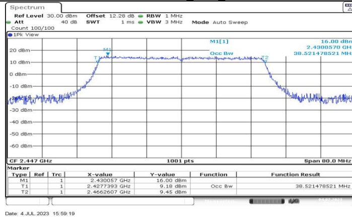
11BE40MIMO_Ant5_2447
