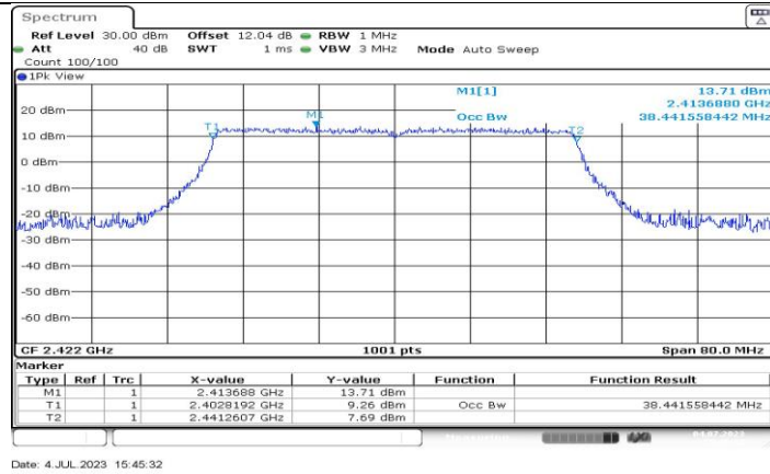
11BE40MIMO_Ant2_2422
