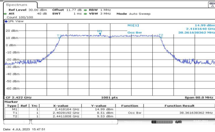
11BE40MIMO_Ant11_2422
