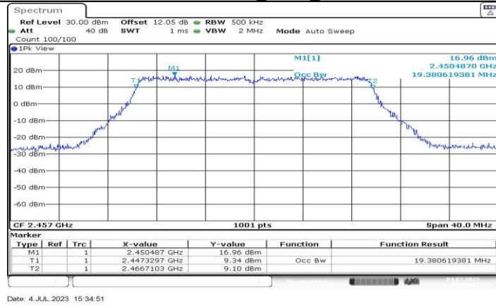
11BE20MIMO_Ant2_2457
