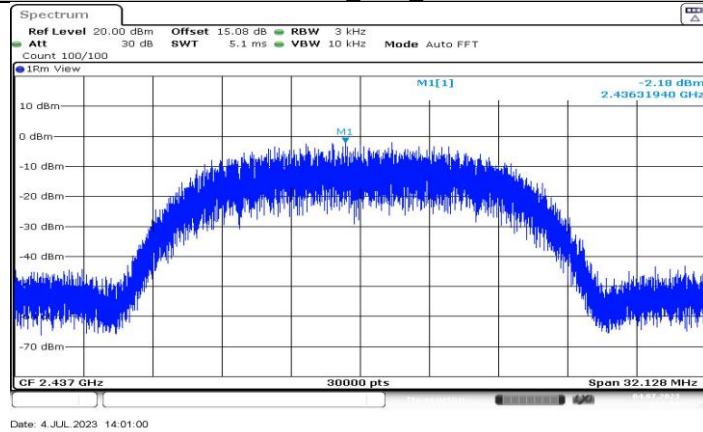
11B-CDD_Ant11_2437
