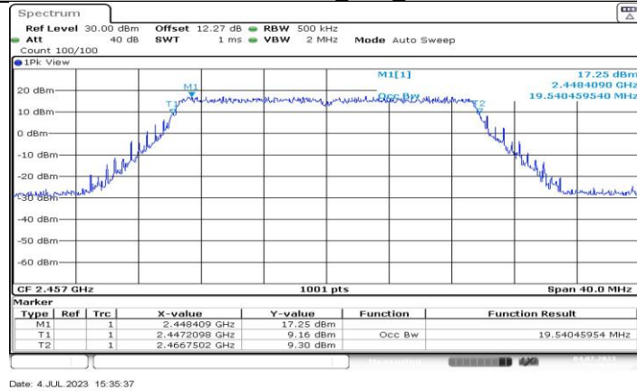
11BE20MIMO_Ant5_2457
