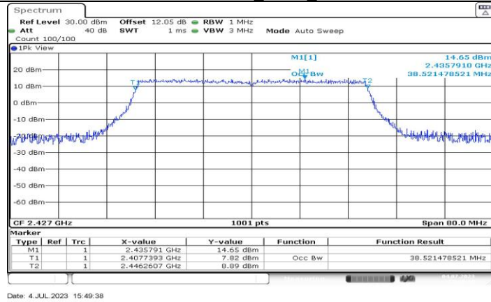
11BE40MIMO_Ant2_2427
