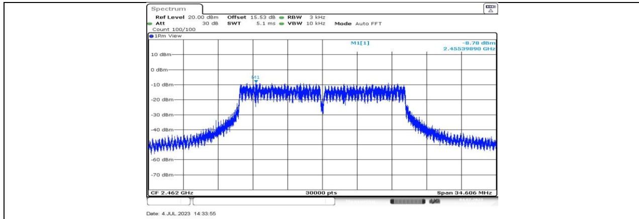
11G-CDD_Ant11_2462
