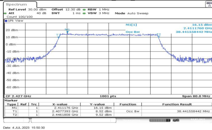
11BE40MIMO_Ant5_2427
