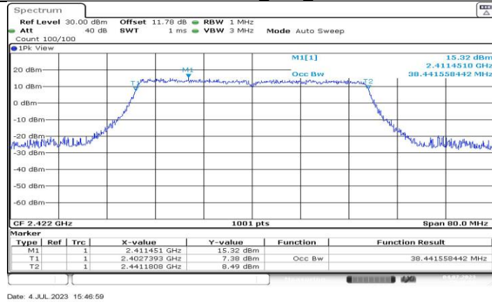
11BE40MIMO_Ant8_2422
