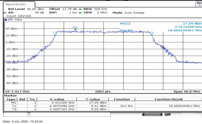
11BE20MIMO_Ant8_2417
