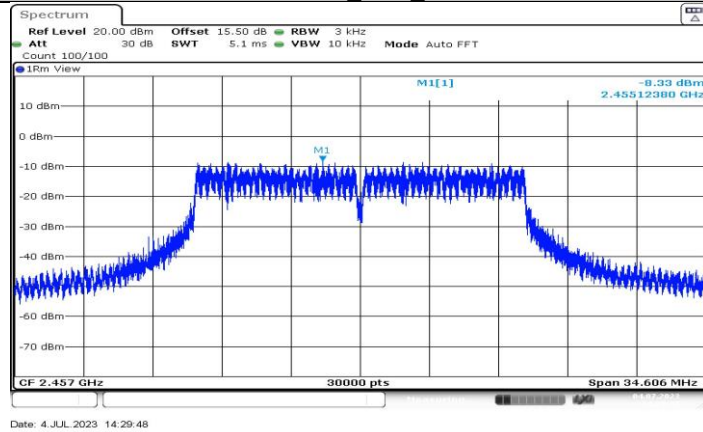
11G-CDD_Ant11_2457
