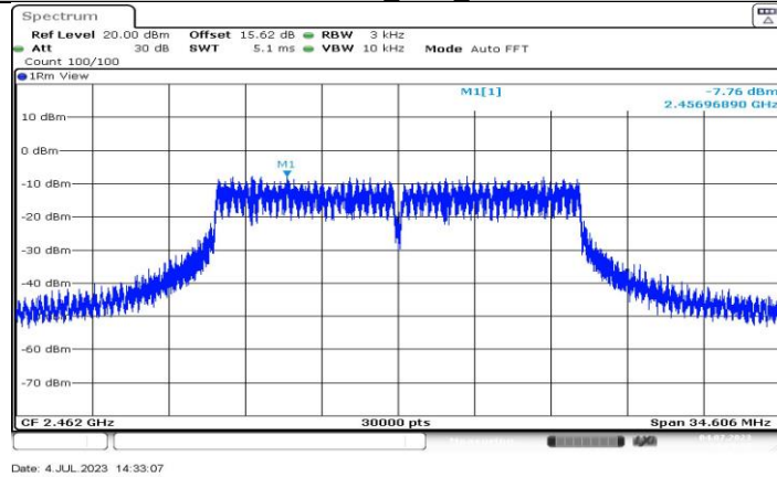
11G-CDD_Ant8_2462
