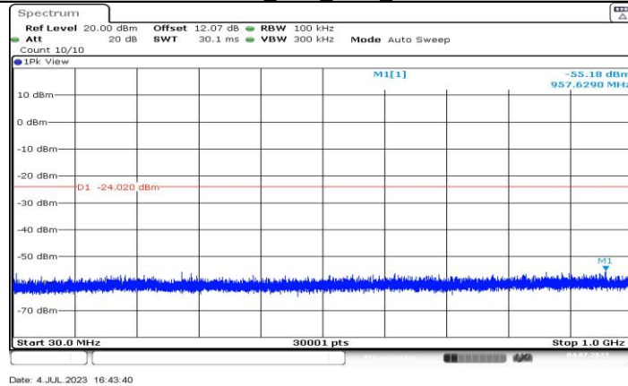
11BE40MIMO_Ant2_2437_30-1000
