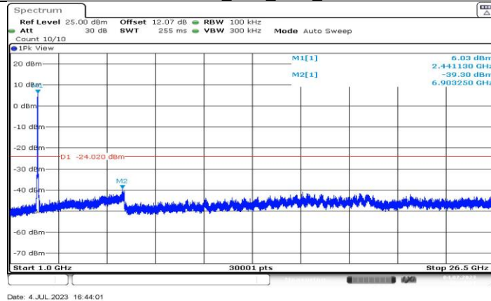
11BE40MIMO_Ant2_2437_1000-26500
