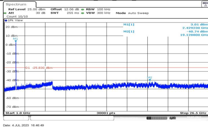
11BE40MIMO_Ant2_2447_1000-26500
