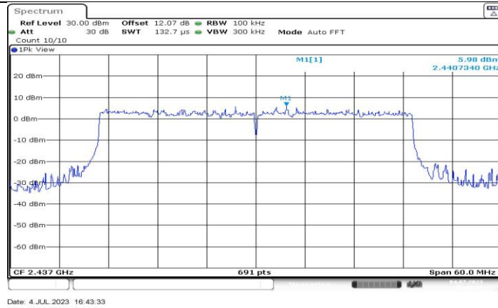
11BE40MIMO_Ant2_2437_0-Reference
