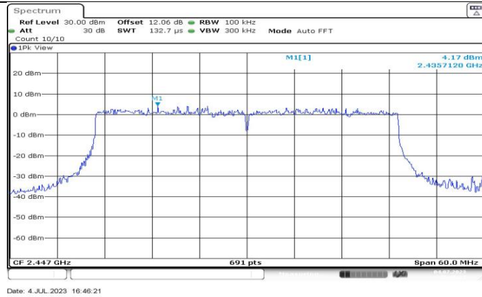
11BE40MIMO_Ant2_2447_0-Reference
