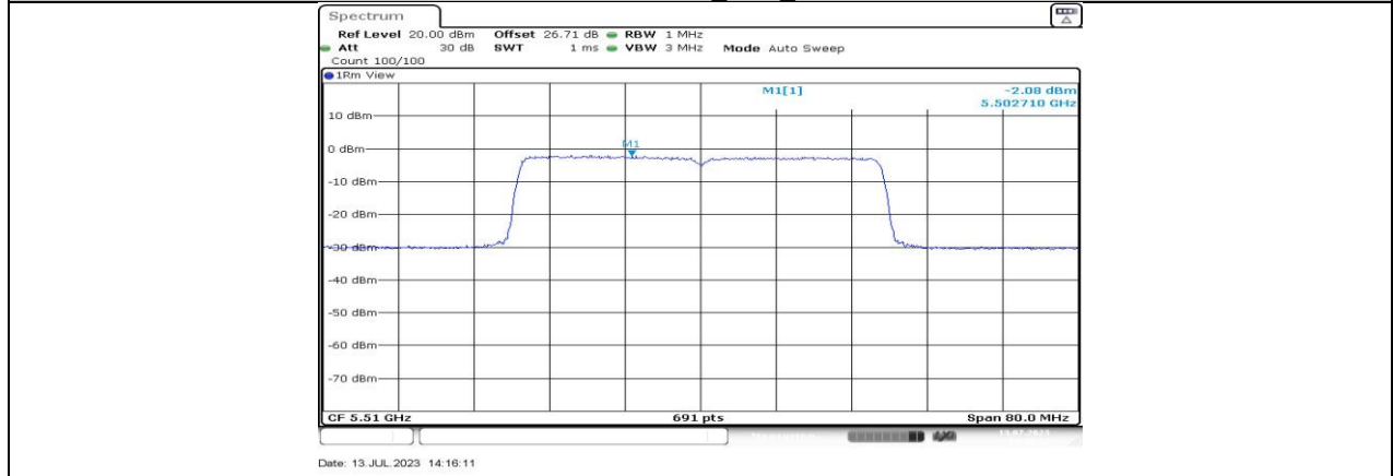
11BE40MIMO_Ant1_5510
