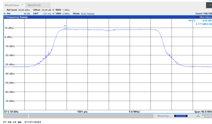
11BE20MIMO_Ant1_5180
