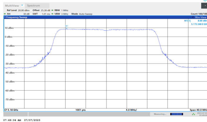
11BE20MIMO_Ant4_5180
