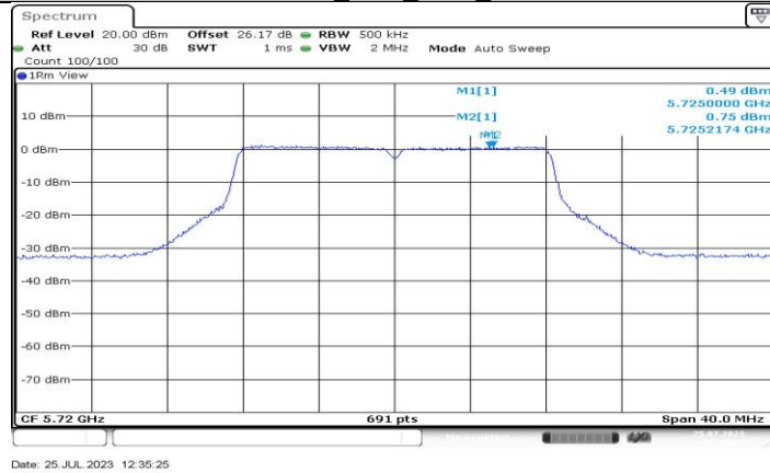
11A-CDD_Ant2_5720_UNII-3
