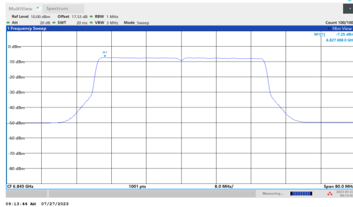
11BE40MIMO_Ant1_6845
