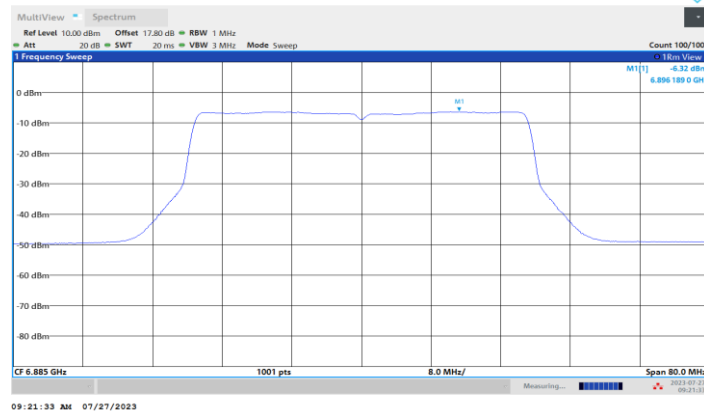
11BE40MIMO_Ant3_6885
