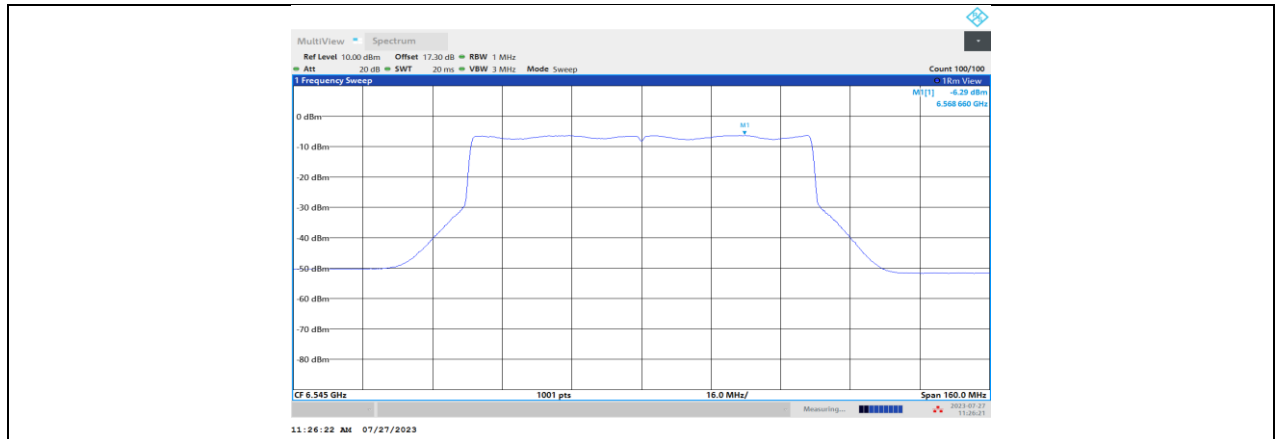
11BE80MIMO_Ant3_6545
