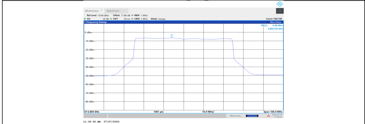
11BE80MIMO_Ant3_6865
