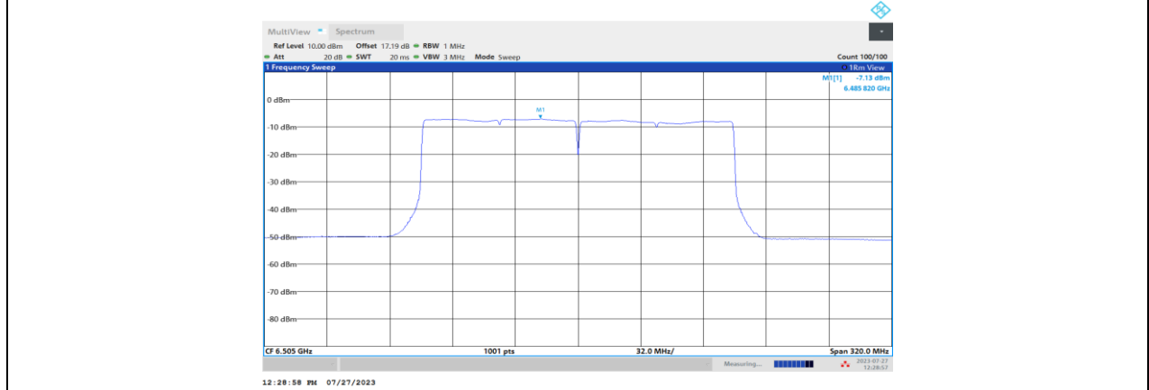
11BE160MIMO_Ant1_6505
