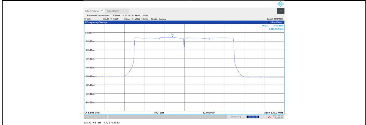
11BE160MIMO_Ant4_6505
