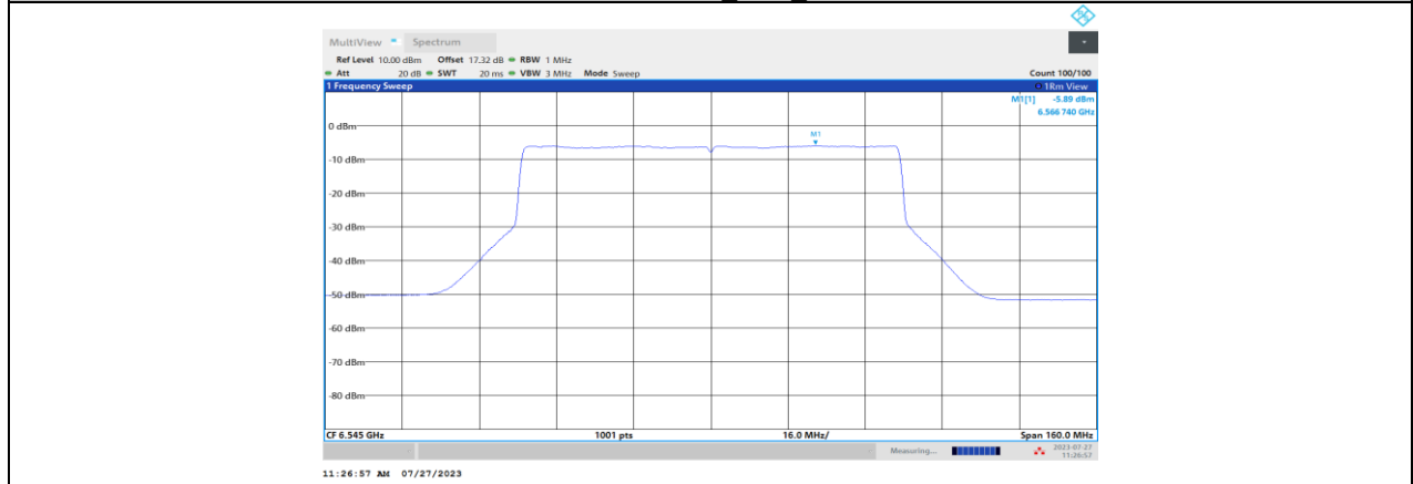
11BE80MIMO_Ant4_6545
