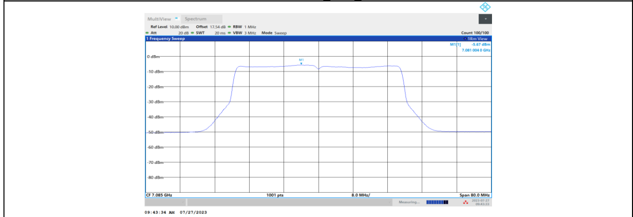
11BE40MIMO_Ant3_7085
