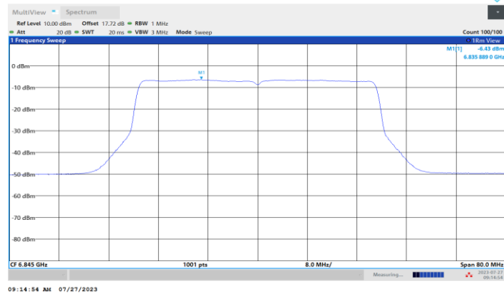
11BE40MIMO_Ant3_6845
