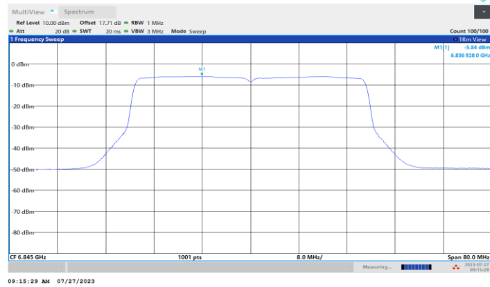
11BE40MIMO_Ant4_6845
