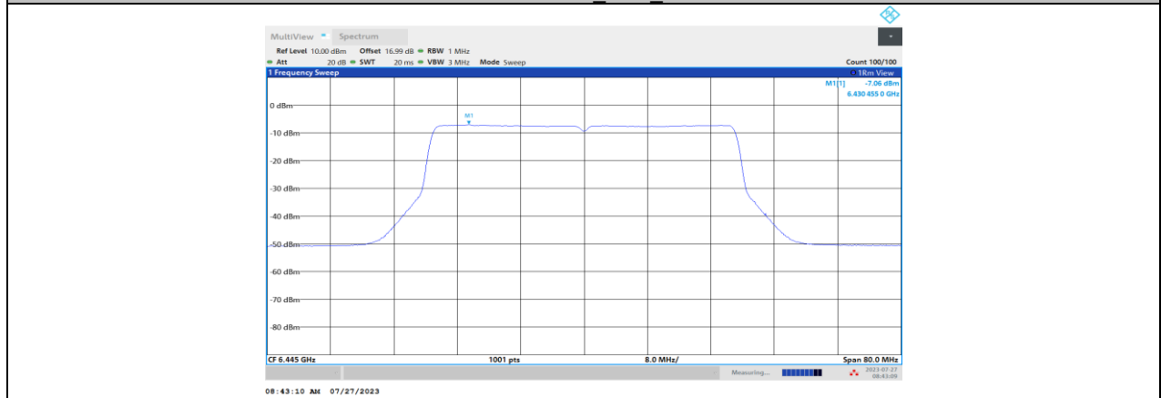
11BE40MIMO_Ant2_6445
