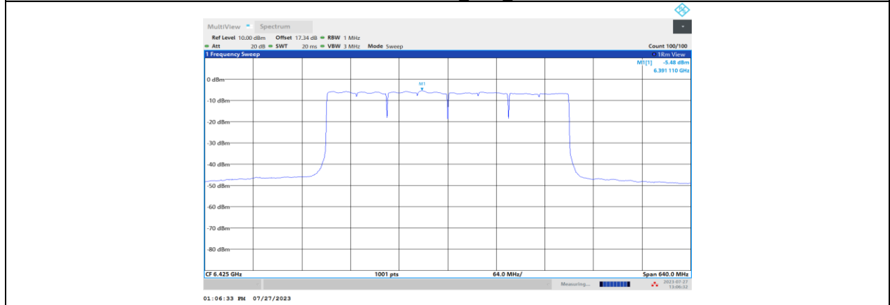
11BE320MIMO_Ant4_6425
