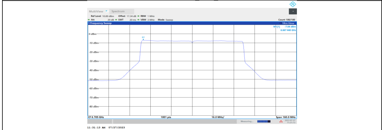
11BE80MIMO_Ant1_6705
