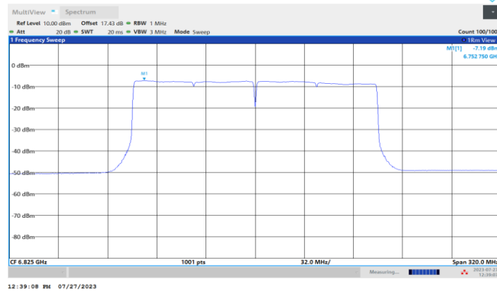
11BE160MIMO_Ant2_6825
