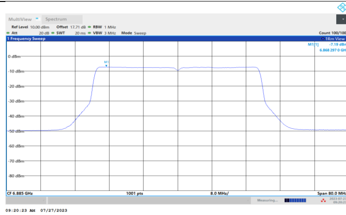
11BE40MIMO_Ant1_6885
