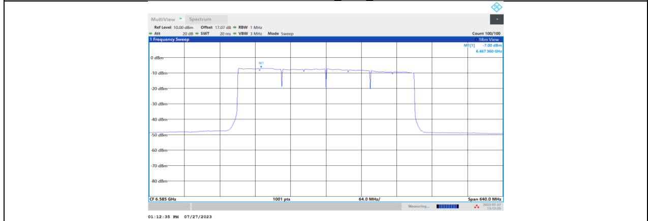
11BE320MIMO_Ant1_6585
