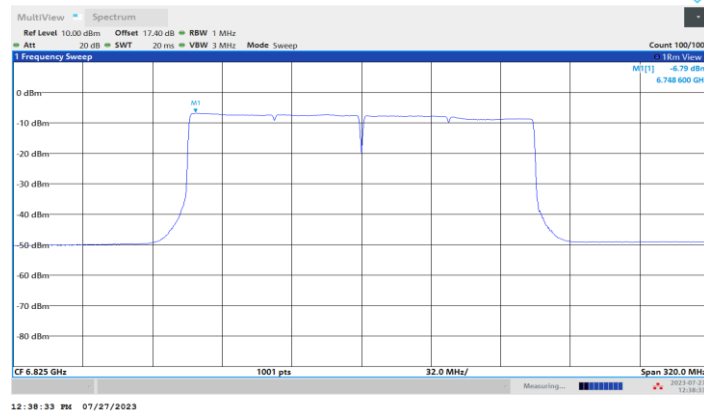
11BE160MIMO_Ant1_6825
