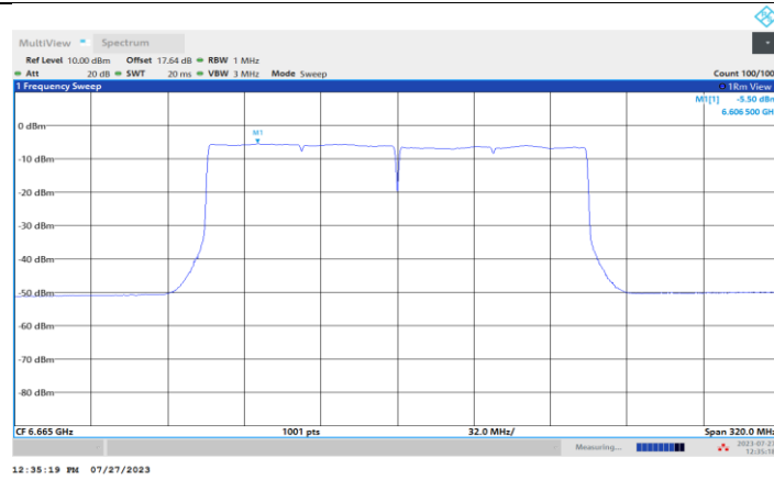
11BE160MIMO_Ant4_6665
