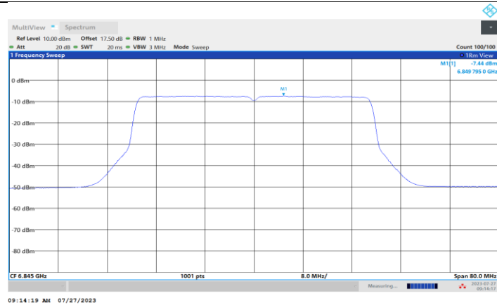
11BE40MIMO_Ant2_6845
