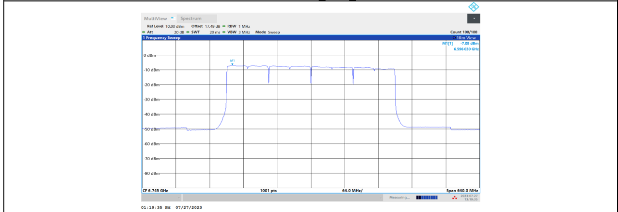
11BE320MIMO_Ant2_6745
