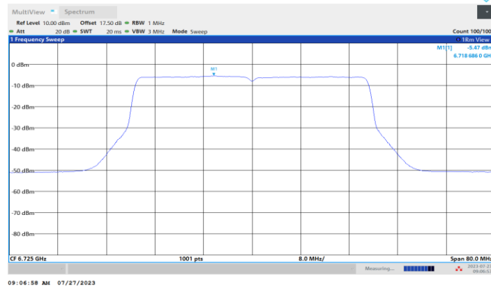
11BE40MIMO_Ant4_6725
