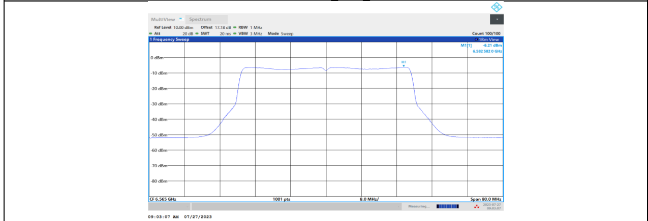
11BE40MIMO_Ant3_6565
