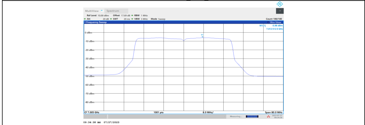
11BE40MIMO_Ant4_7005
