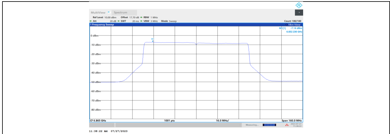
11BE80MIMO_Ant1_6865
