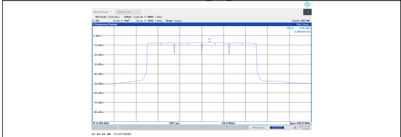
11BE320MIMO_Ant2_6265
