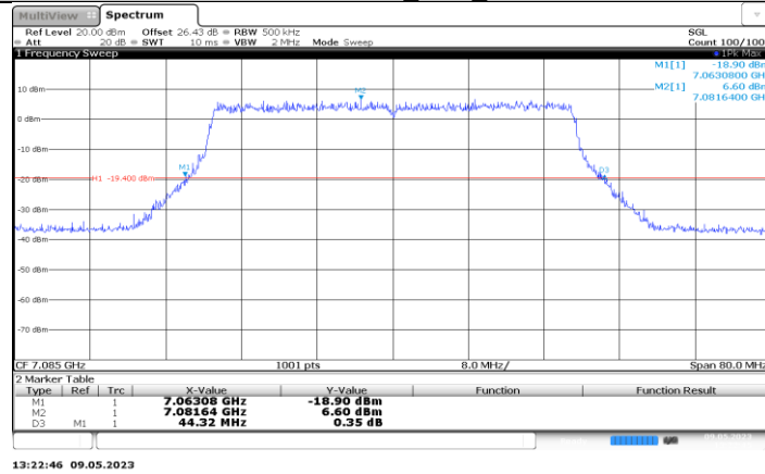
11AX40MIMO_Ant3_7085
