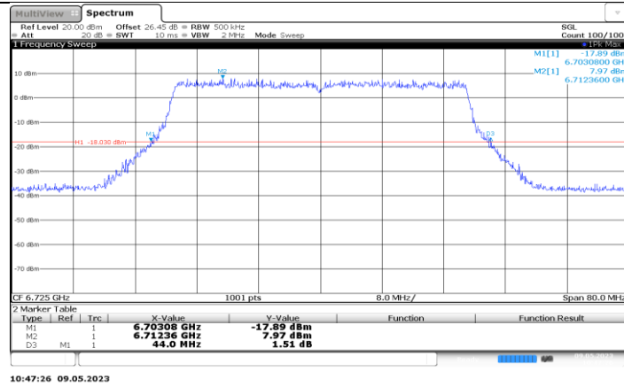
11AX40MIMO_Ant3_6725
