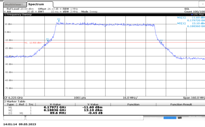
11AX80MIMO_Ant6_6225
