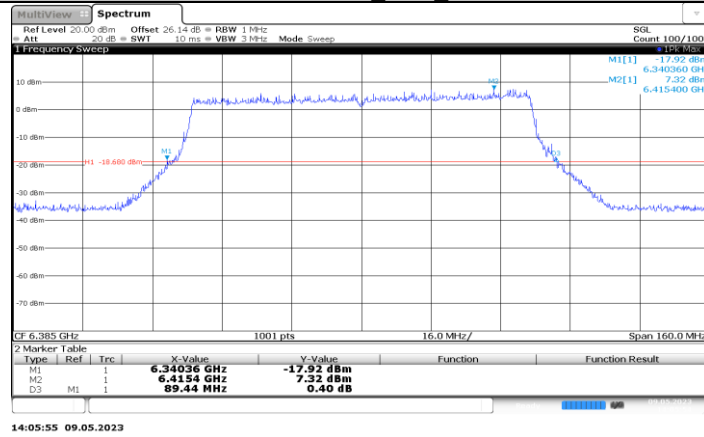
11AX80MIMO_Ant3_6385
