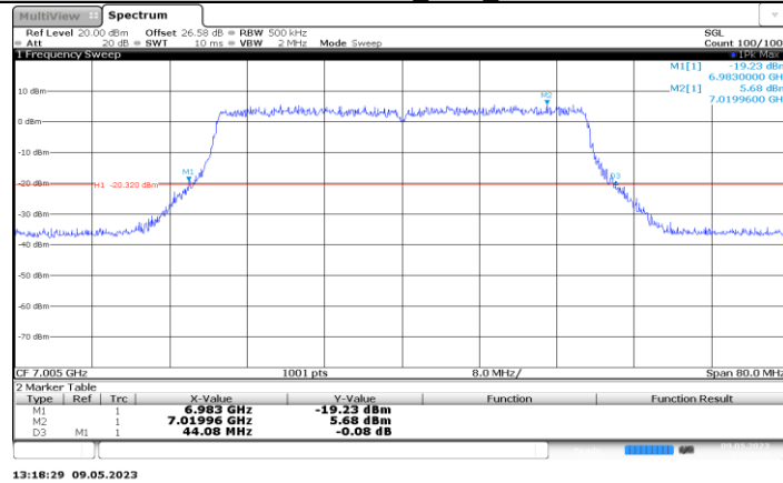
11AX40MIMO_Ant6_7005
