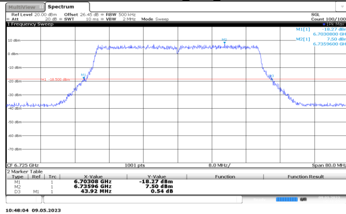
11AX40MIMO_Ant6_6725
