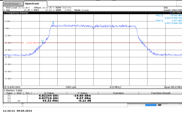
11AX40MIMO_Ant3_6845
