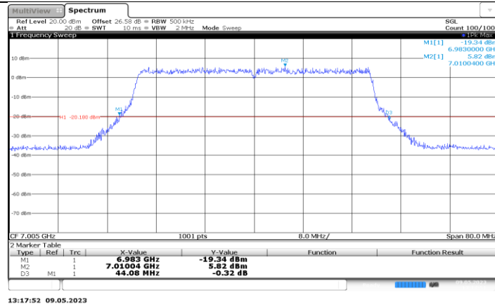
11AX40MIMO_Ant3_7005
