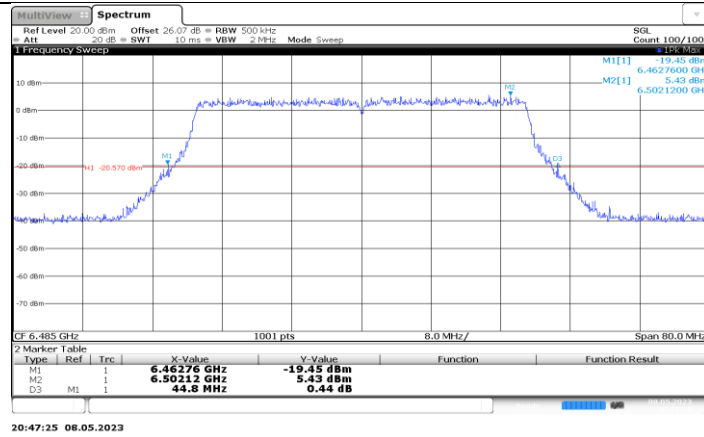
11AX40MIMO_Ant6_6485
