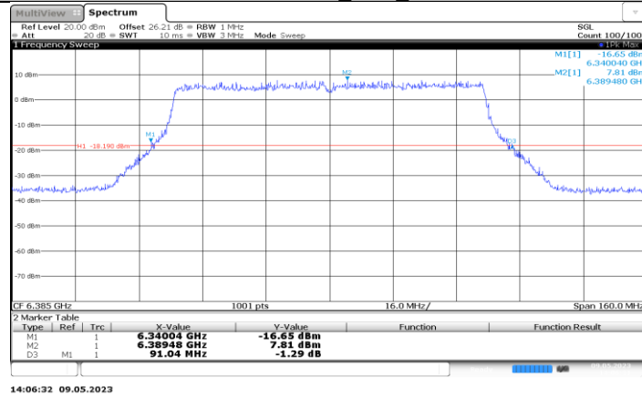
11AX80MIMO_Ant6_6385
