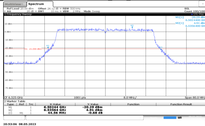
11AX40MIMO_Ant6_6525
