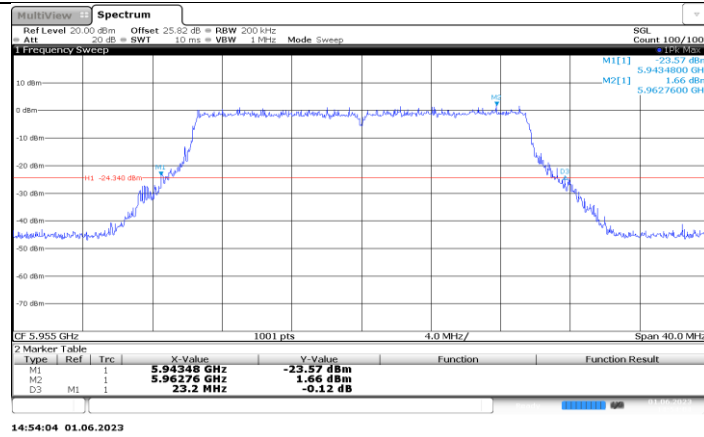
11BE20MIMO_Ant6_5955
