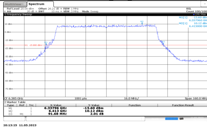
11BE80MIMO_Ant6_6385
