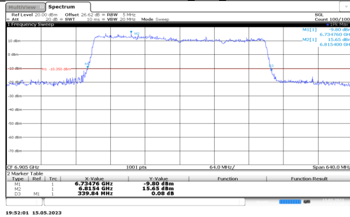
11BE320MIMO_Ant6_6905
