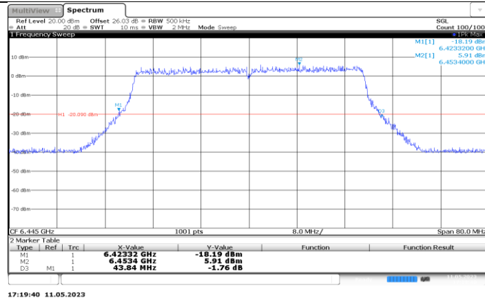
11BE40MIMO_Ant6_6445
