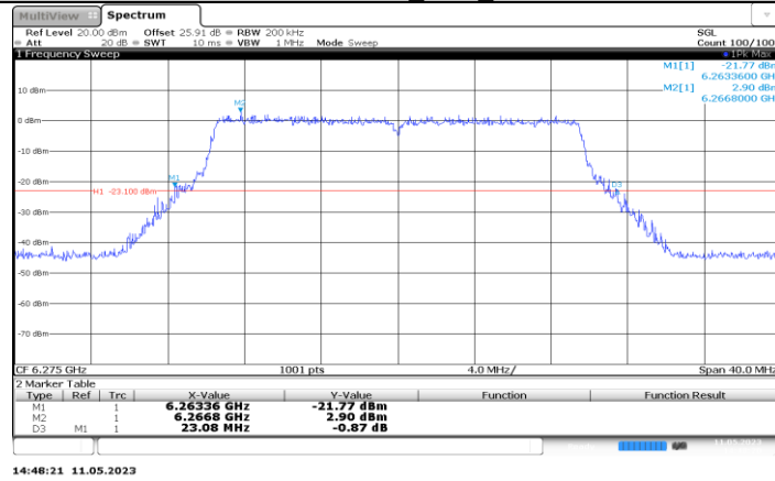
11BE20MIMO_Ant6_6275
