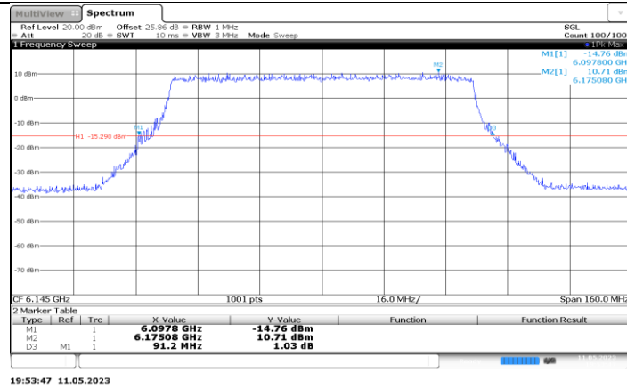
11BE80MIMO_Ant6_6145
