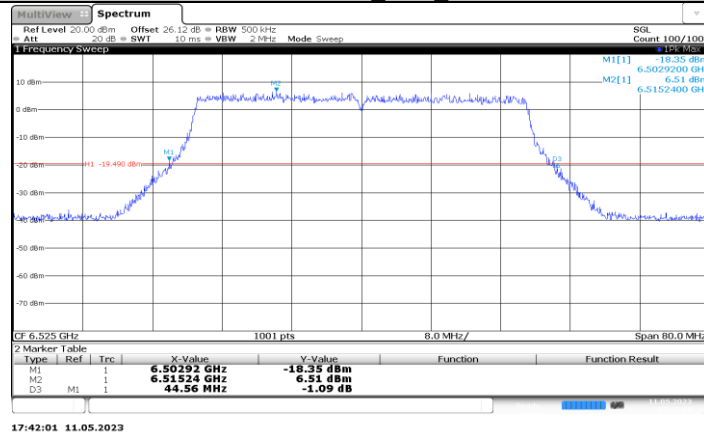
11BE40MIMO_Ant6_6525
