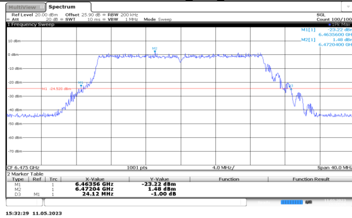
11BE20MIMO_Ant6_6475
