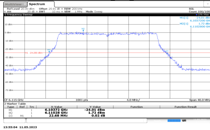
11BE20MIMO_Ant3_6115
