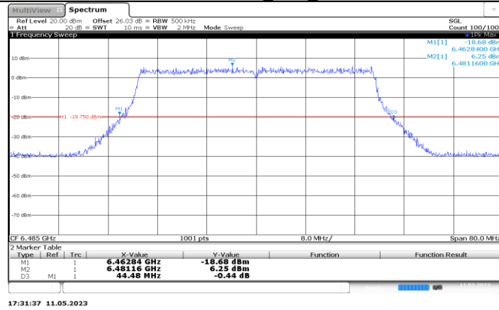
11BE40MIMO_Ant3_6485
