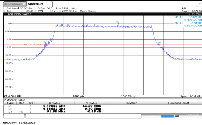
11BE80MIMO_Ant6_6545
