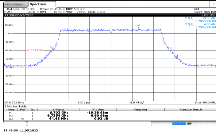
11BE40MIMO_Ant3_6725
