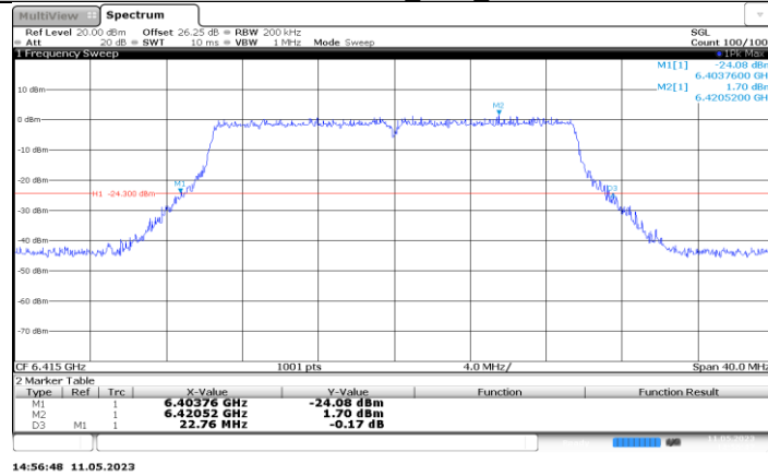
11BE20MIMO_Ant3_6415
