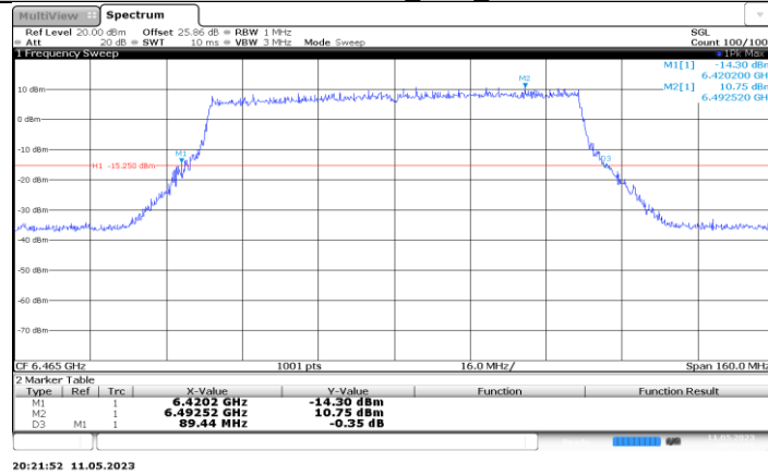
11BE80MIMO_Ant3_6465
