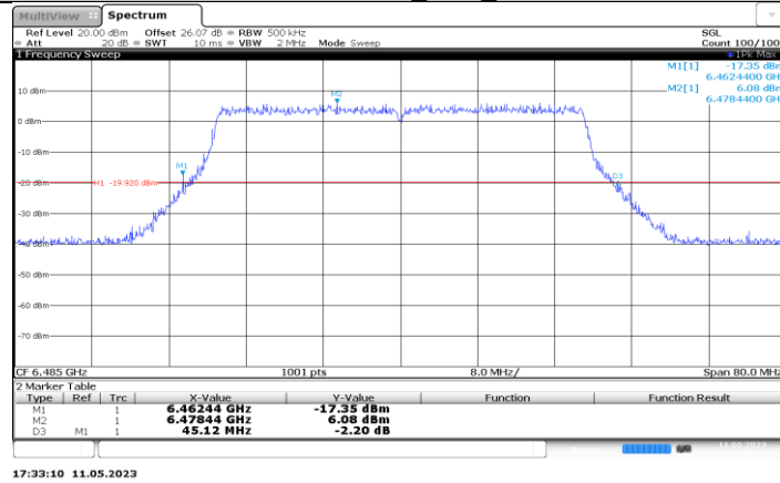
11BE40MIMO_Ant6_6485
