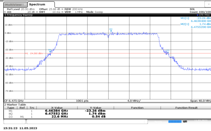
11BE20MIMO_Ant3_6475
