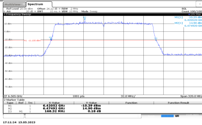
11BE160MIMO_Ant6_6505
