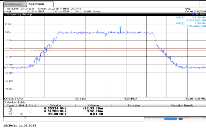
11BE20MIMO_Ant3_6515
