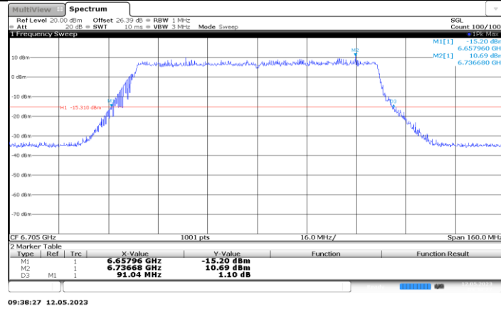
11BE80MIMO_Ant3_6705
