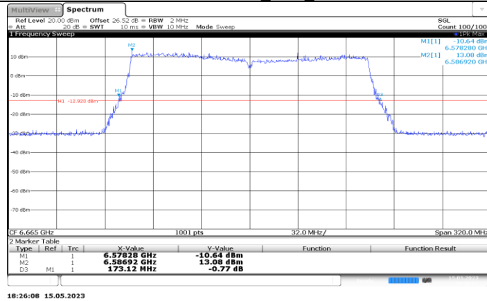
11BE160MIMO_Ant3_6665
