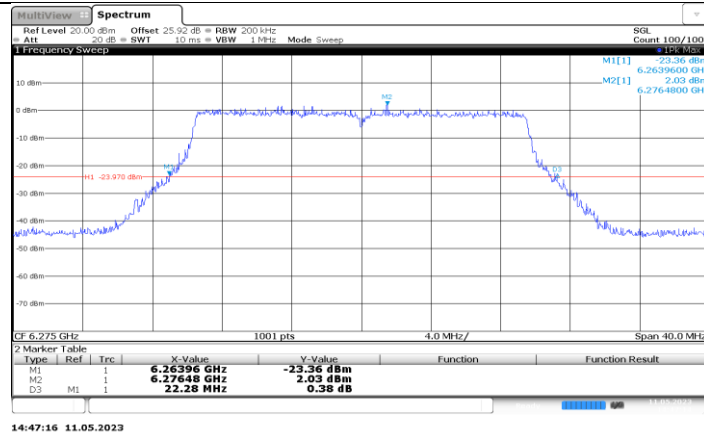
11BE20MIMO_Ant3_6275
