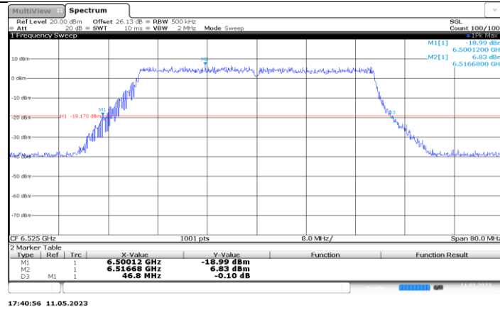
11BE40MIMO_Ant3_6525
