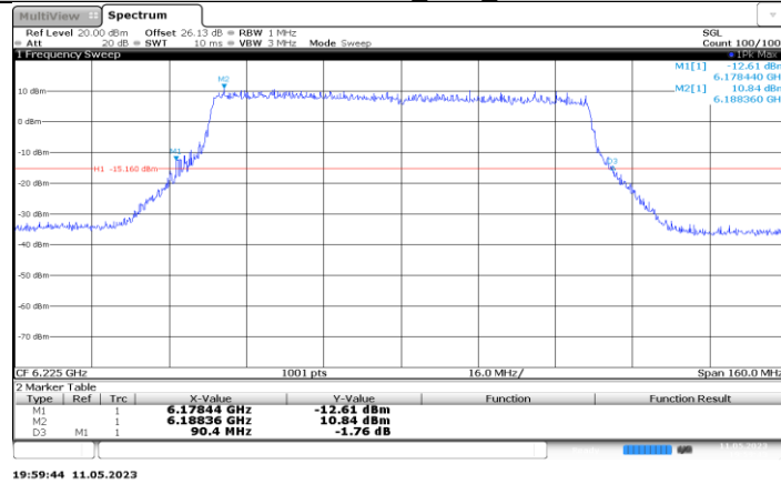
11BE80MIMO_Ant6_6225
