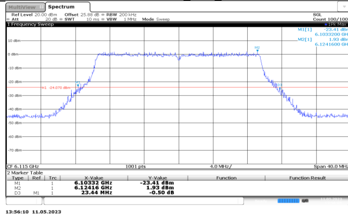
11BE20MIMO_Ant6_6115
