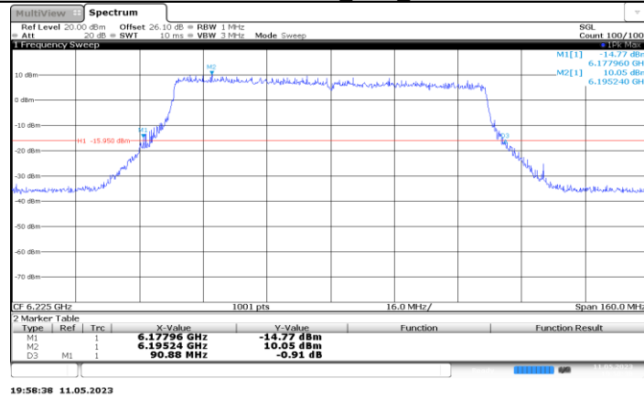
11BE80MIMO_Ant3_6225
