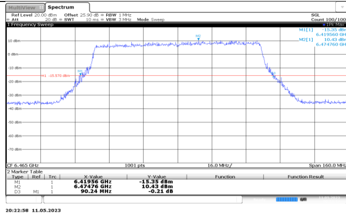
11BE80MIMO_Ant6_6465
