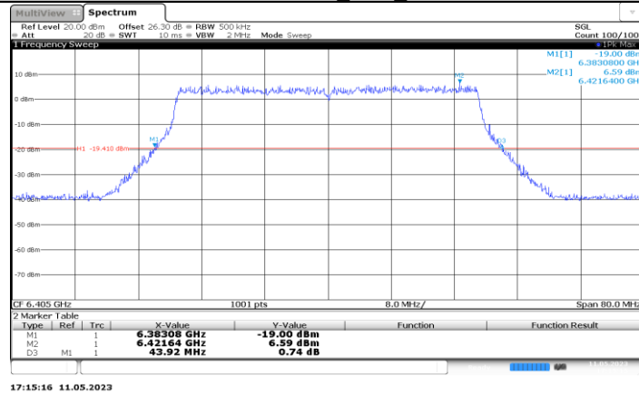
11BE40MIMO_Ant6_6405
