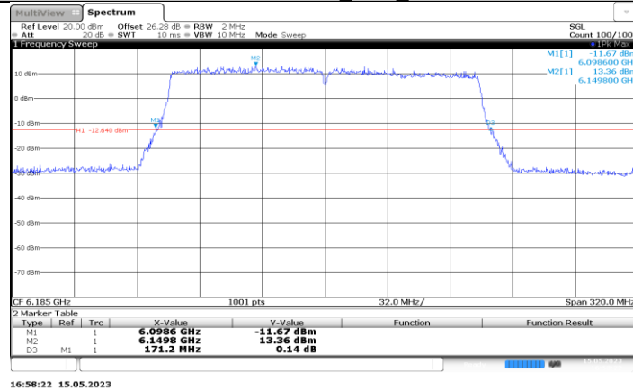
11BE160MIMO_Ant6_6185
