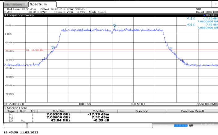
11BE40MIMO_Ant6_7085
