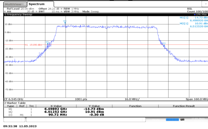
11BE80MIMO_Ant3_6545
