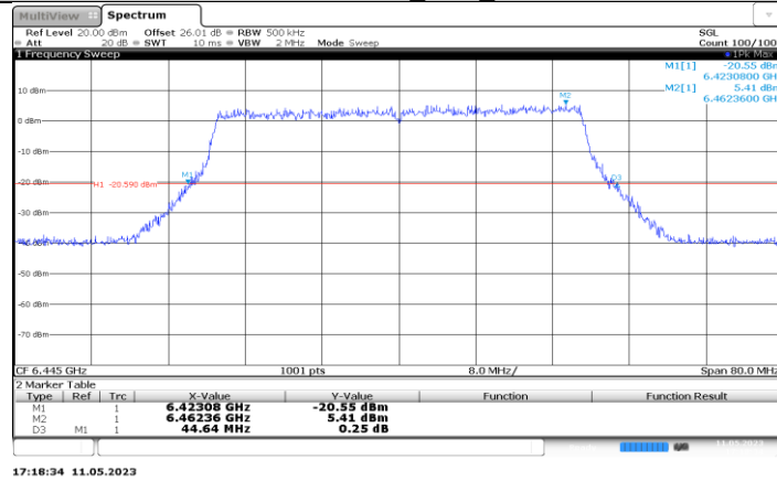
11BE40MIMO_Ant3_6445
