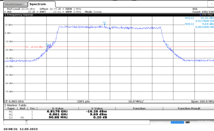
11BE80MIMO_Ant3_6865
