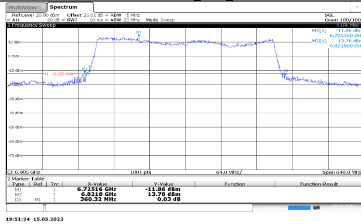
11BE320MIMO_Ant3_6905
