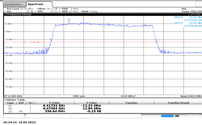
11BE320MIMO_Ant6_6585
