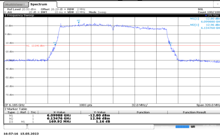
11BE160MIMO_Ant3_6185
