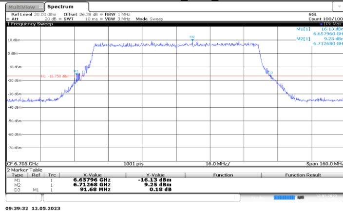
11BE80MIMO_Ant6_6705
