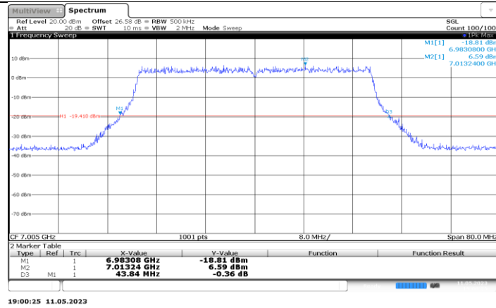
11BE40MIMO_Ant6_7005
