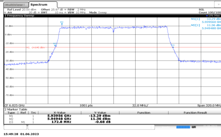
11BE160MIMO_Ant6_6025
