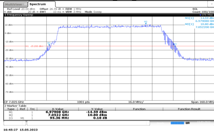
11BE80MIMO_Ant6_7025
