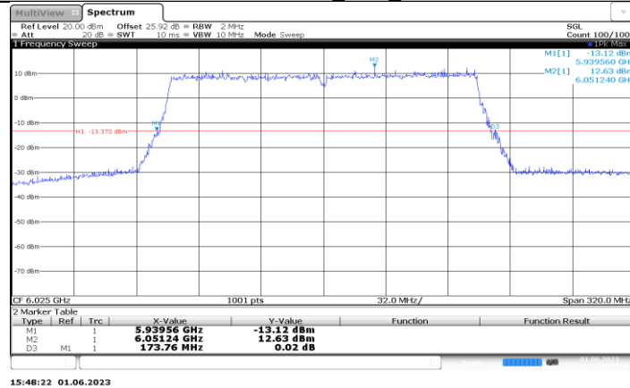
11BE160MIMO_Ant3_6025
