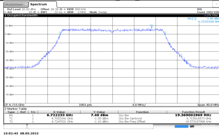
11AX20MIMO_Ant6_6715
