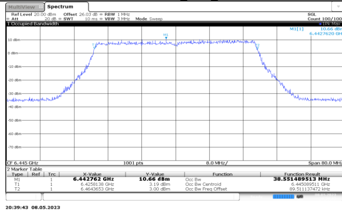
11AX40MIMO_Ant6_6445
