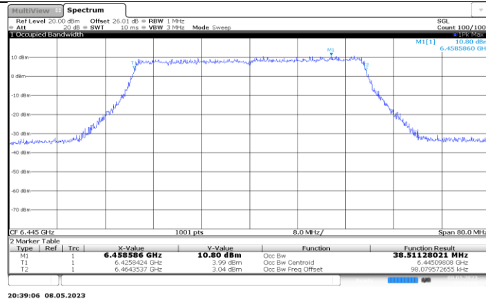
11AX40MIMO_Ant3_6445
