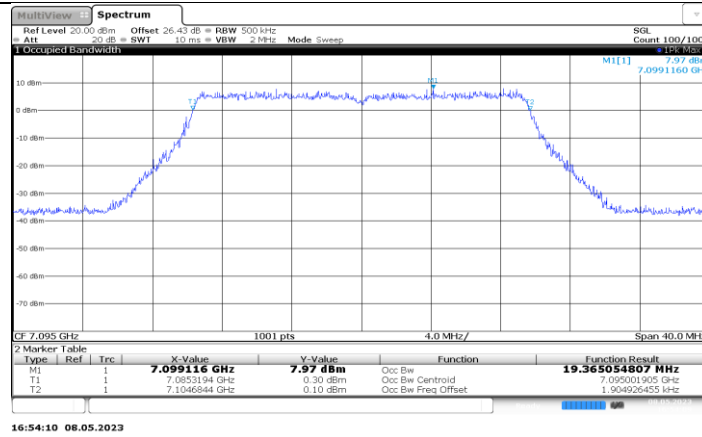
11AX20MIMO_Ant3_7095
