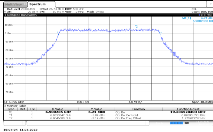
11BE20MIMO_Ant3_6895
