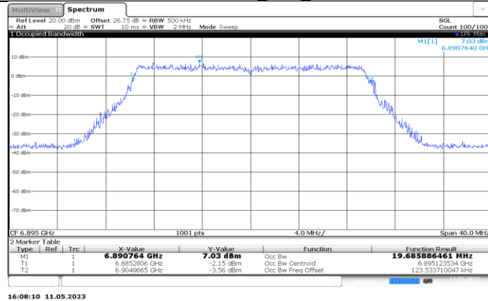
11BE20MIMO_Ant6_6895
