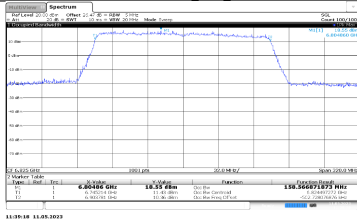
11AX160MIMO_Ant6_6825
