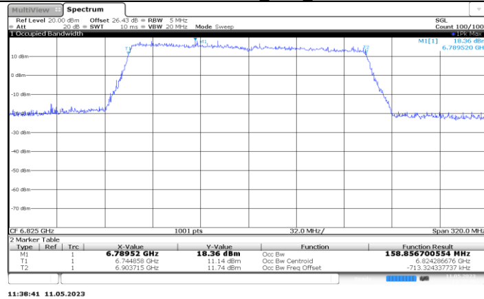
11AX160MIMO_Ant3_6825
