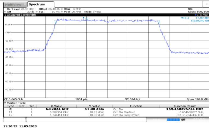
11AX160MIMO_Ant6_6665
