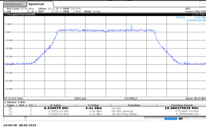
11AX20MIMO_Ant6_6515
