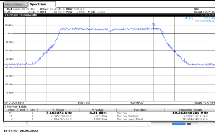
11AX20MIMO_Ant6_7095
