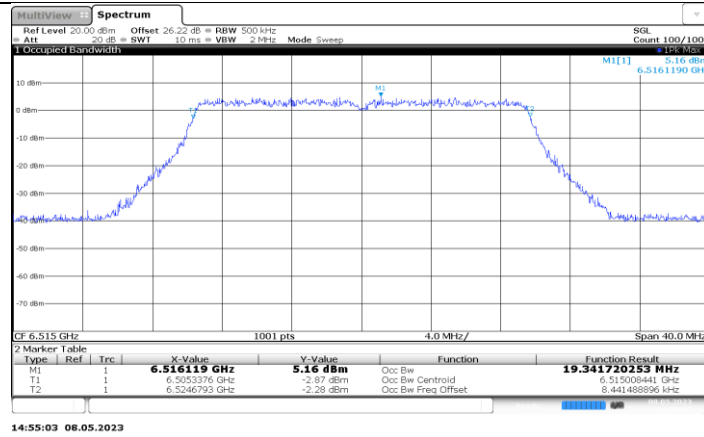
11AX20MIMO_Ant3_6515
