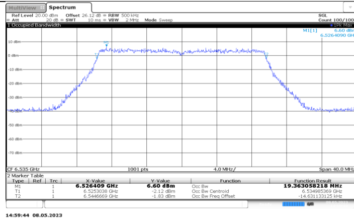
11AX20MIMO_Ant6_6535
