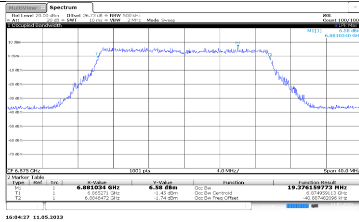
11BE20MIMO_Ant6_6875
