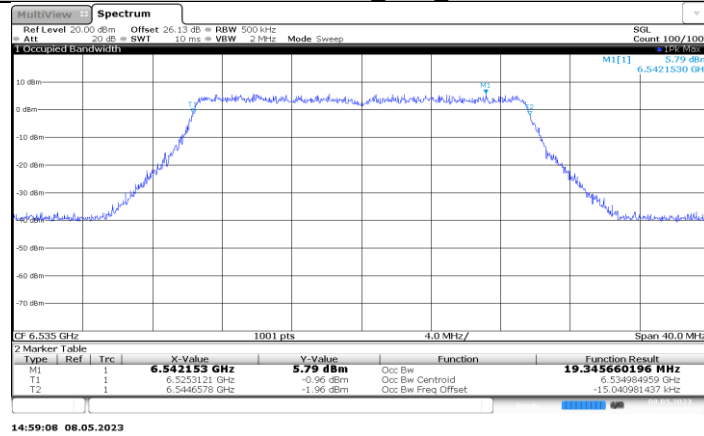
11AX20MIMO_Ant3_6535
