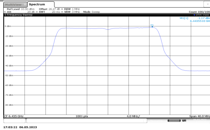
11AX20MIMO_Ant6_6435
