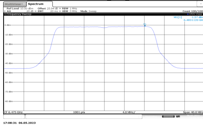
11AX20MIMO_Ant3_6475
