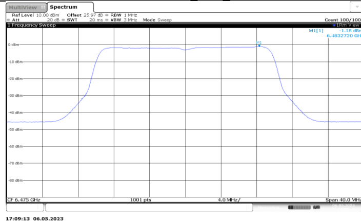
11AX20MIMO_Ant6_6475
