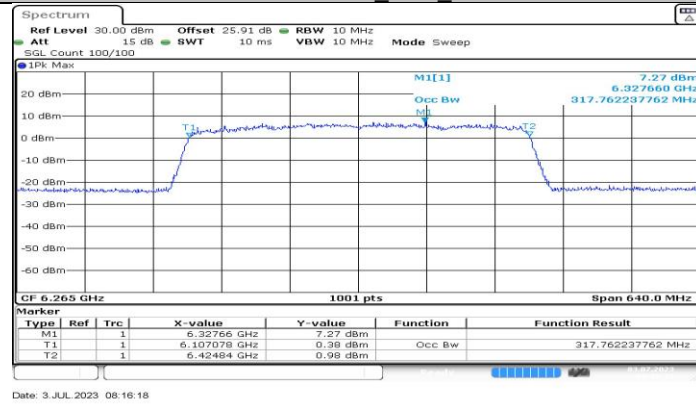
11BE320MIMO_Ant6_6265
