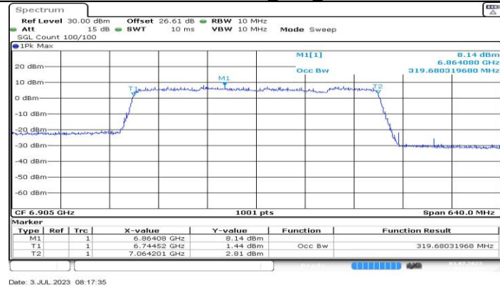
11BE320MIMO_Ant3_6905
