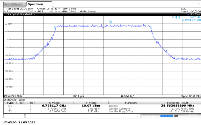
11BE40MIMO_Ant6_6725
