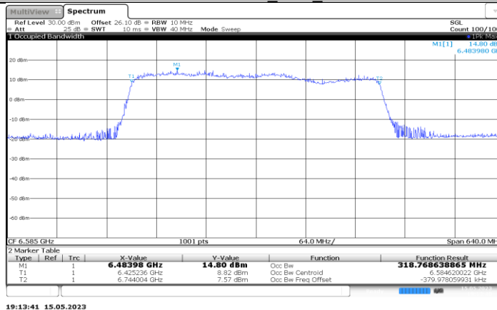
11BE320MIMO_Ant3_6585
