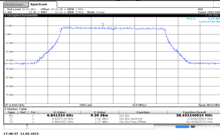
11BE40MIMO_Ant3_6845
