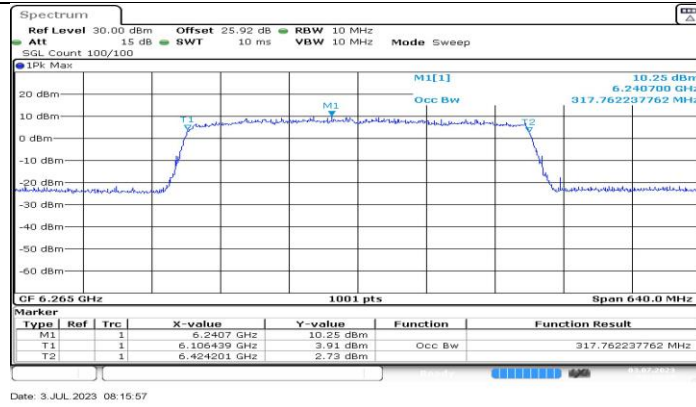
11BE320MIMO_Ant3_6265
