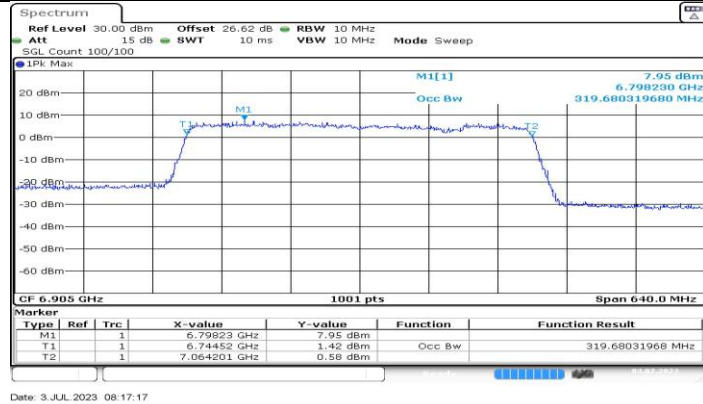
11BE320MIMO_Ant6_6905
