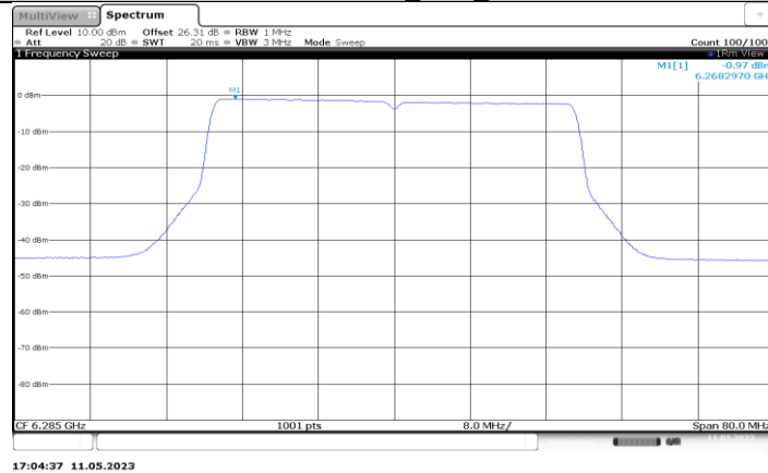
11BE40MIMO_Ant6_6285
