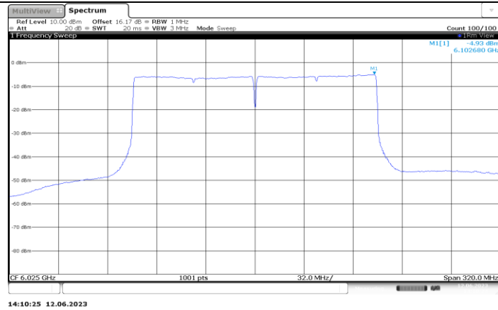
11AX160MIMO_Ant3_6025
