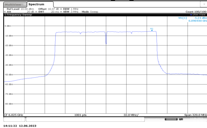
11AX160MIMO_Ant6_6025
