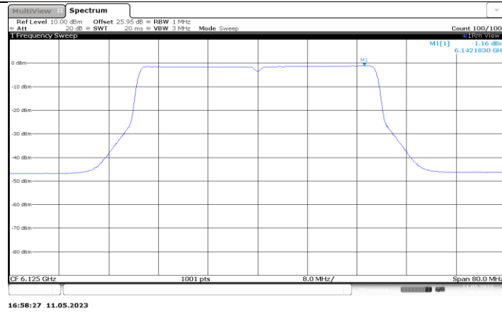
11BE40MIMO_Ant6_6125
