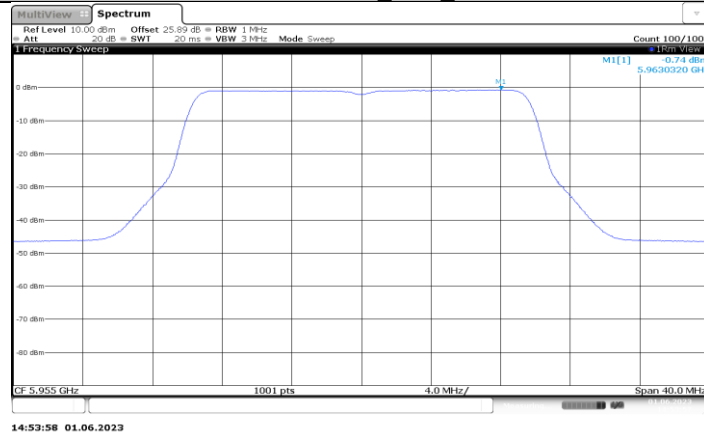
11BE20MIMO_Ant3_5955
