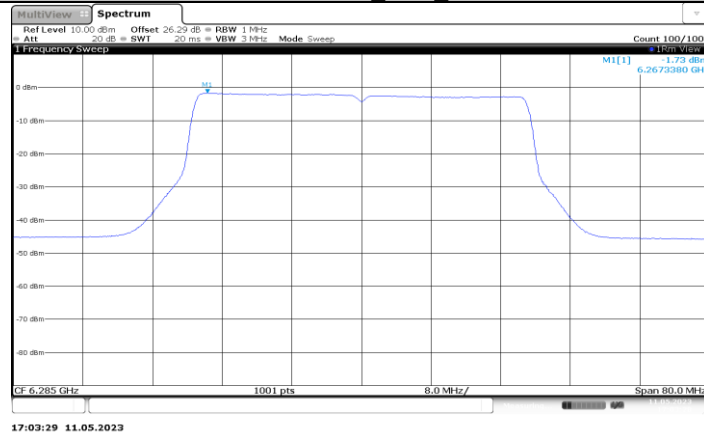
11BE40MIMO_Ant3_6285
