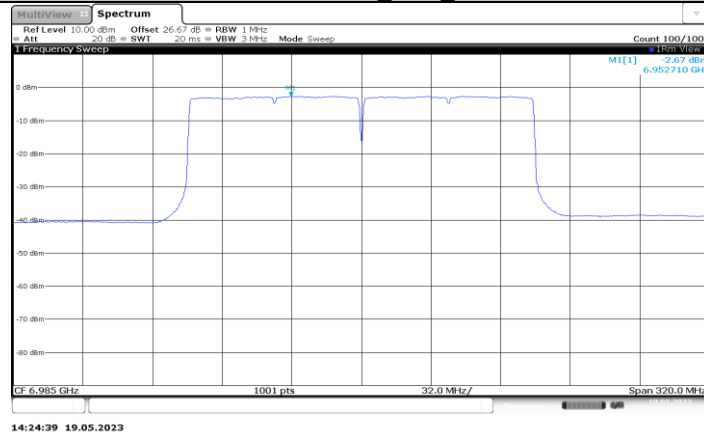
11AX160MIMO_Ant6_6985
