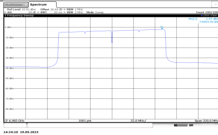
11AX160MIMO_Ant3_6985
