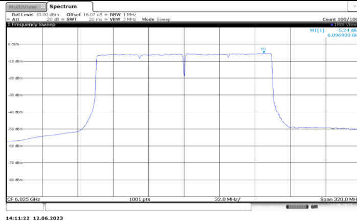
11AX160MIMO_Ant6_6025
