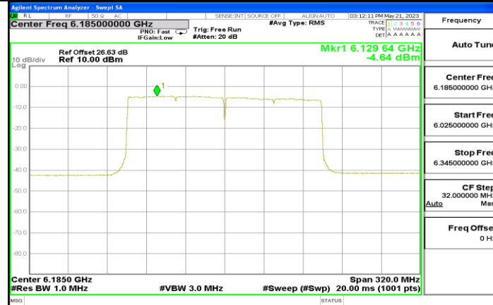
11AX160MIMO_Ant3_6185
