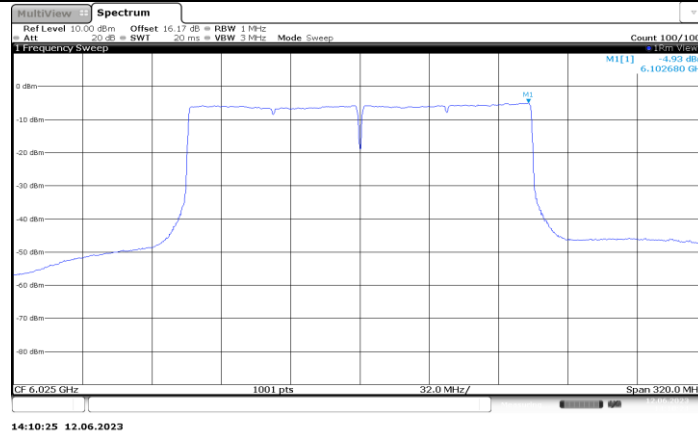
11AX160MIMO_Ant3_6025
