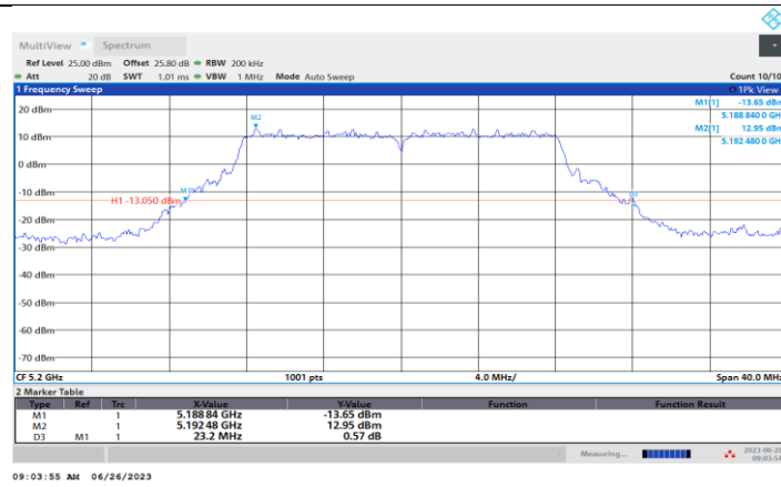
11A-CDD_Ant6_5200
