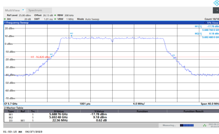
11AX20-CDD_Ant6_5700
