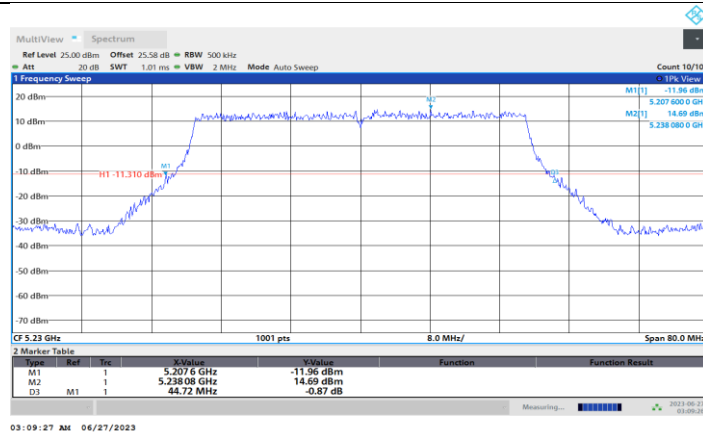
11AX40-CDD_Ant5_5230
