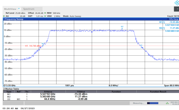
11AX40-CDD_Ant6_5550
