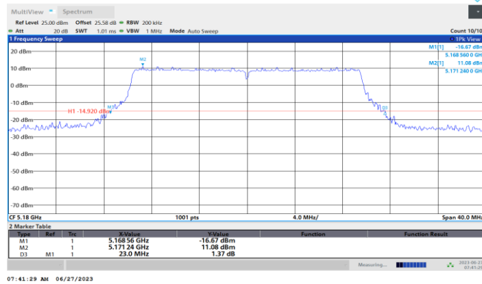
11BE20-CDD_Ant5_5180
