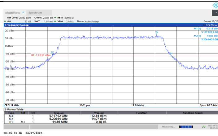
11BE40-CDD_Ant5_5190
