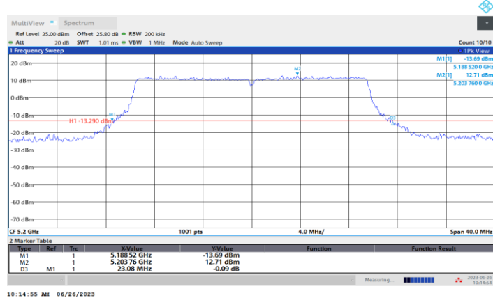
11AX20-CDD_Ant6_5200
