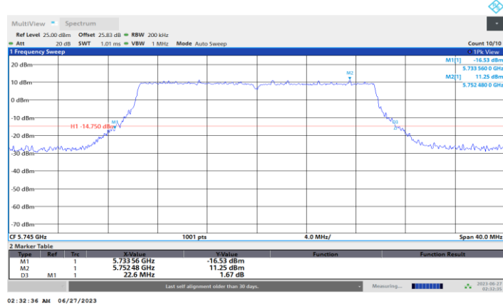
11AX20-CDD_Ant5_5745
