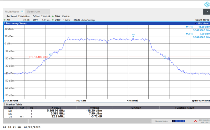
11A-CDD_Ant6_5580
