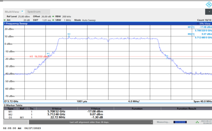
11AX20-CDD_Ant6_5720
