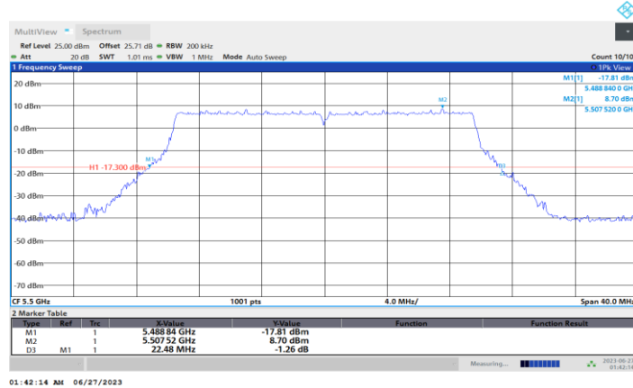
11AX20-CDD_Ant5_5500
