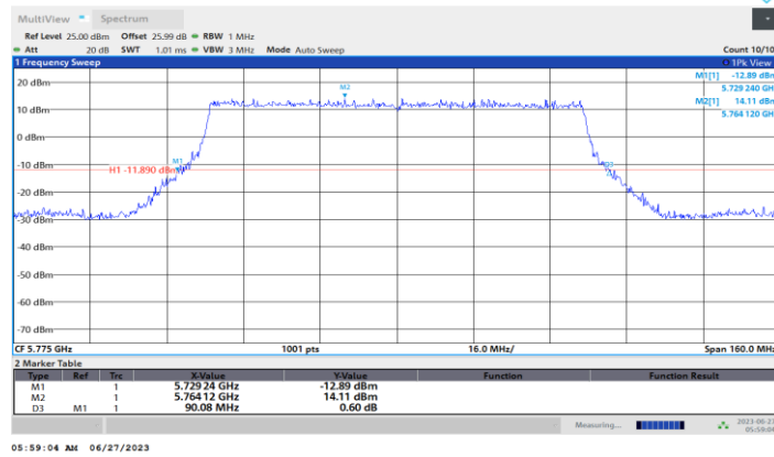
11AX80-CDD_Ant6_5775
