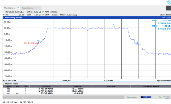
11BE20-CDD_Ant6_5745
