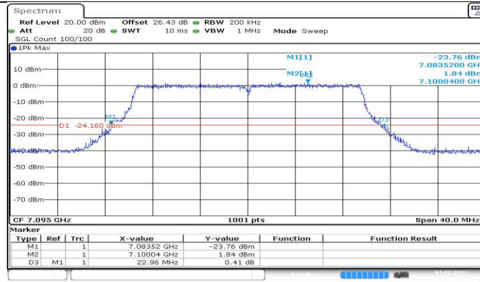
11AX20MIMO_Ant2_7095
