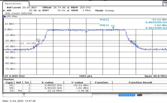
11BE20MIMO_Ant1_6895
