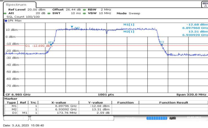
11BE160MIMO_Ant3_6985
