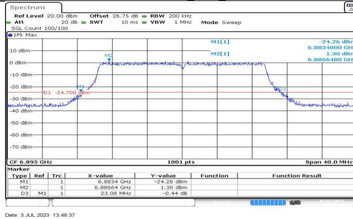
11BE20MIMO_Ant2_6895
