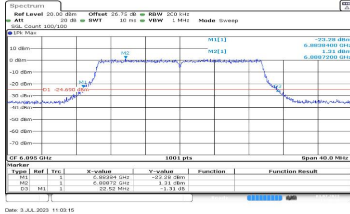
11AX20MIMO_Ant2_6895
