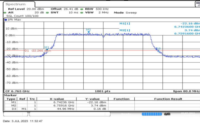
11AX40MIMO_Ant1_6765
