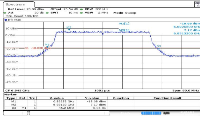
11AX40MIMO_Ant2_6845
