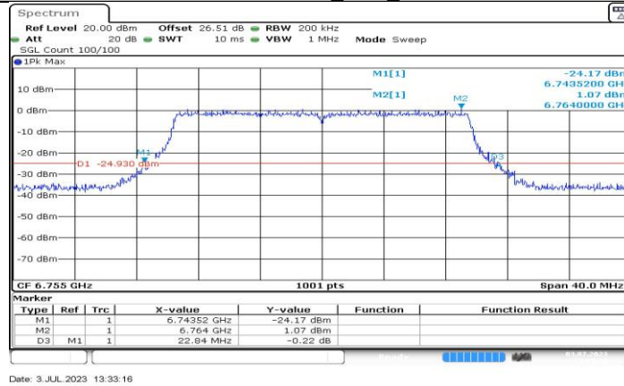
11BE20MIMO_Ant2_6755
