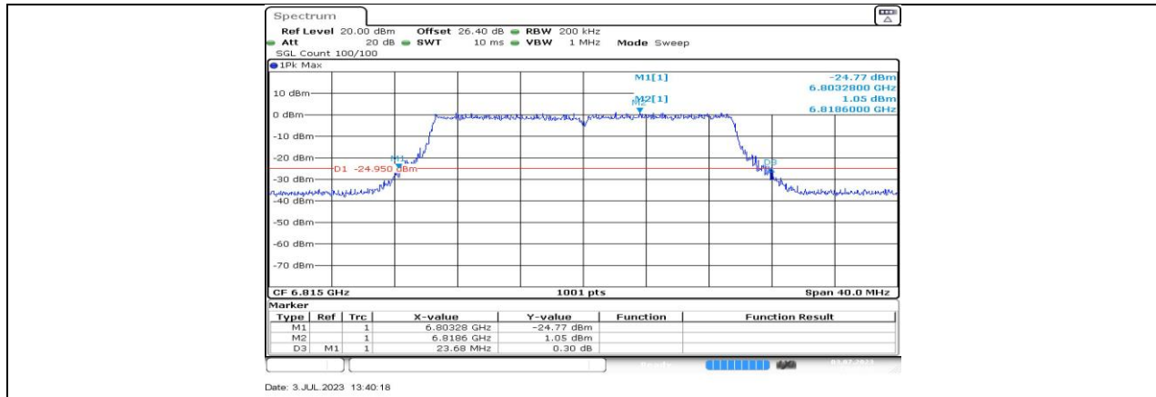
11BE20MIMO_Ant1_6815
