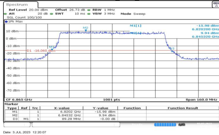
11AX80MIMO_Ant2_6865
