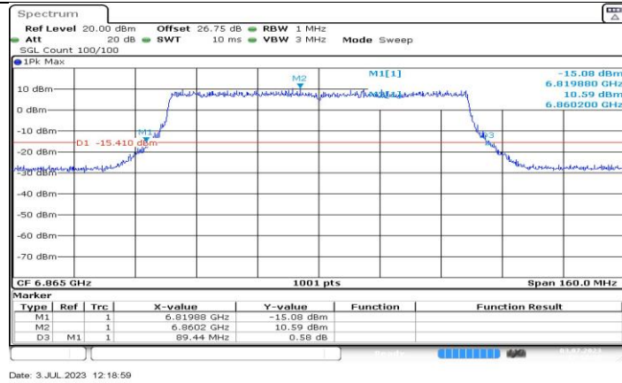
11AX80MIMO_Ant1_6865
