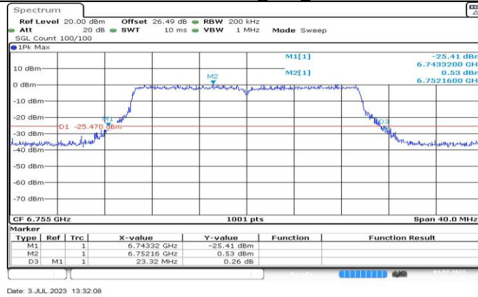
11BE20MIMO_Ant1_6755
