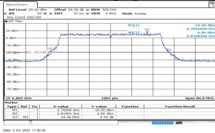
11AX40MIMO_Ant2_6805
