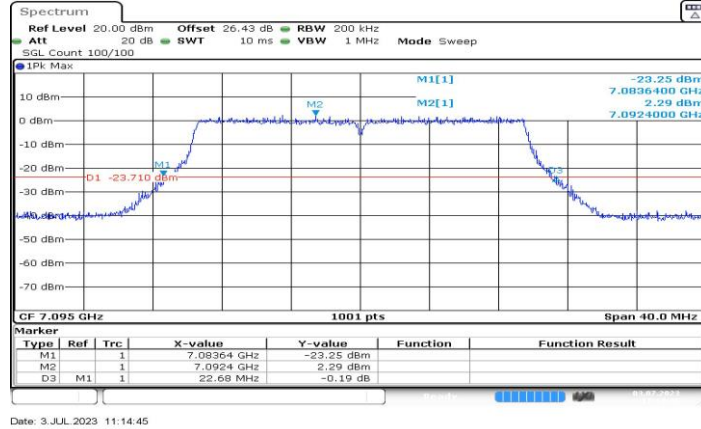
11AX20MIMO_Ant1_7095
