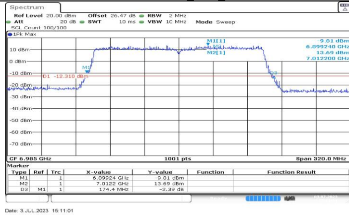
11BE160MIMO_Ant4_6985
