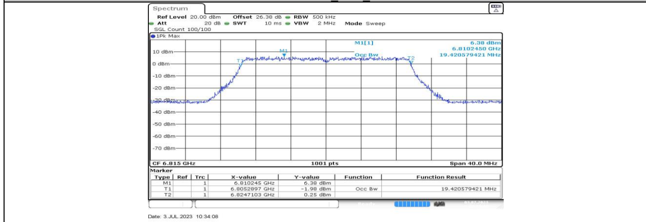
11AX20MIMO_Ant2_6815
