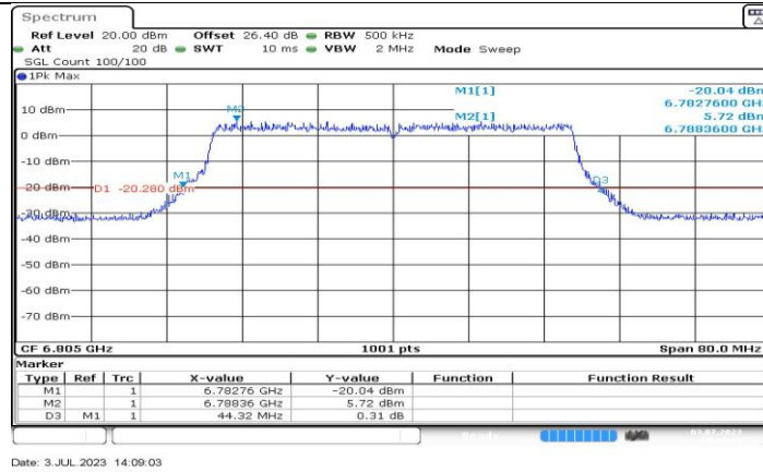
11BE40MIMO_Ant1_6805
