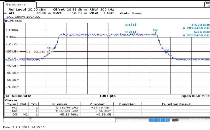
11BE40MIMO_Ant2_6805
