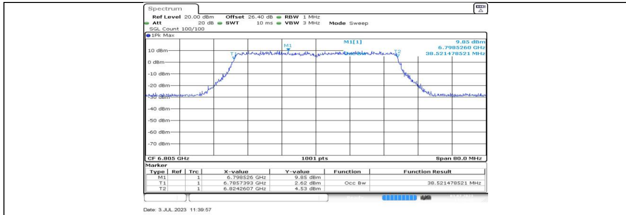
11AX40MIMO_Ant1_6805
