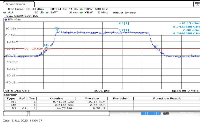
11BE40MIMO_Ant1_6765
