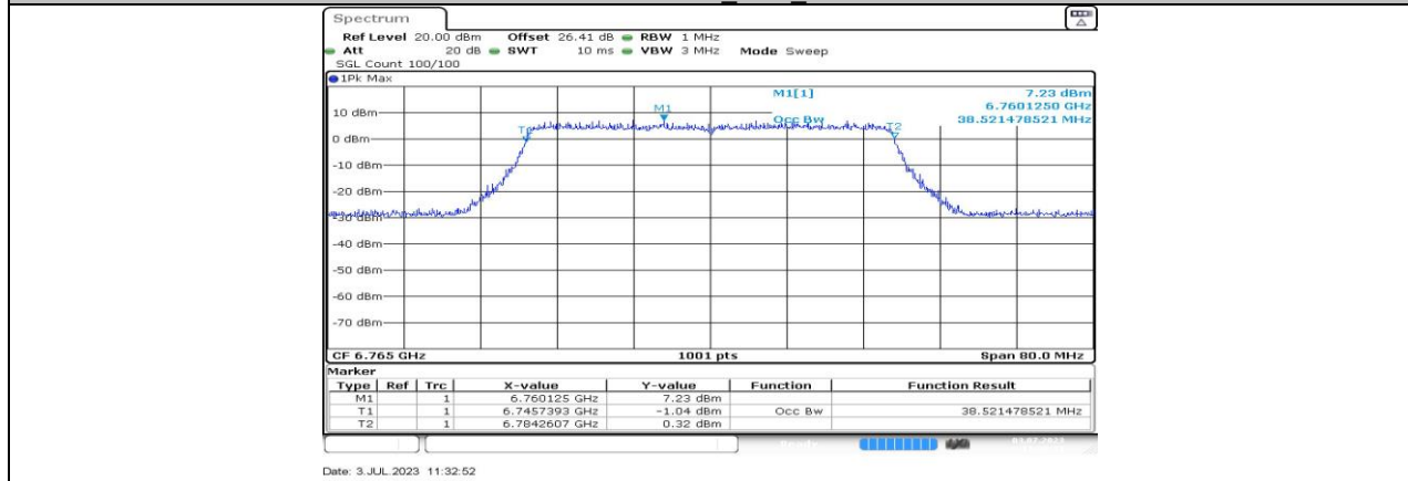
11AX40MIMO_Ant1_6765
