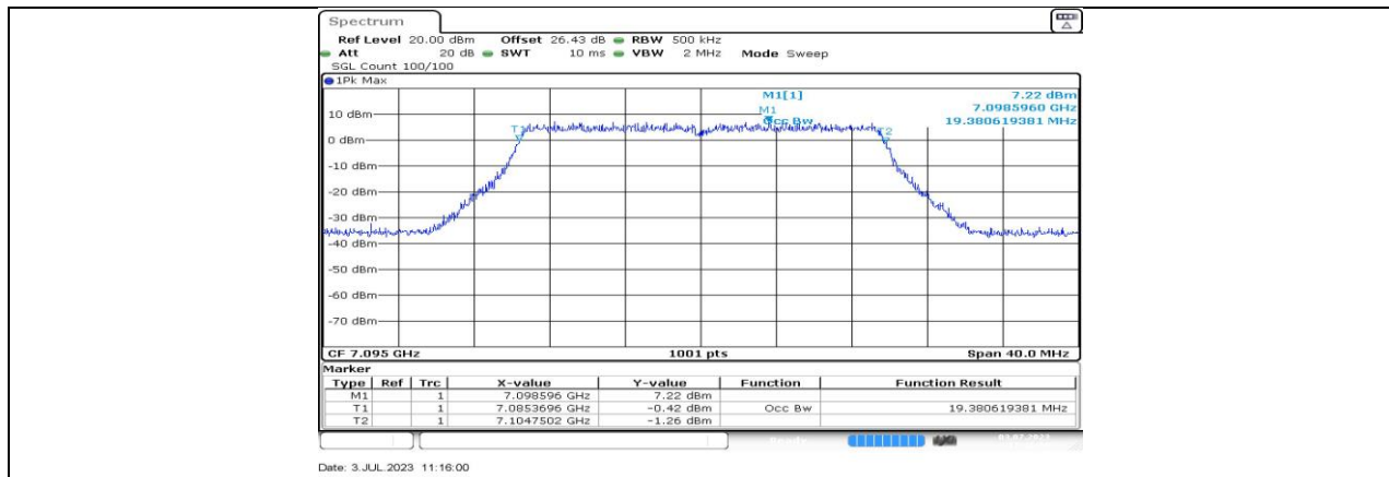
11AX20MIMO_Ant2_7095
