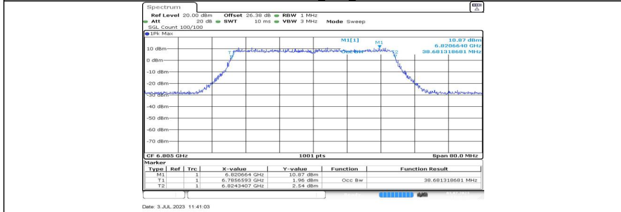
11AX40MIMO_Ant2_6805
