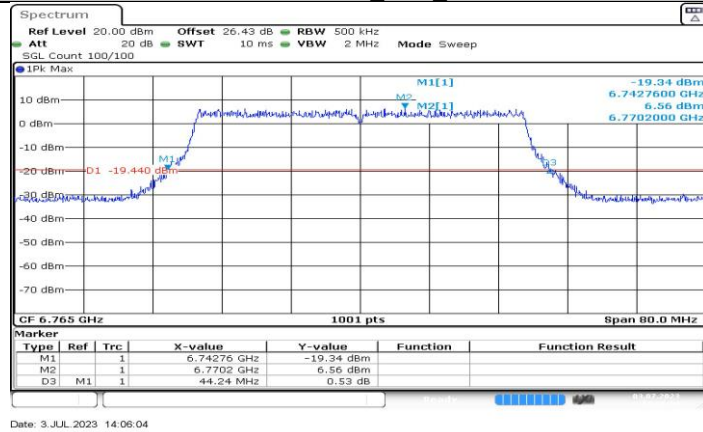
11BE40MIMO_Ant2_6765
