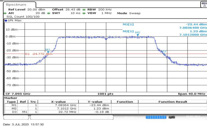
11BE20MIMO_Ant2_7095
