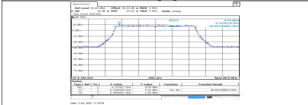
11AX40MIMO_Ant2_6765
