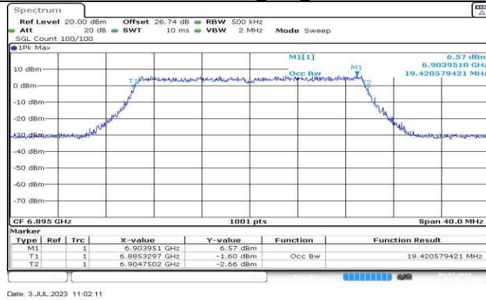
11AX20MIMO_Ant1_6895
