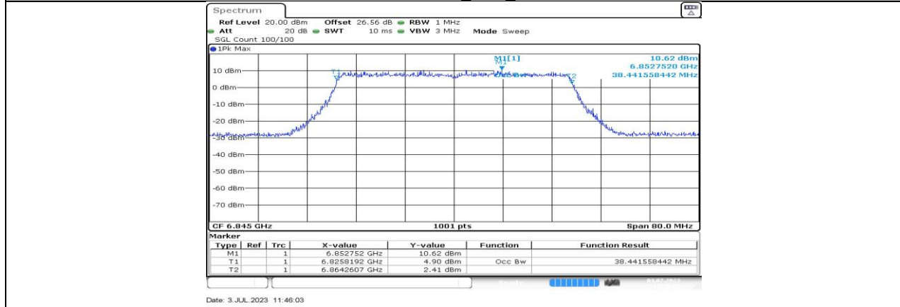
11AX40MIMO_Ant1_6845
