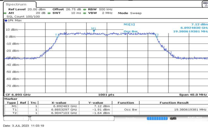
11AX20MIMO_Ant2_6895
