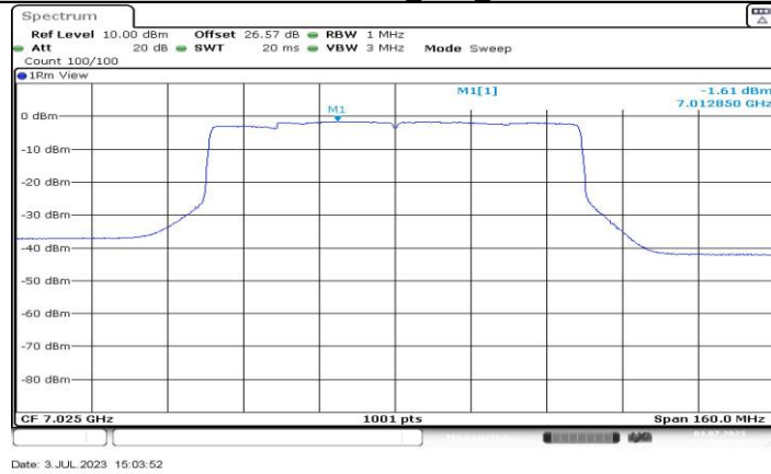
11BE80MIMO_Ant1_7025
