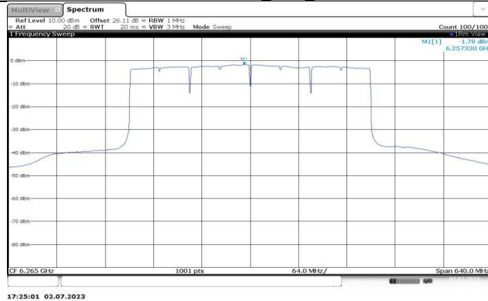
11BE320MIMO_Ant3_6265
