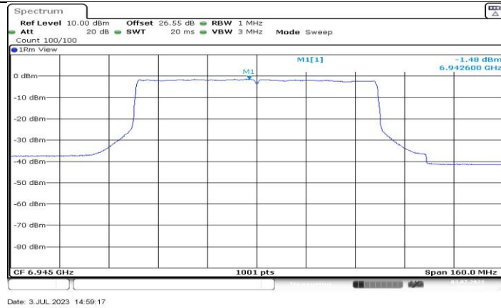
11BE80MIMO_Ant2_6945
