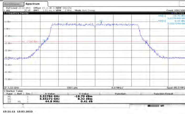
11AX40MIMO_Ant3_5550
