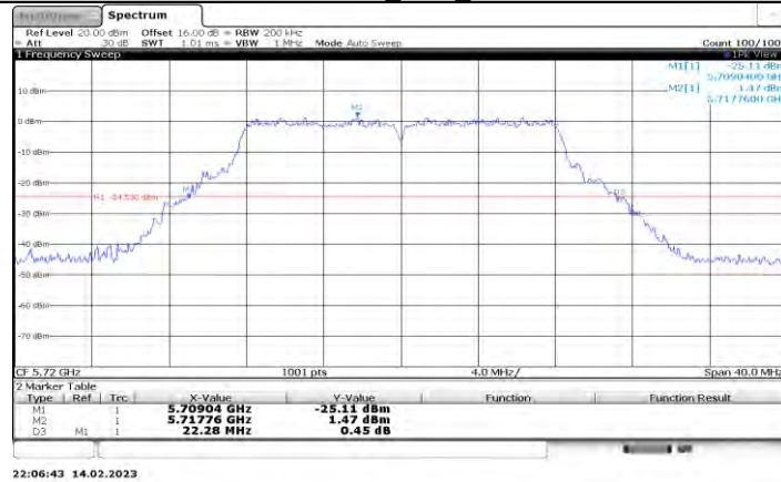
11A-CDD_Ant2_5720
