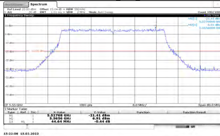
11AX40MIMO_Ant4_5550
