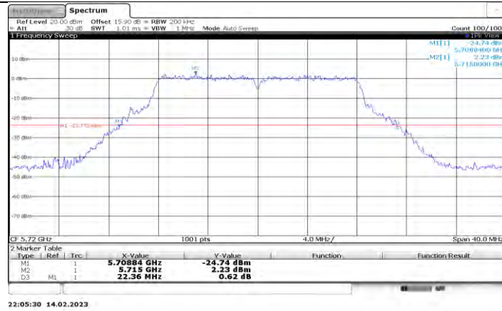
11A-CDD_Ant1_5720
