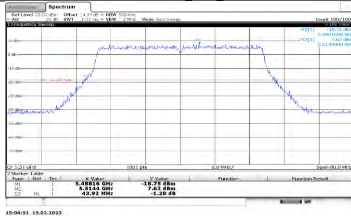
11AX40MIMO_Ant3_5510
