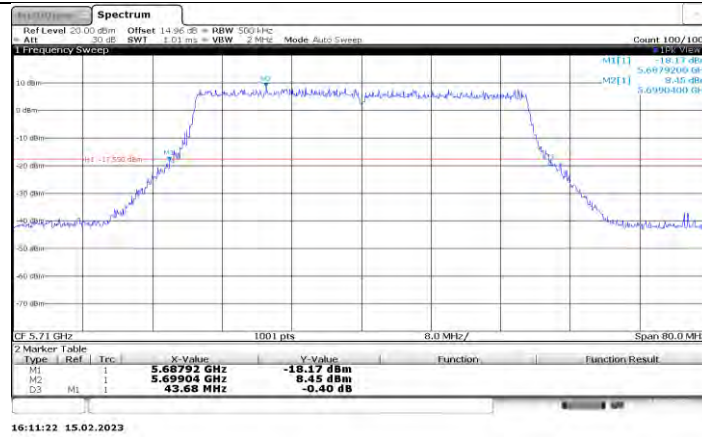
11AX40MIMO_Ant4_5710
