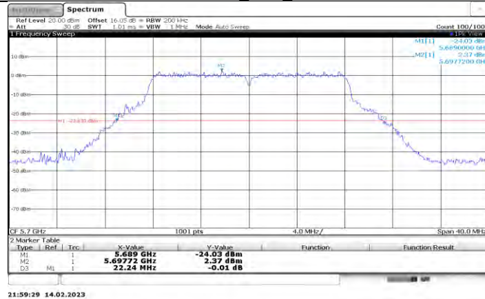
11A-CDD_Ant1_5700
