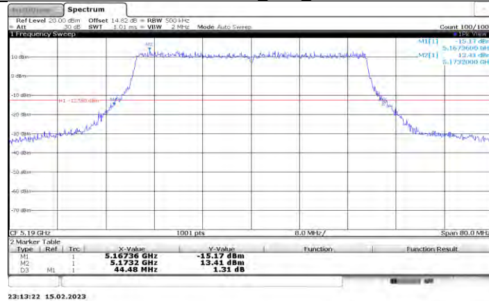
11BE40MIMO_Ant3_5190
