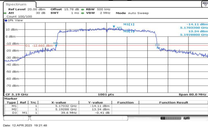
11AX40-CDD_Ant2_5190
