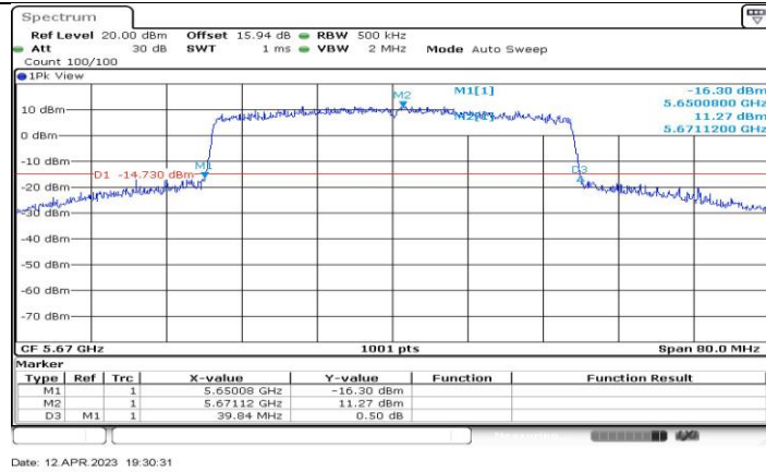
11AX40-CDD_Ant1_5670
