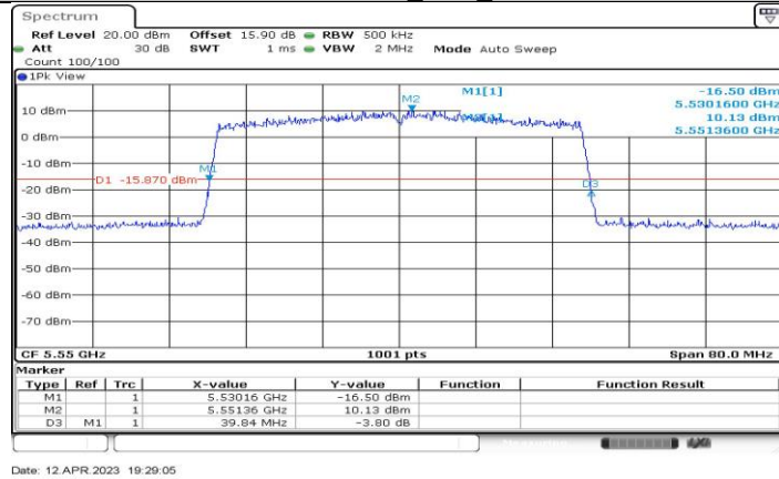
11AX40-CDD_Ant1_5550
