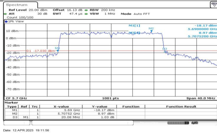
11AX20-CDD_Ant2_5700
