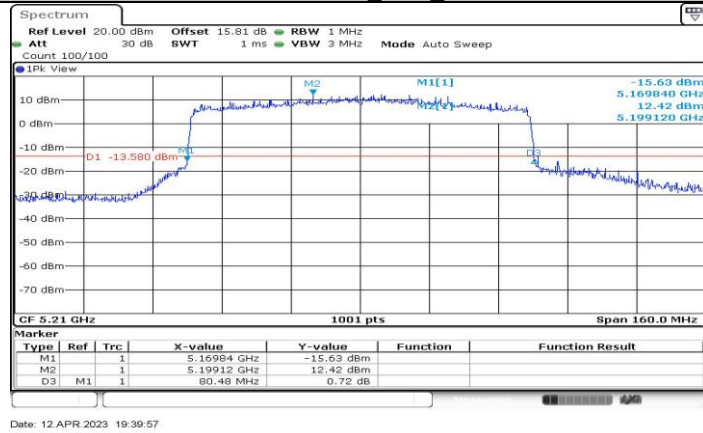
11AX80-CDD_Ant2_5210
