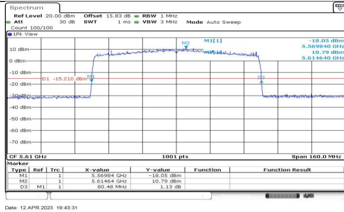
11AX80-CDD_Ant1_5610
