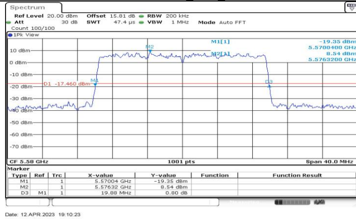
11AX20-CDD_Ant1_5580
