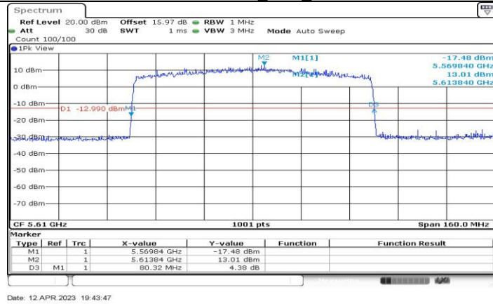
11AX80-CDD_Ant2_5610
