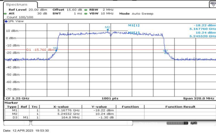
11AX160-CDD_Ant1_5250
