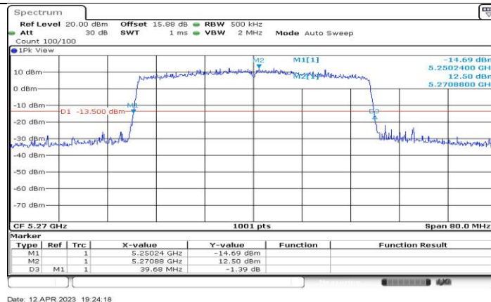
11AX40-CDD_Ant2_5270
