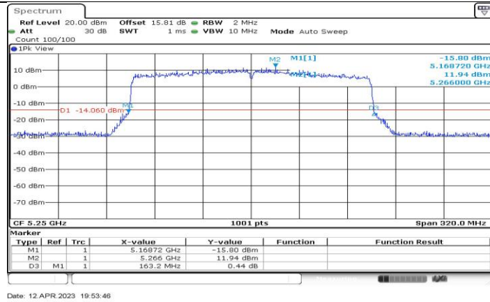
11AX160-CDD_Ant2_5250
