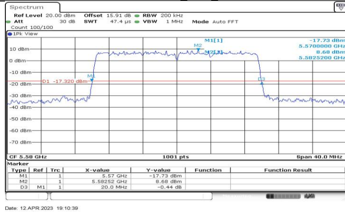
11AX20-CDD_Ant2_5580
