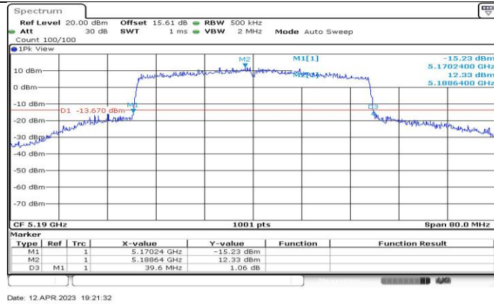
11AX40-CDD_Ant1_5190
