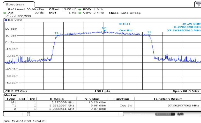
11AX40-CDD_Ant2_5270
