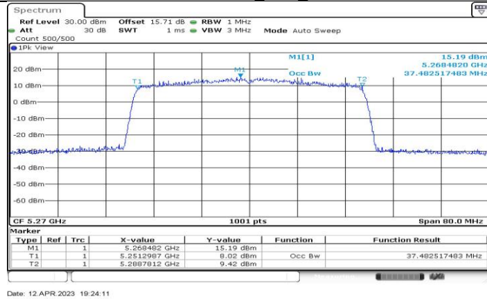
11AX40-CDD_Ant1_5270
