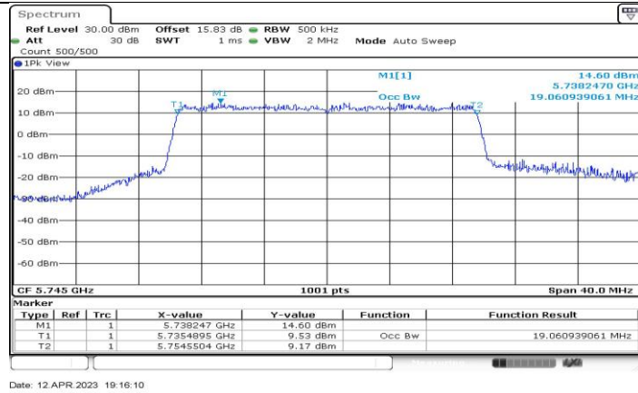
11AX20-CDD_Ant1_5745
