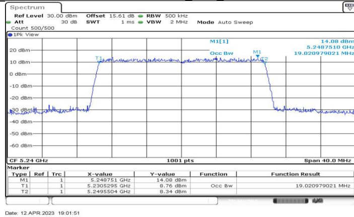
11AX20-CDD_Ant1_5240
