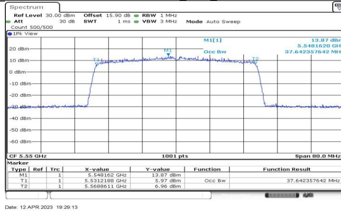
11AX40-CDD_Ant1_5550
