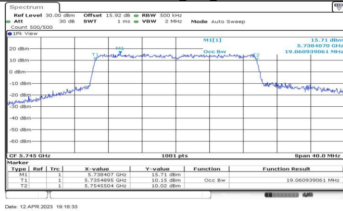
11AX20-CDD_Ant2_5745
