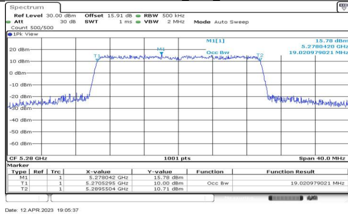
11AX20-CDD_Ant2_5280
