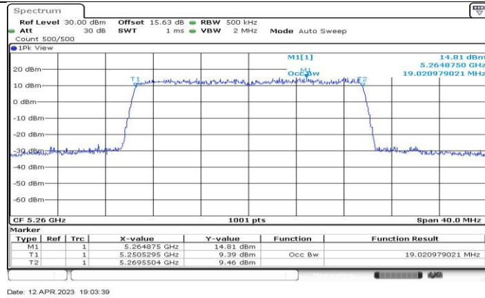
11AX20-CDD_Ant1_5260
