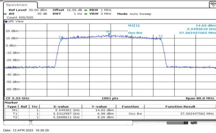
11AX40-CDD_Ant2_5550
