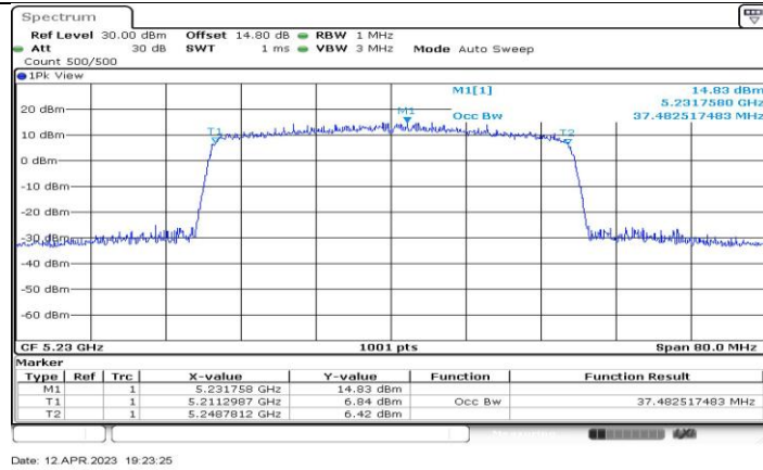
11AX40-CDD_Ant3_5230
