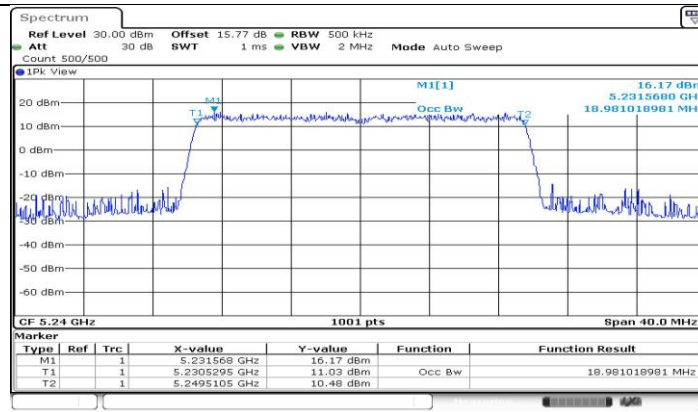
11AX20-CDD_Ant2_5240
