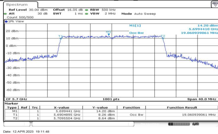
11AX20-CDD_Ant1_5700
