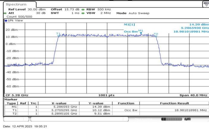
11AX20-CDD_Ant1_5280
