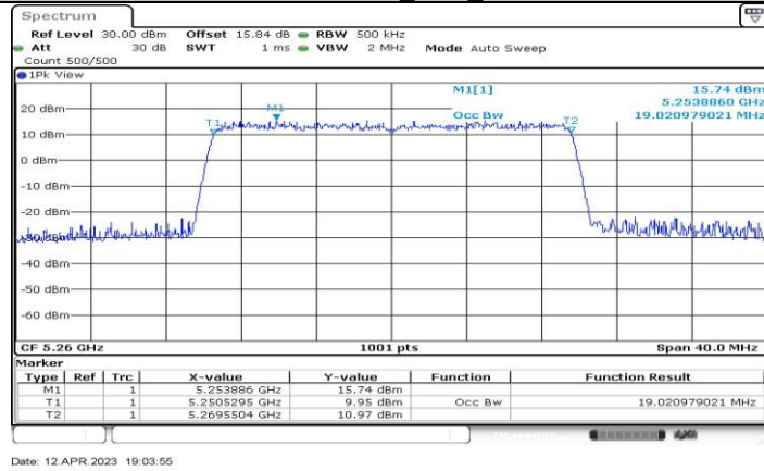
11AX20-CDD_Ant2_5260
