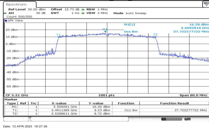
11AX40-CDD_Ant1_5510
