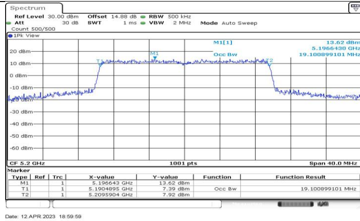
11AX20-CDD_Ant3_5200
