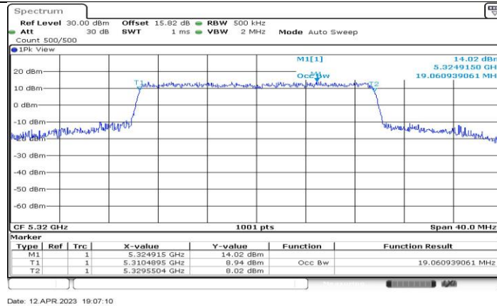
11AX20-CDD_Ant2_5320
