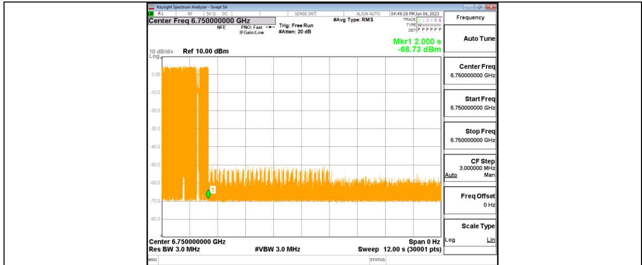
11BE320MIMO Ant1 6905 Low 6750 1
