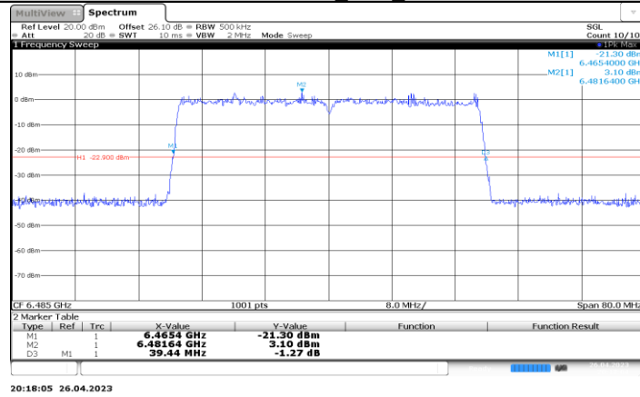
11BE40-CDD_Ant3_6485
