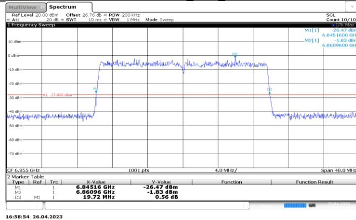
11BE20-CDD_Ant3_6855
