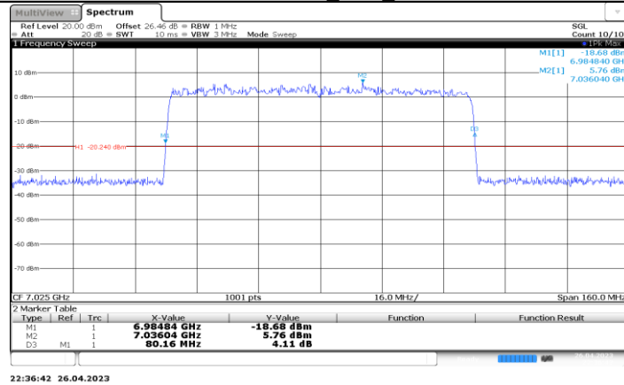
11BE80-CDD_Ant3_7025
