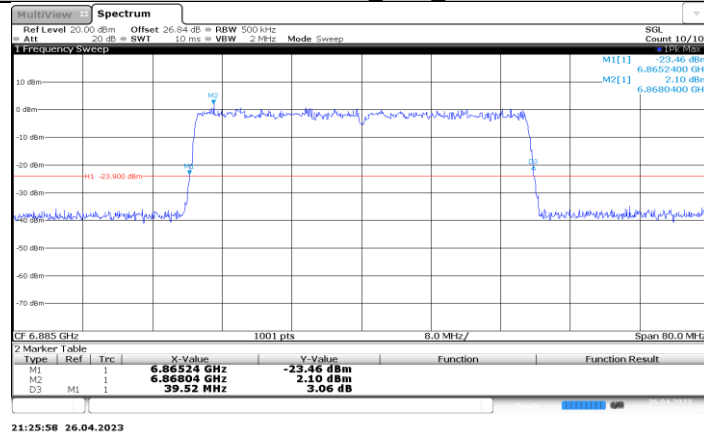
11BE40-CDD_Ant3_6885
