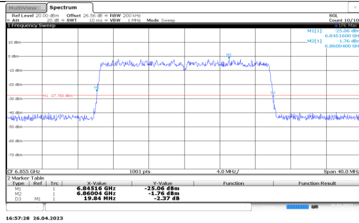
11BE20-CDD_Ant1_6855
