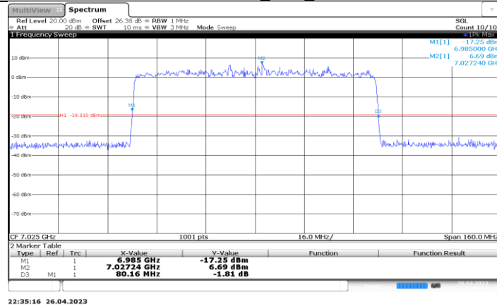
11BE80-CDD_Ant1_7025
