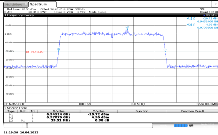
11BE40-CDD_Ant2_6965
