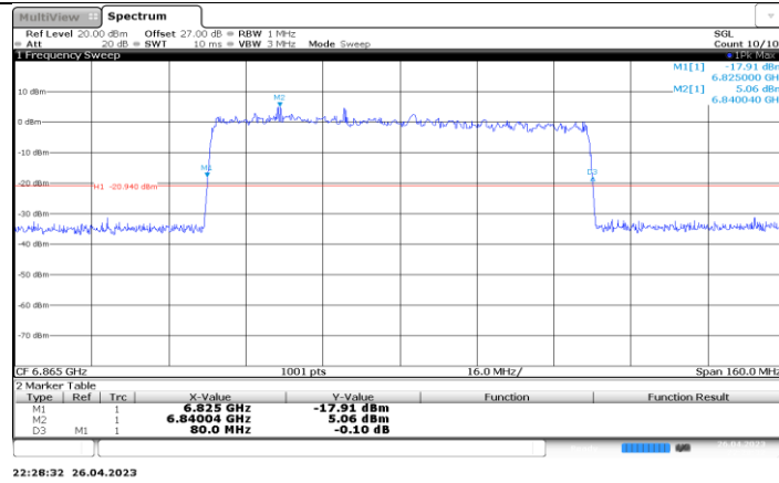
11BE80-CDD_Ant4_6865
