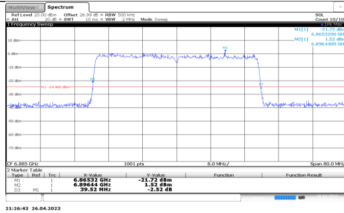
11BE40-CDD_Ant4_6885
