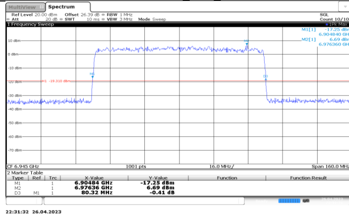
11BE80-CDD_Ant2_6945
