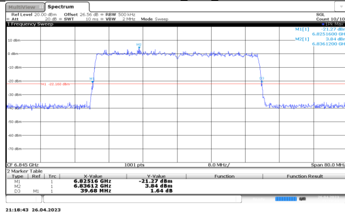
11BE40-CDD_Ant1_6845
