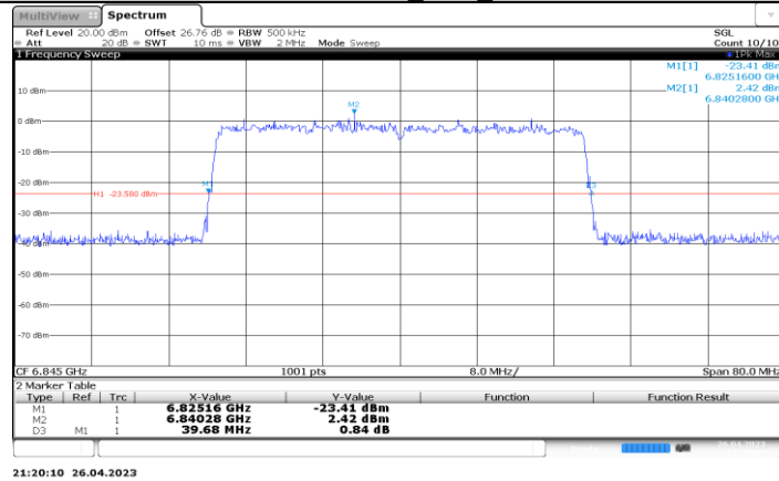
11BE40-CDD_Ant3_6845
