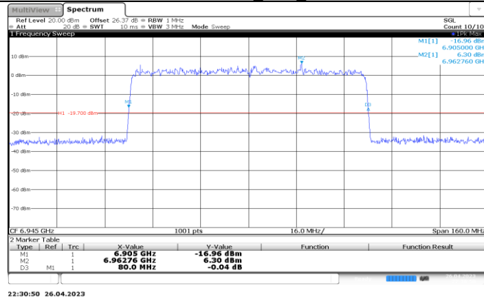
11BE80-CDD_Ant1_6945
