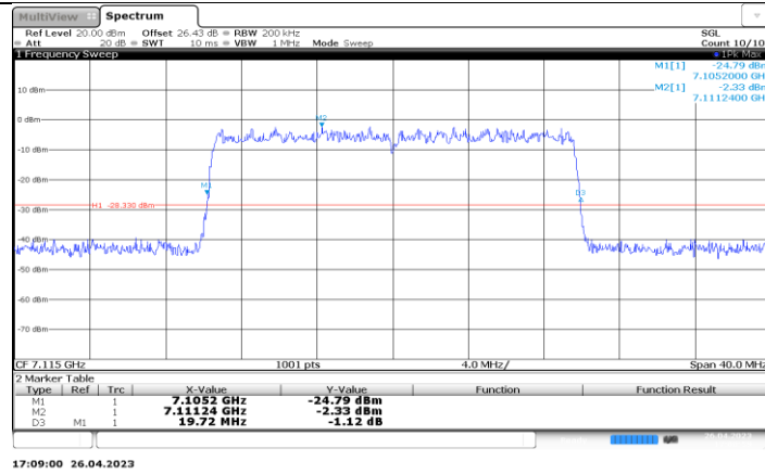
11BE20-CDD_Ant1_7115
