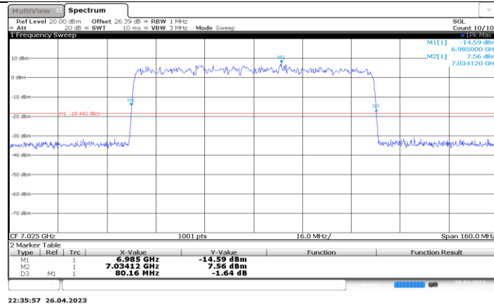
11BE80-CDD_Ant2_7025
