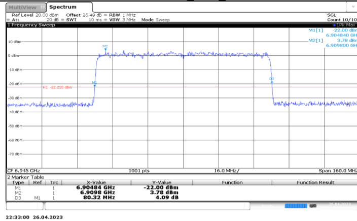
11BE80-CDD_Ant4_6945
