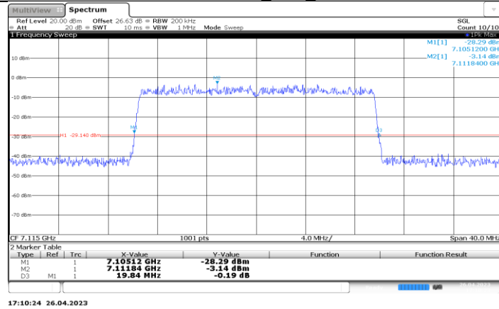
11BE20-CDD_Ant3_7115
