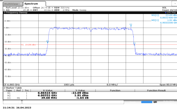
11BE40-CDD_Ant1_6885
