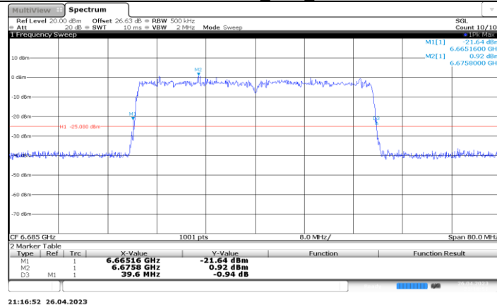
11BE40-CDD_Ant4_6685
