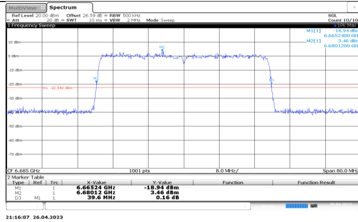
11BE40-CDD_Ant3_6685
