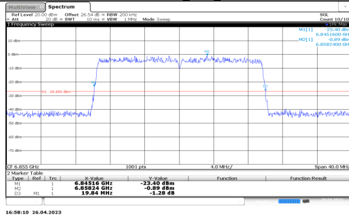
11BE20-CDD_Ant2_6855
