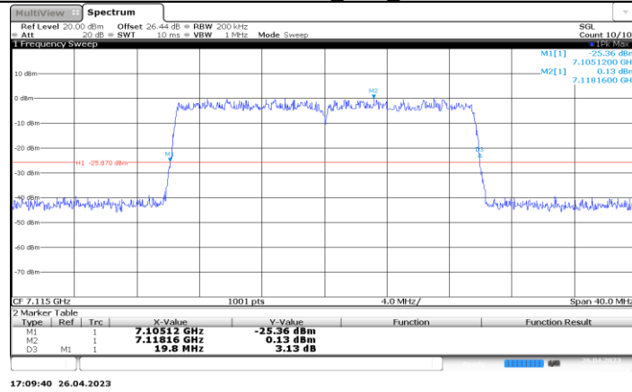
11BE20-CDD_Ant2_7115
