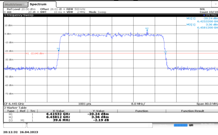
11BE40-CDD_Ant1_6445
