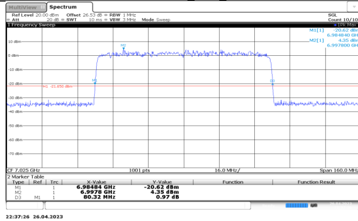
11BE80-CDD_Ant4_7025
