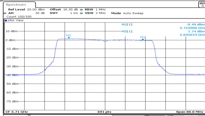
11BE40MIMO_Ant2_5710_UNII-2C
