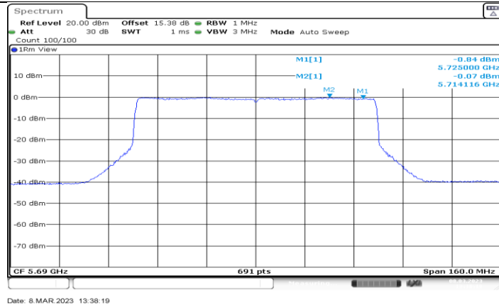
11AX80MIMO_Ant3_5690_UNII-2C
