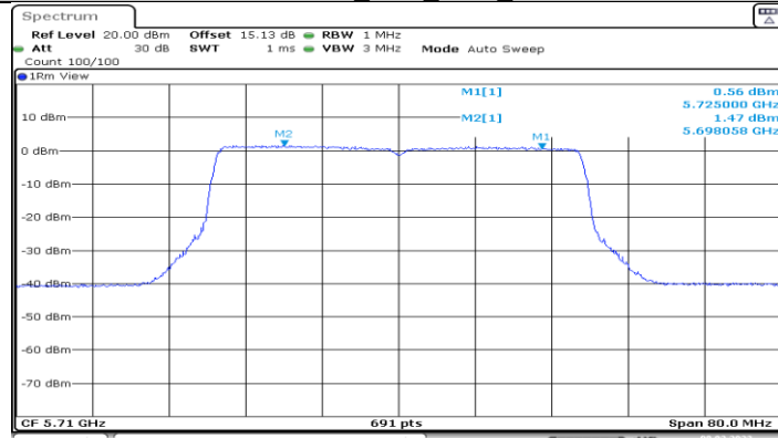
11BE40MIMO_Ant3_5710_UNII-2C
