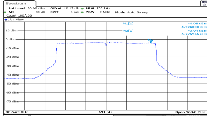
11AX80MIMO_Ant3_5690_UNII-3
