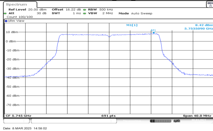
11BE20MIMO_Ant2_5745
