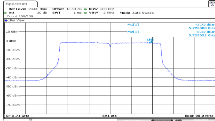
11AX40MIMO_Ant3_5710_UNII-3
