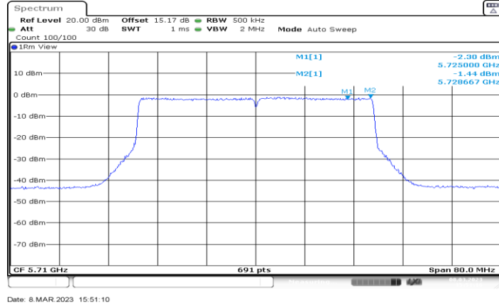
11BE40MIMO_Ant3_5710_UNII-3
