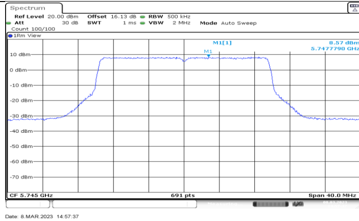
11BE20MIMO_Ant1_5745
