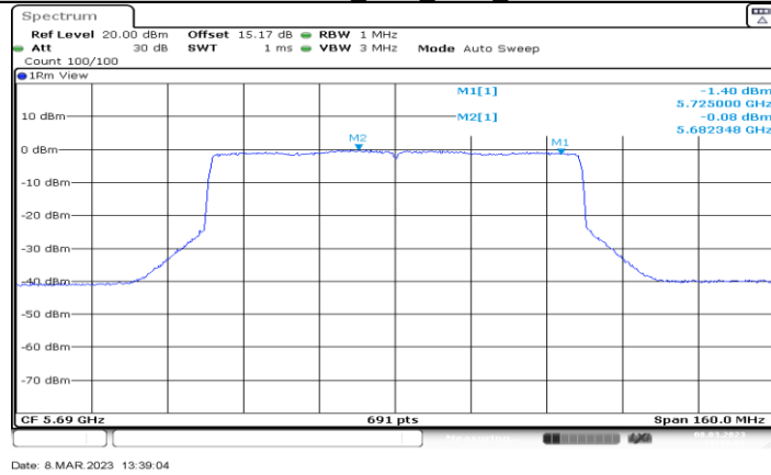
11AX80MIMO_Ant4_5690_UNII-2C
