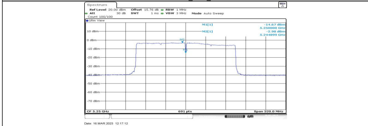
11AX160MIMO_Ant1_5250_UNII-1
