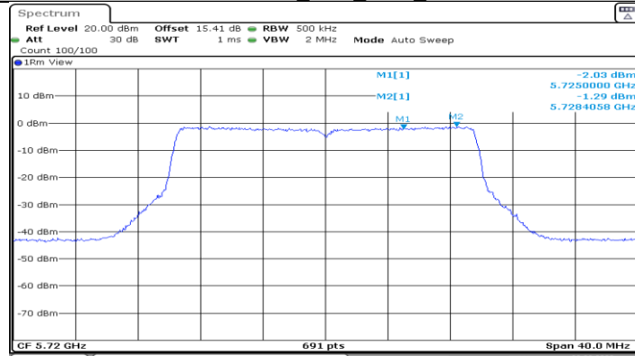
11BE20MIMO_Ant3_5720_UNII-3
