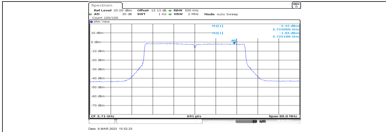
11BE40MIMO_Ant4_5710_UNII-3
