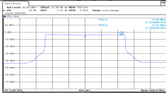
11AX80MIMO_Ant2_5690_UNII-3
