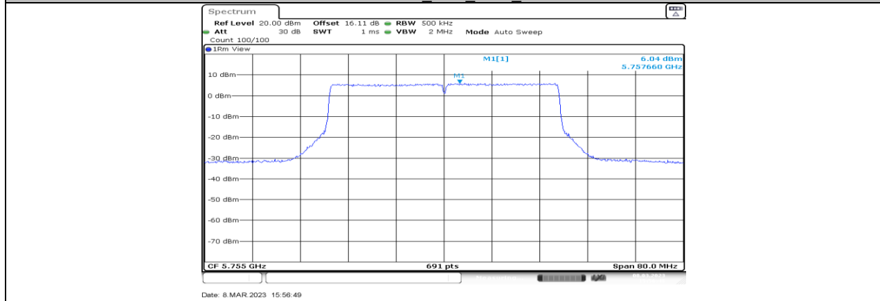
11BE40MIMO_Ant1_5755
