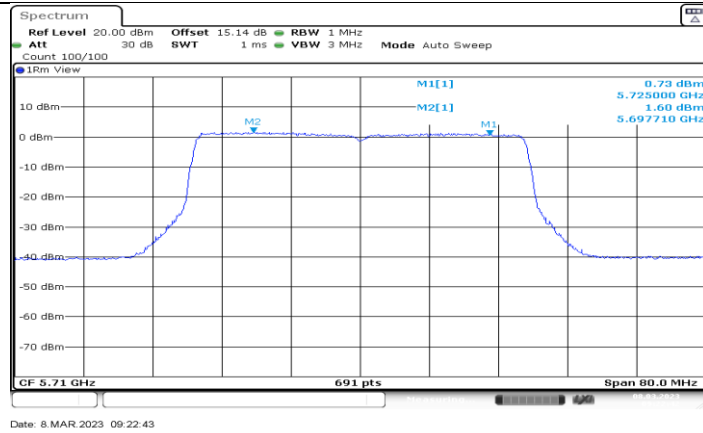
11AX40MIMO Ant4 5710 UNII-2C
