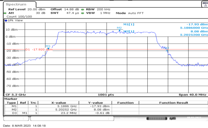
11BE20MIMO_Ant3_5200
