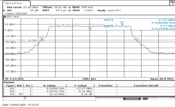
11BE20MIMO_Ant1_5240
