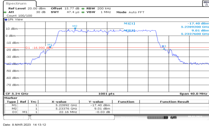
11BE20MIMO_Ant2_5240
