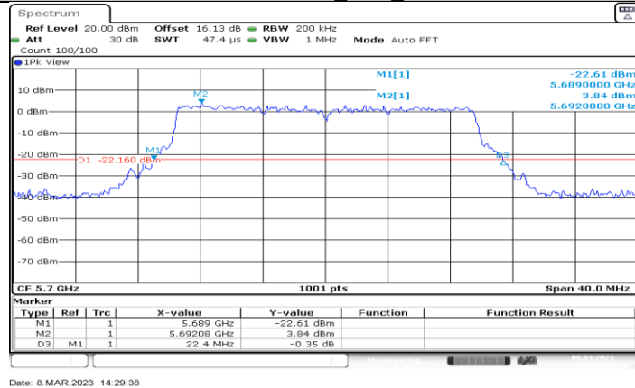
11BE20MIMO_Ant2_5700
