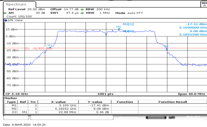
11BE20MIMO_Ant4_5180
