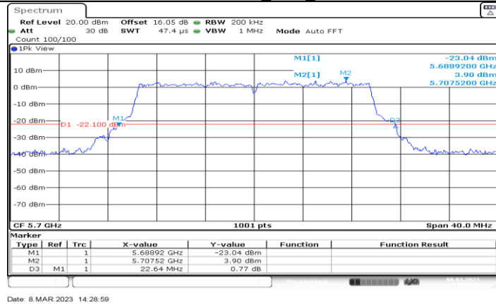
11BE20MIMO_Ant1_5700
