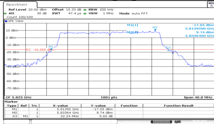
11BE20MIMO_Ant2_5825
