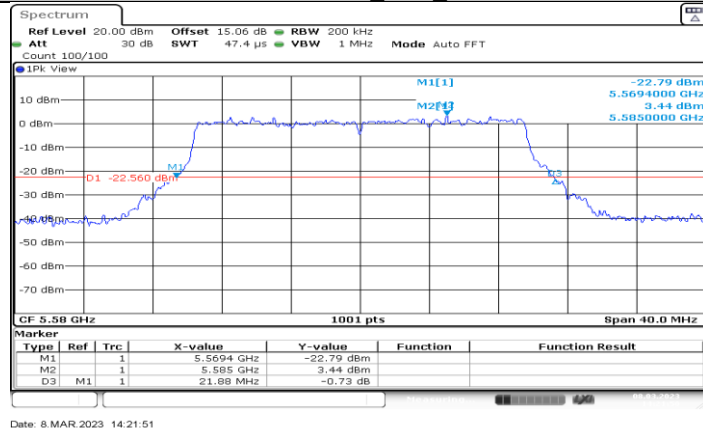
11BE20MIMO_Ant3_5580
