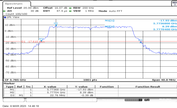
11BE20MIMO_Ant2_5785
