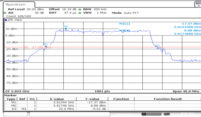
11BE20MIMO_Ant2_5825
