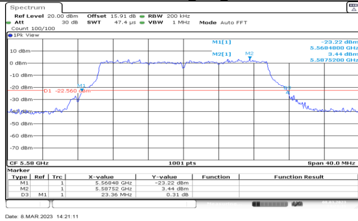
11BE20MIMO_Ant2_5580
