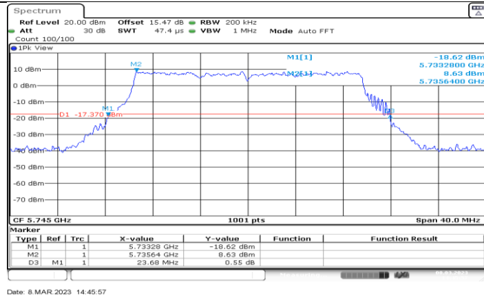
11BE20MIMO_Ant4_5745
