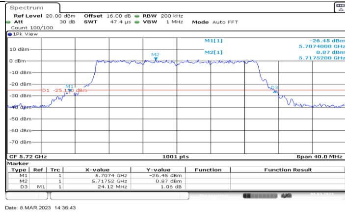
11BE20MIMO_Ant2_5720
