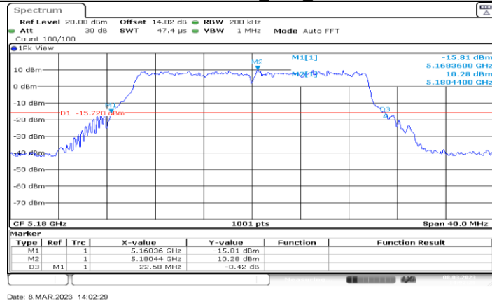
11BE20MIMO_Ant3_5180
