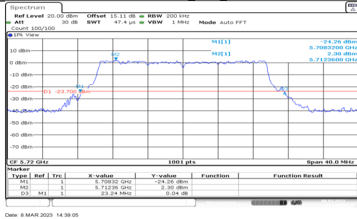
11BE20MIMO_Ant4_5720
