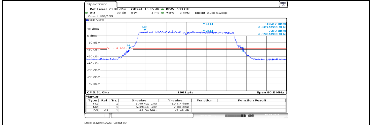
11AX40MIMO_Ant2_5510
