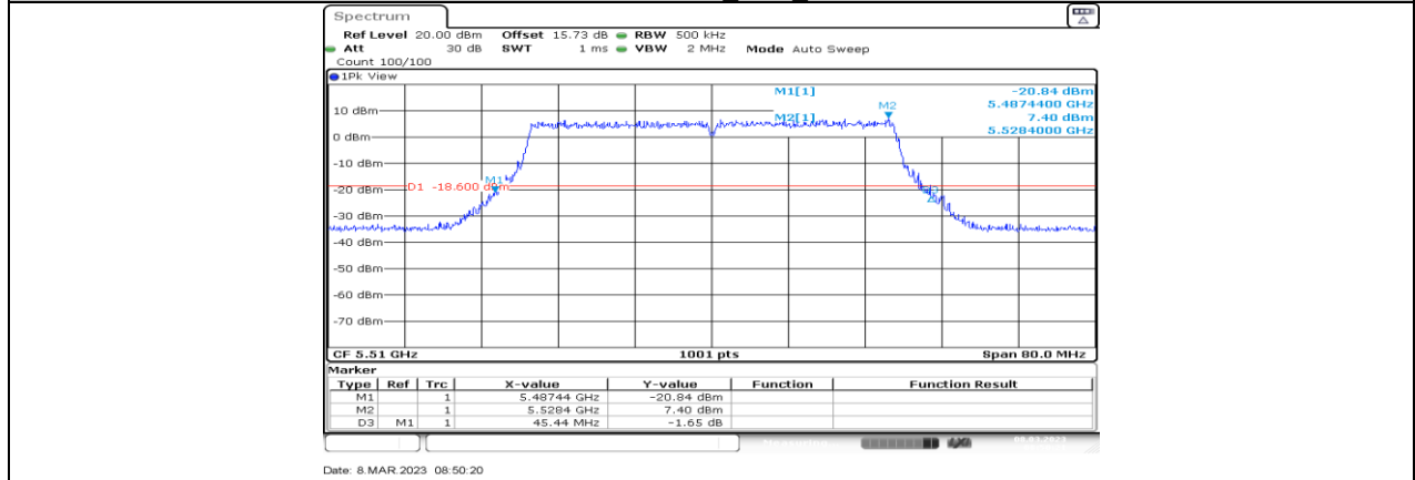
11AX40MIMO_Ant1_5510
