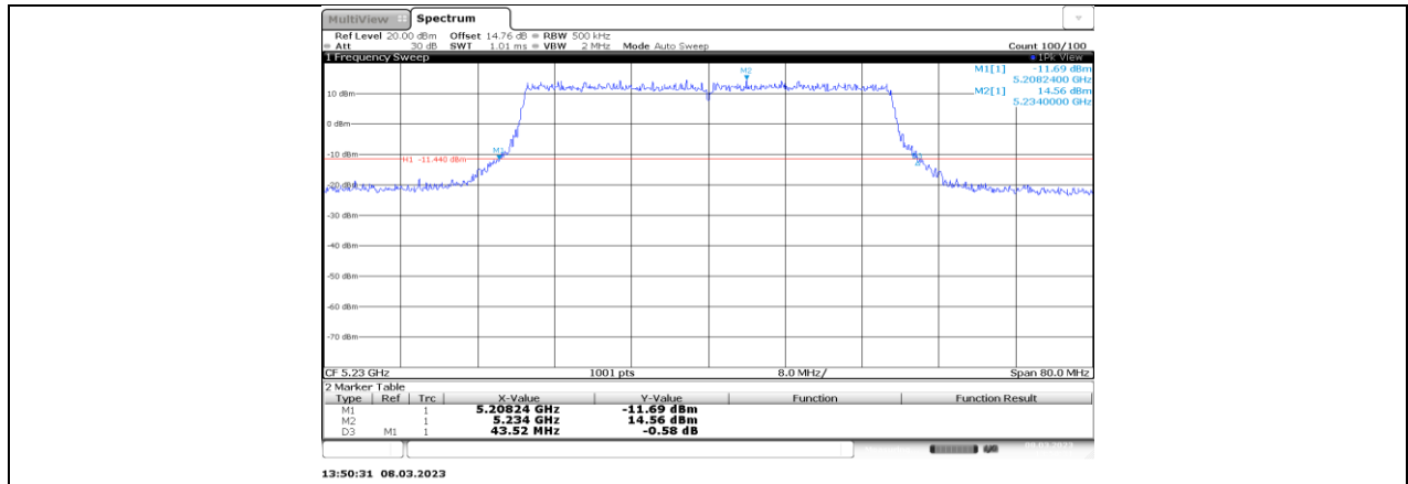
11AX40MIMO_Ant4_5230
