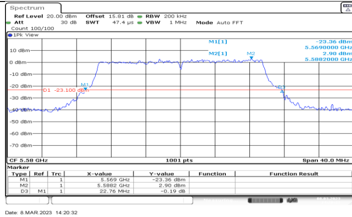
11BE20MIMO_Ant1_5580
