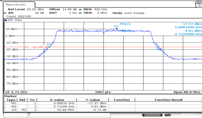
11AX40MIMO_Ant3_5710
