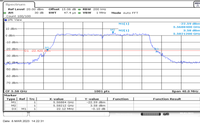
11BE20MIMO_Ant4_5580
