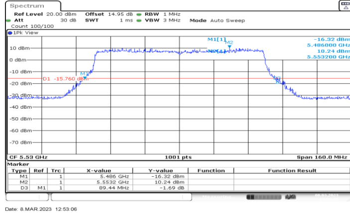
11AX80MIMO_Ant4_5530
