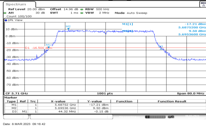
11AX40MIMO_Ant4_5710
