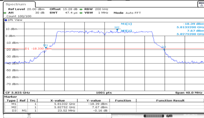
11BE20MIMO_Ant3_5825
