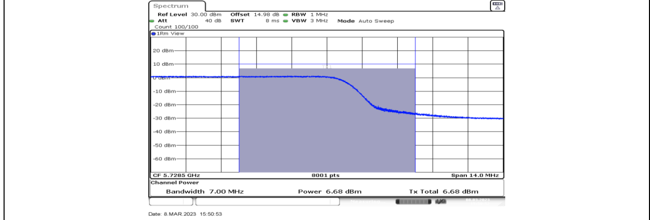
11BE40MIMO_Ant3_5710_UNII-3
