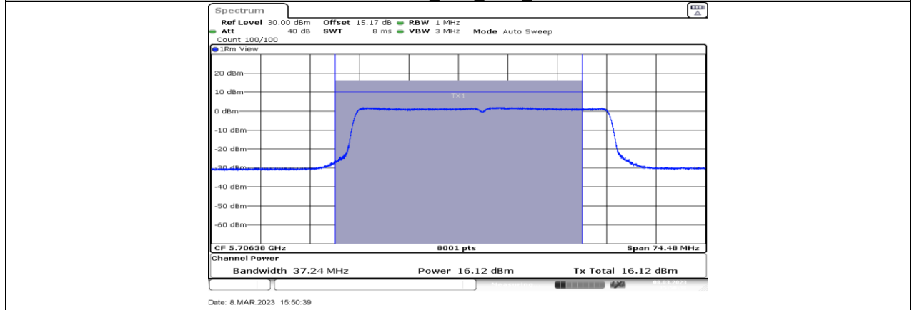
11BE40MIMO_Ant3_5710_UNII-2C
