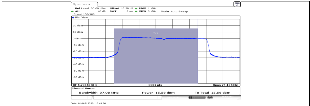
11BE40MIMO_Ant2_5710_UNII-2C
