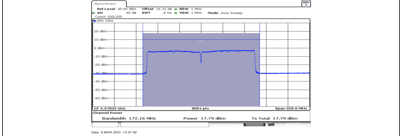
11AX160MIMO_Ant3_5570
