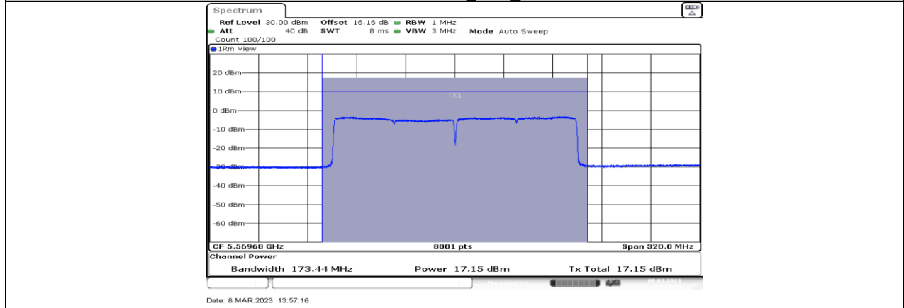
11AX160MIMO_Ant2_5570
