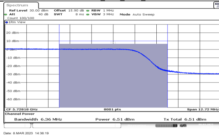
11BE20MIMO_Ant1_5720_UNII-3
