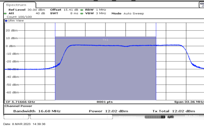
11BE20MIMO_Ant4_5720_UNII-2C
