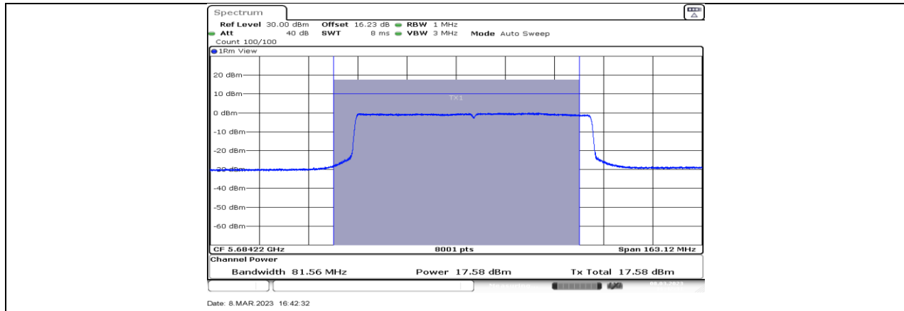
11BE80MIMO_Ant1_5690_UNII-2C
