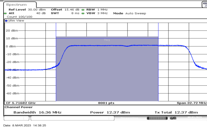
11BE20MIMO_Ant3_5720_UNII-2C
