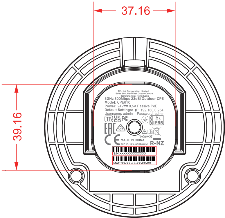
尺寸圖
