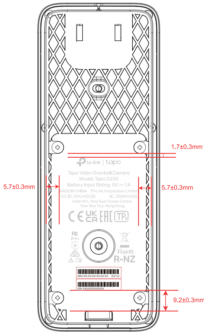
尺寸图
