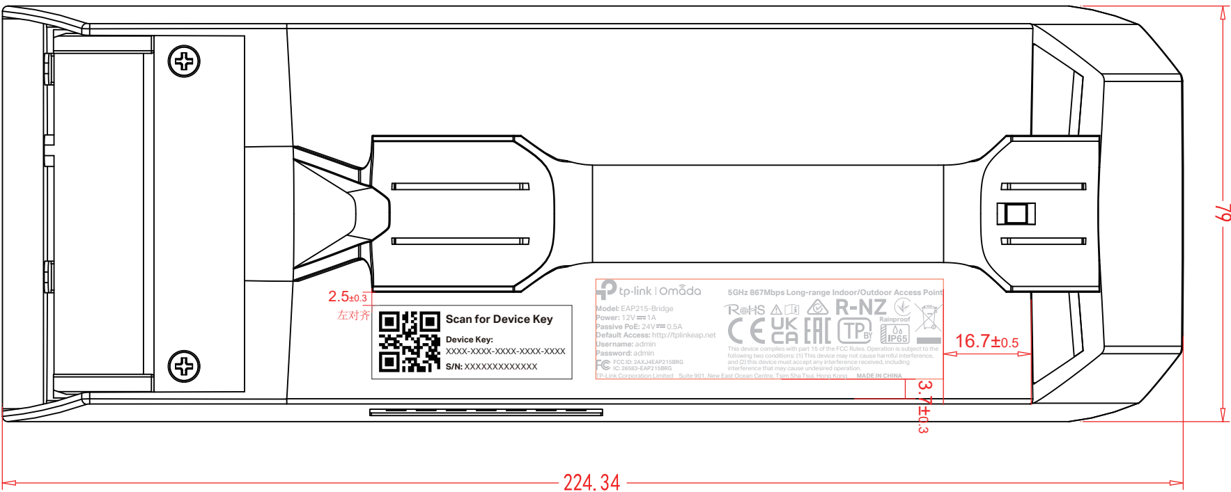
尺寸图
