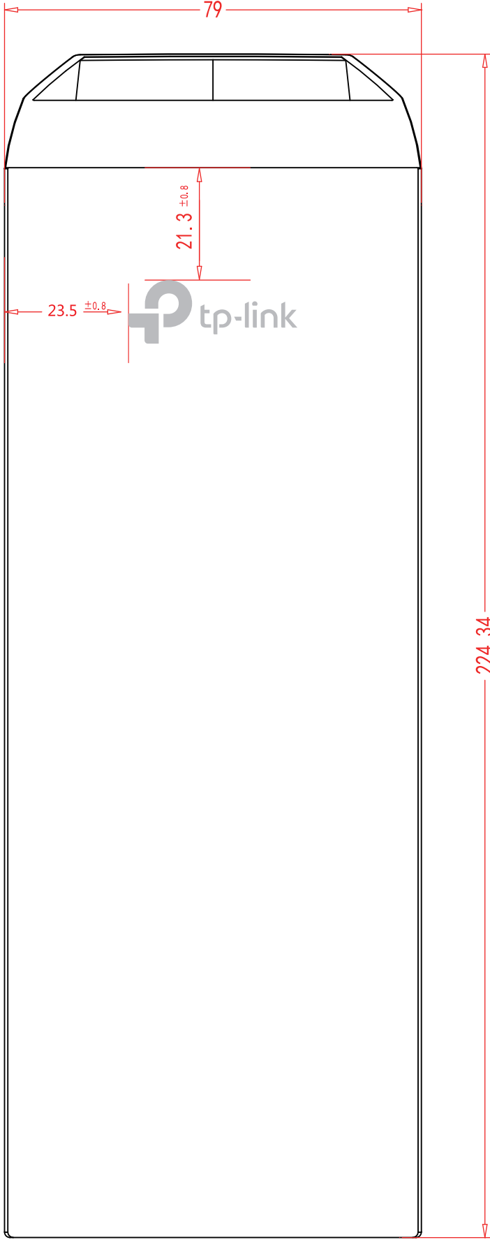
尺寸图
