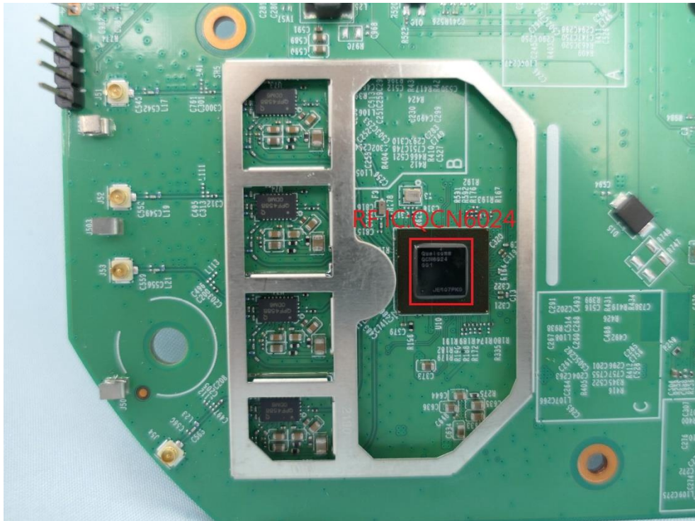
(17) EUT Photo
