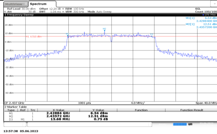
11G-CDD_Ant2_2437
