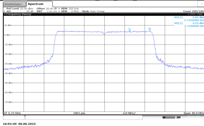
11AX20MIMO_Ant2_5720_UNII-3
