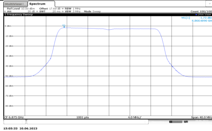
11AX20MIMO_Ant5_6875
