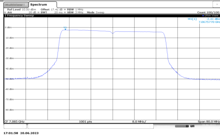
11AX40MIMO_Ant5_7085
