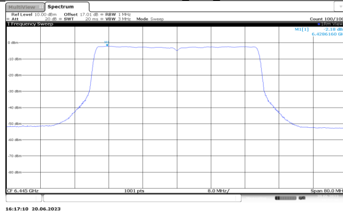
11AX40MIMO_Ant5_6445
