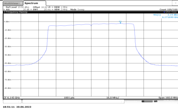
11AX80MIMO_Ant5_6145
