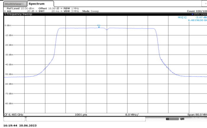
11AX40MIMO_Ant4_6485
