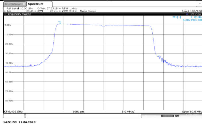
11BE40MIMO_Ant4_6405
