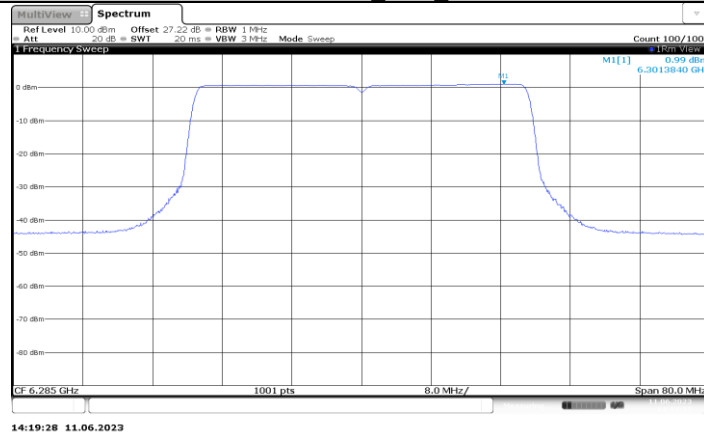
11BE40MIMO_Ant5_6285
