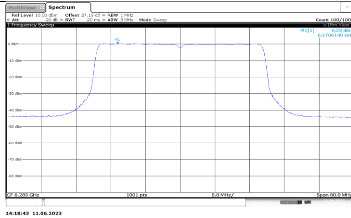
11BE40MIMO_Ant4_6285
