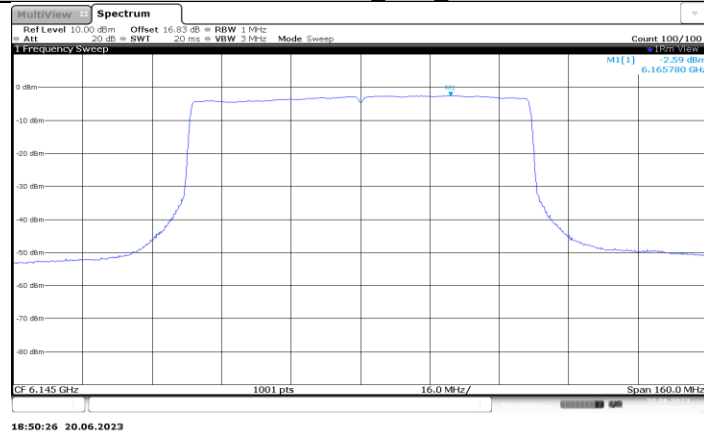
11AX80MIMO_Ant4_6145
