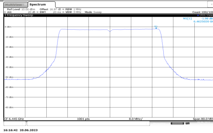
11AX40MIMO_Ant4_6445
