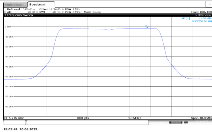
11AX20MIMO_Ant5_6715
