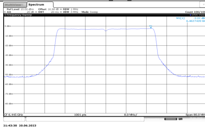
11BE40MIMO_Ant4_6445
