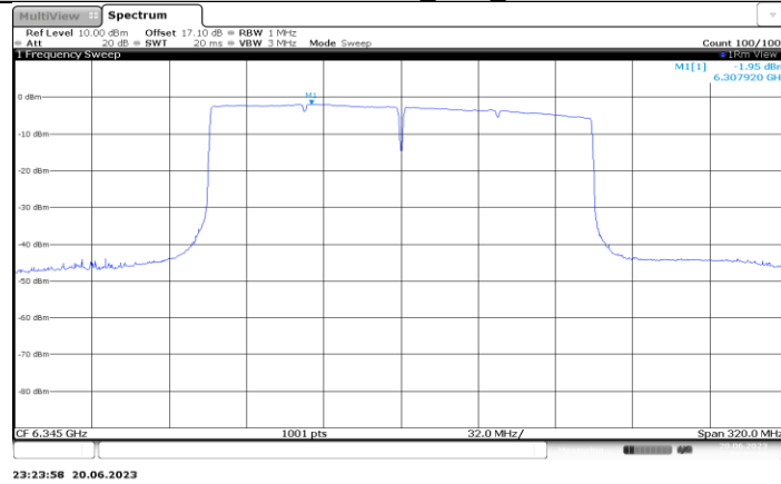
11BE160MIMO_Ant4_6345
