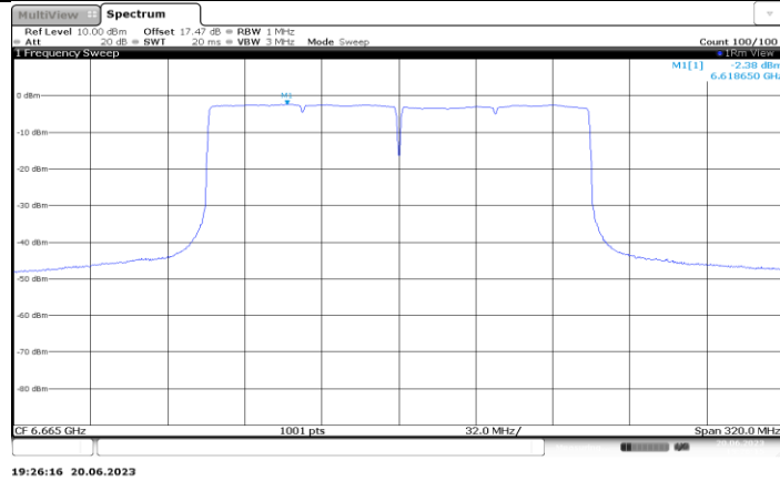
11AX160MIMO_Ant5_6665
