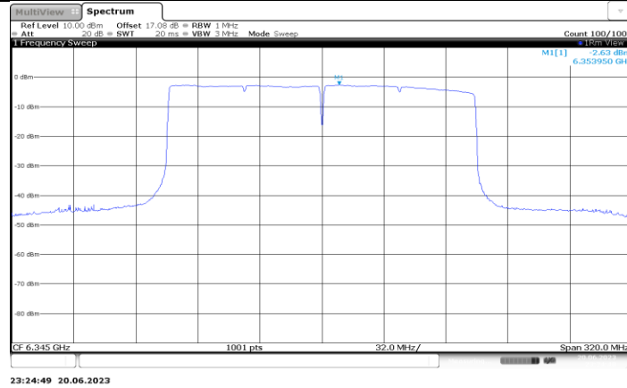
11BE160MIMO_Ant5_6345
