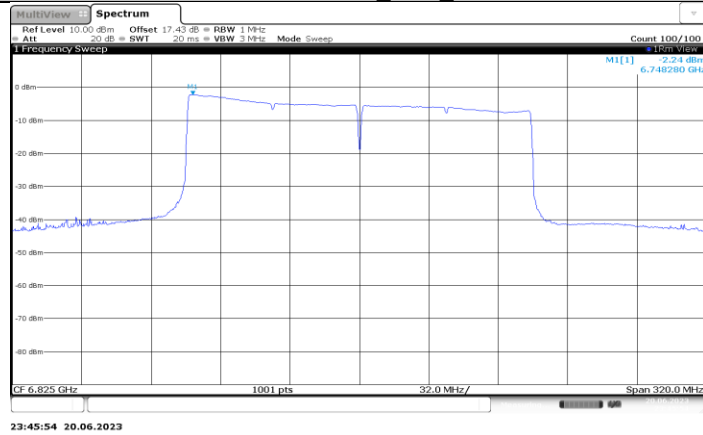
11BE160MIMO_Ant4_6825
