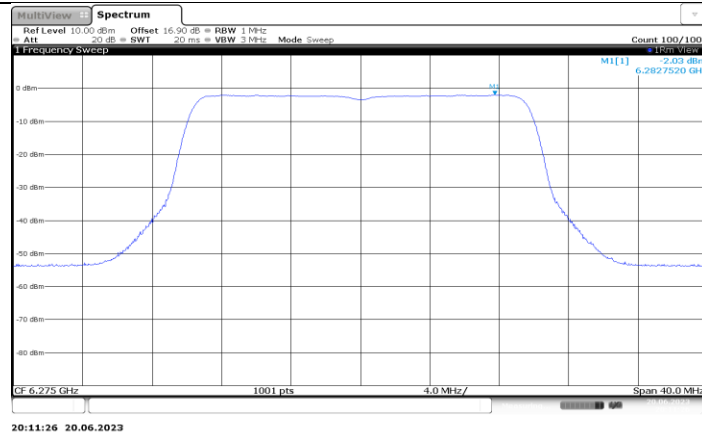
11BE20MIMO_Ant4_6275
