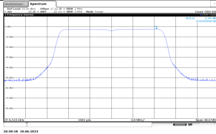
11BE20MIMO_Ant4_6515
