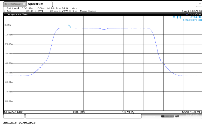
11BE20MIMO_Ant5_6275
