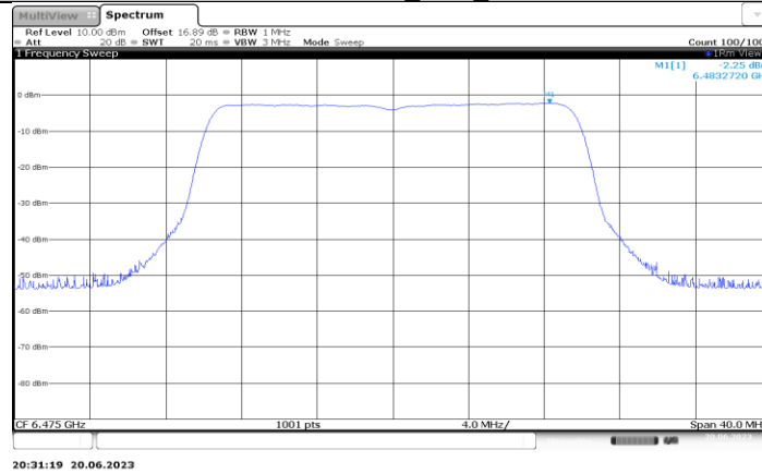
11BE20MIMO_Ant5_6475
