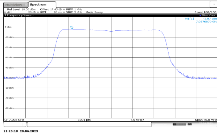
11BE20MIMO_Ant5_7095
