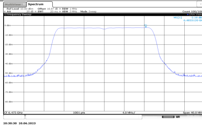
11BE20MIMO_Ant4_6475
