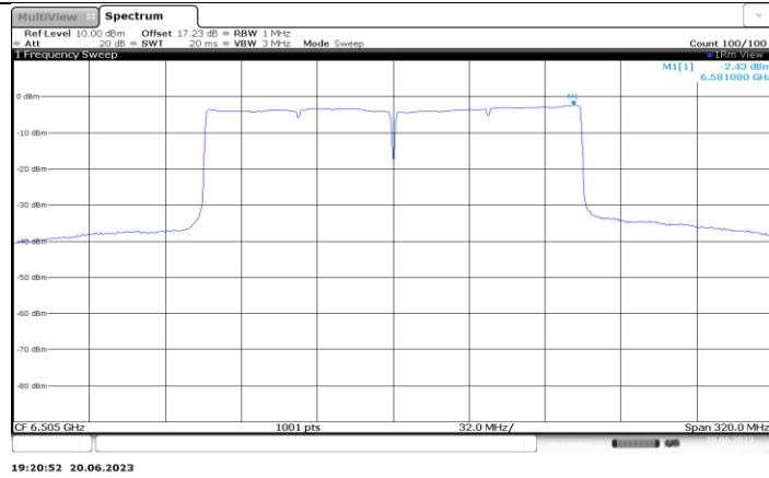
11AX160MIMO_Ant5_6505
