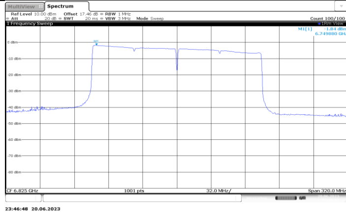
11BE160MIMO_Ant5_6825
