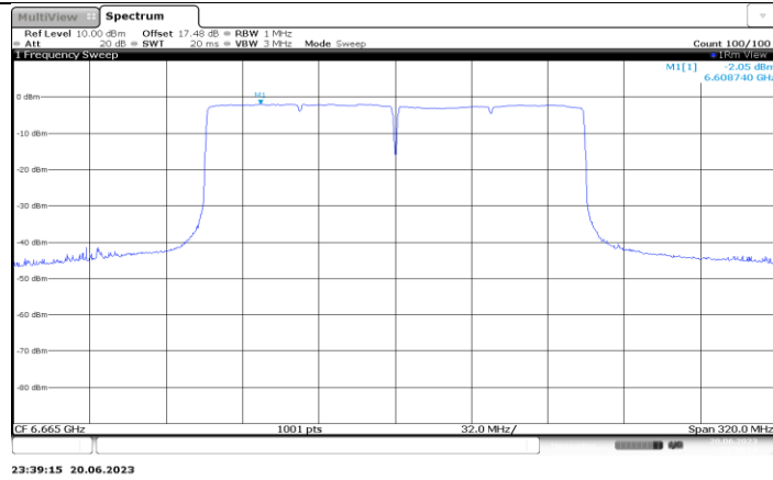
11BE160MIMO_Ant5_6665
