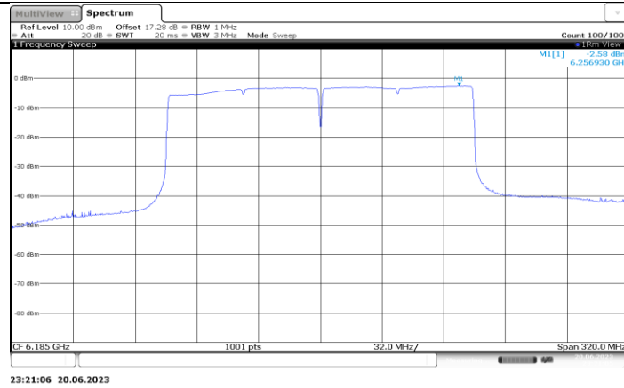
11BE160MIMO_Ant5_6185
