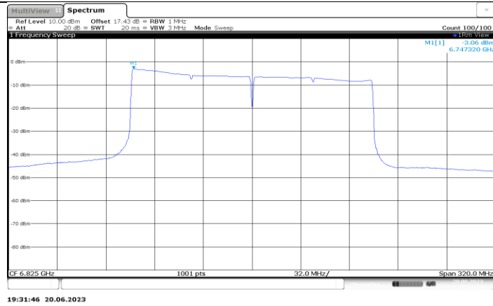
11AX160MIMO_Ant4_6825
