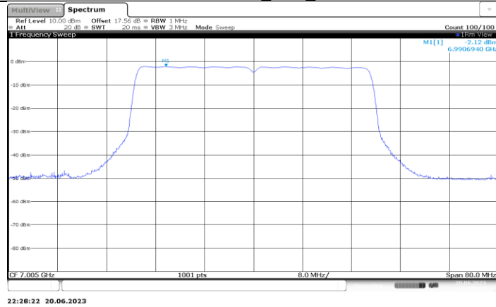
11BE40MIMO_Ant4_7005
