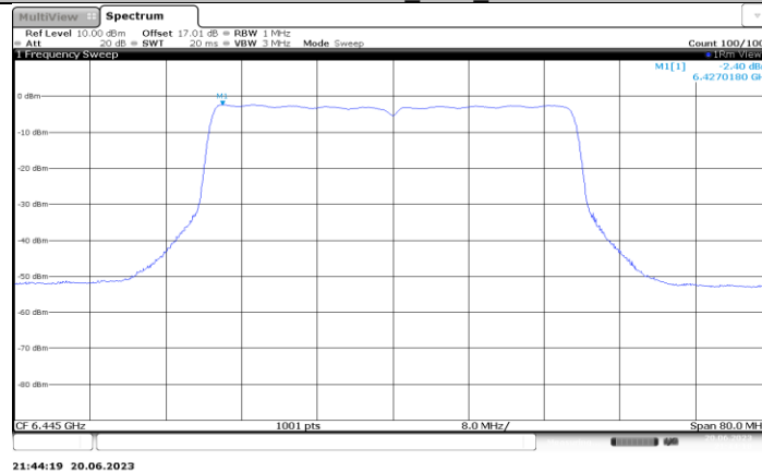
11BE40MIMO_Ant5_6445
