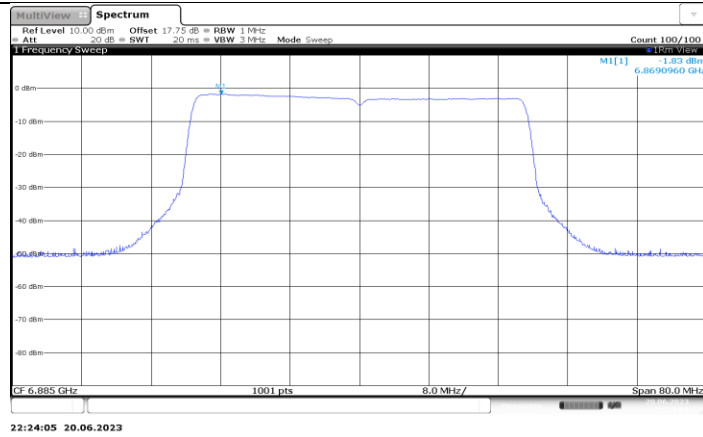
11BE40MIMO_Ant5_6885
