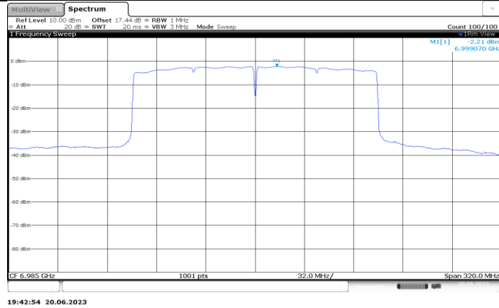
11AX160MIMO_Ant4_6985
