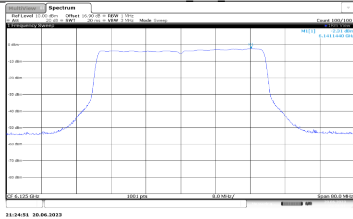
11BE40MIMO_Ant4_6125
