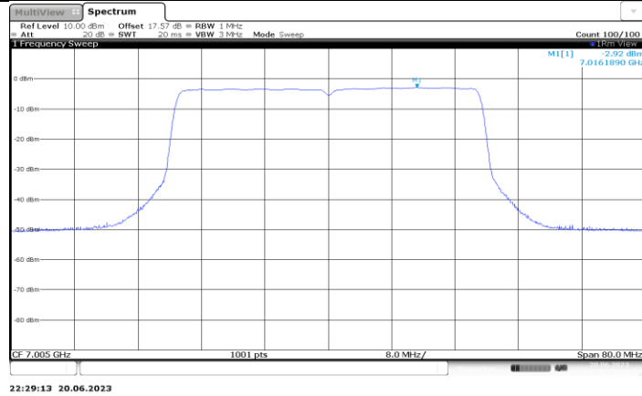
11BE40MIMO_Ant5_7005
