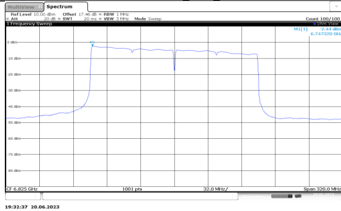
11AX160MIMO_Ant5_6825
