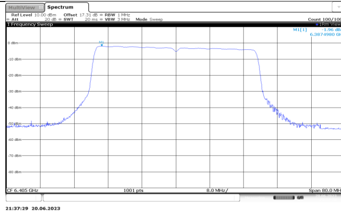
11BE40MIMO_Ant5_6405
